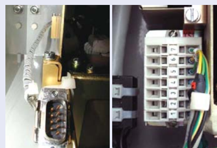
Коммуникационные интерфейсы (RS232 слева, RS485 справа)
