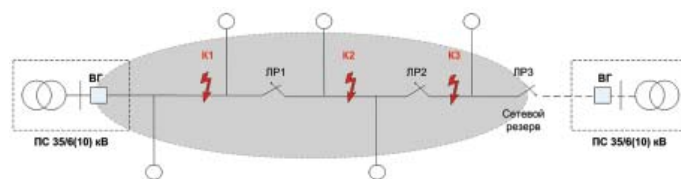
Базовый вариант схемы ВЛ 6-10 кВ
