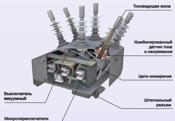
в) внутренне устройство Коммутационный модуль
