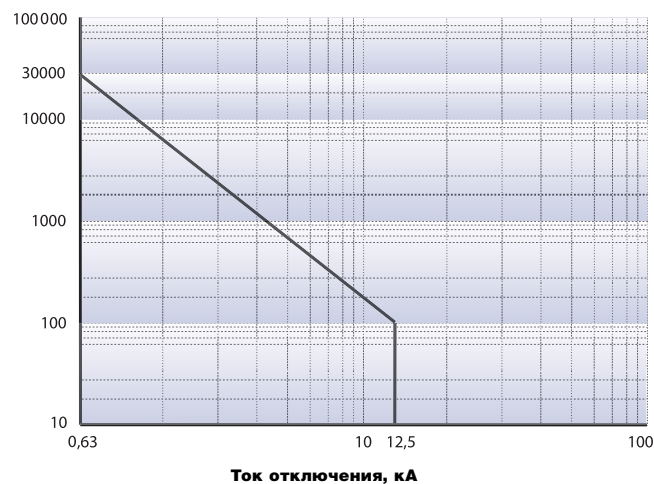
Диаграмма коммутационного ресурса РВА/TEL
