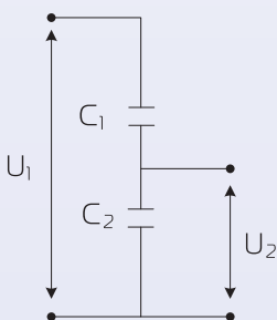
Емкостной делитель напряжения
