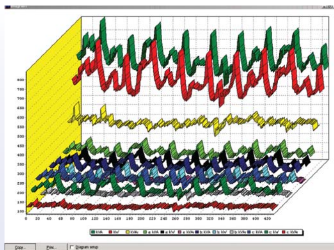
Графическое отображение журнала изменения нагрузок TELUS
