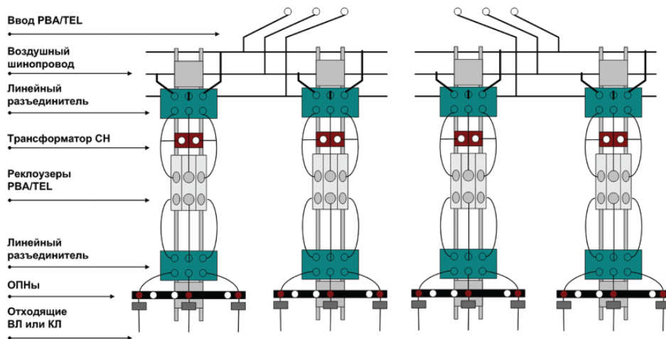
Открытое распределительное устройство с применением РВА/TEL
