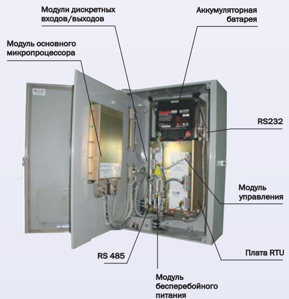
б) внутренние модули
