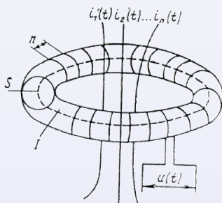
Катушка Роговского
