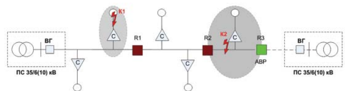
П – плавкие предохранители
