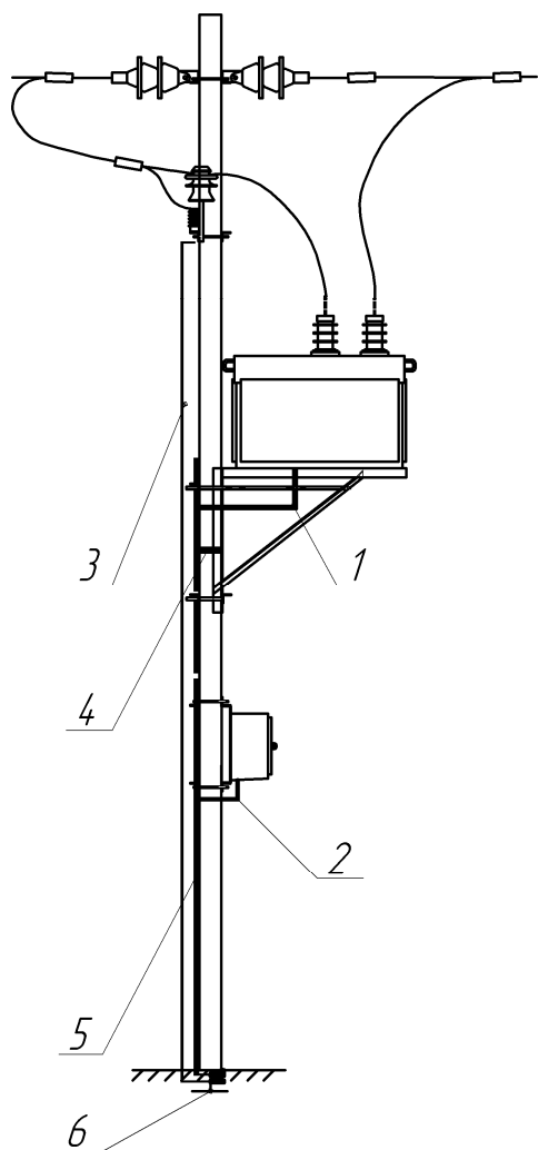
Рис.2. Схема заземления КСО/ПКУ при расположении на 1-й опоре
