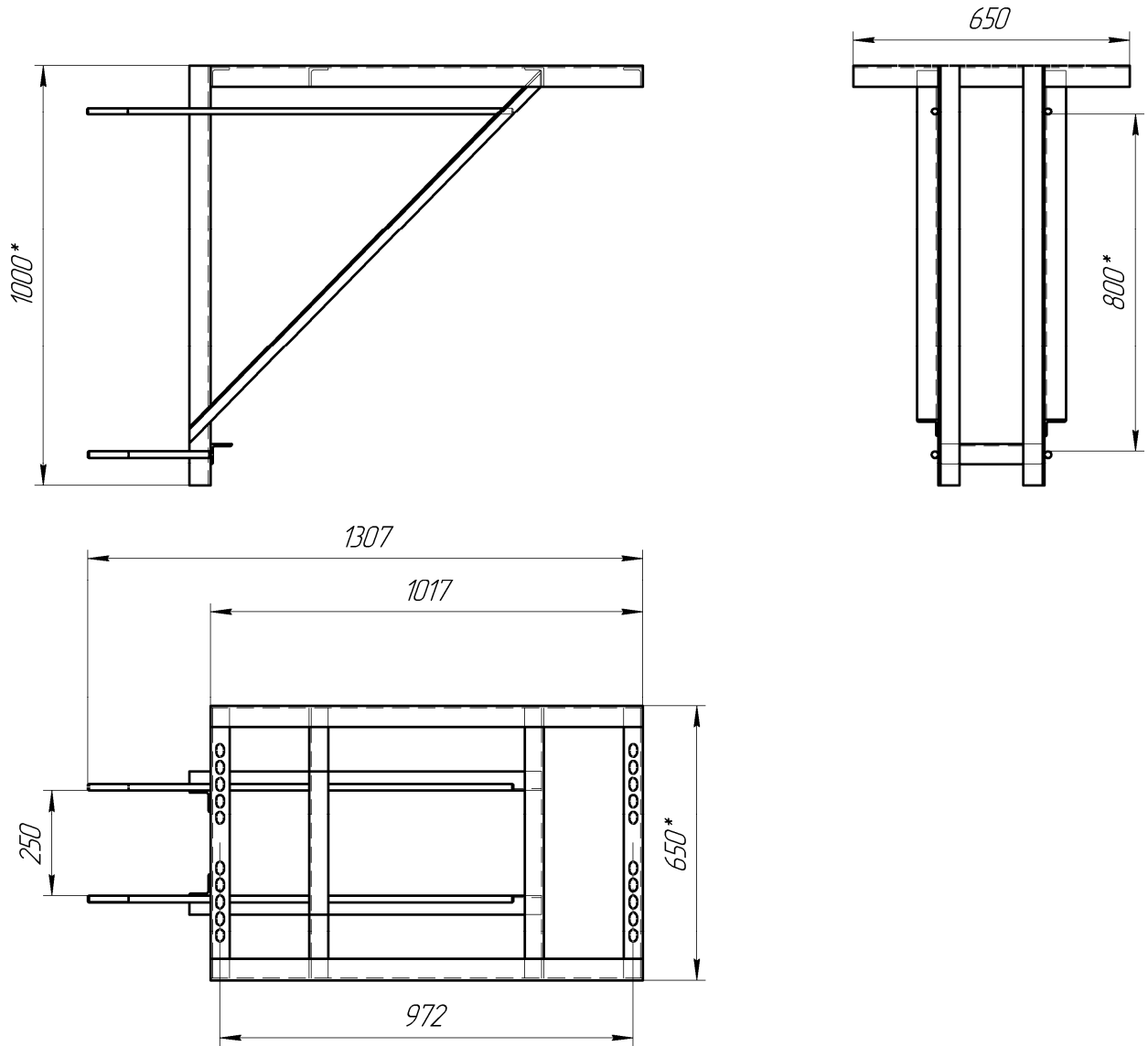
Монтажный комплект для установки на одну опору
