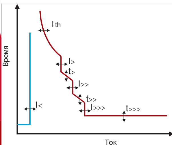
Характеристики отключения
