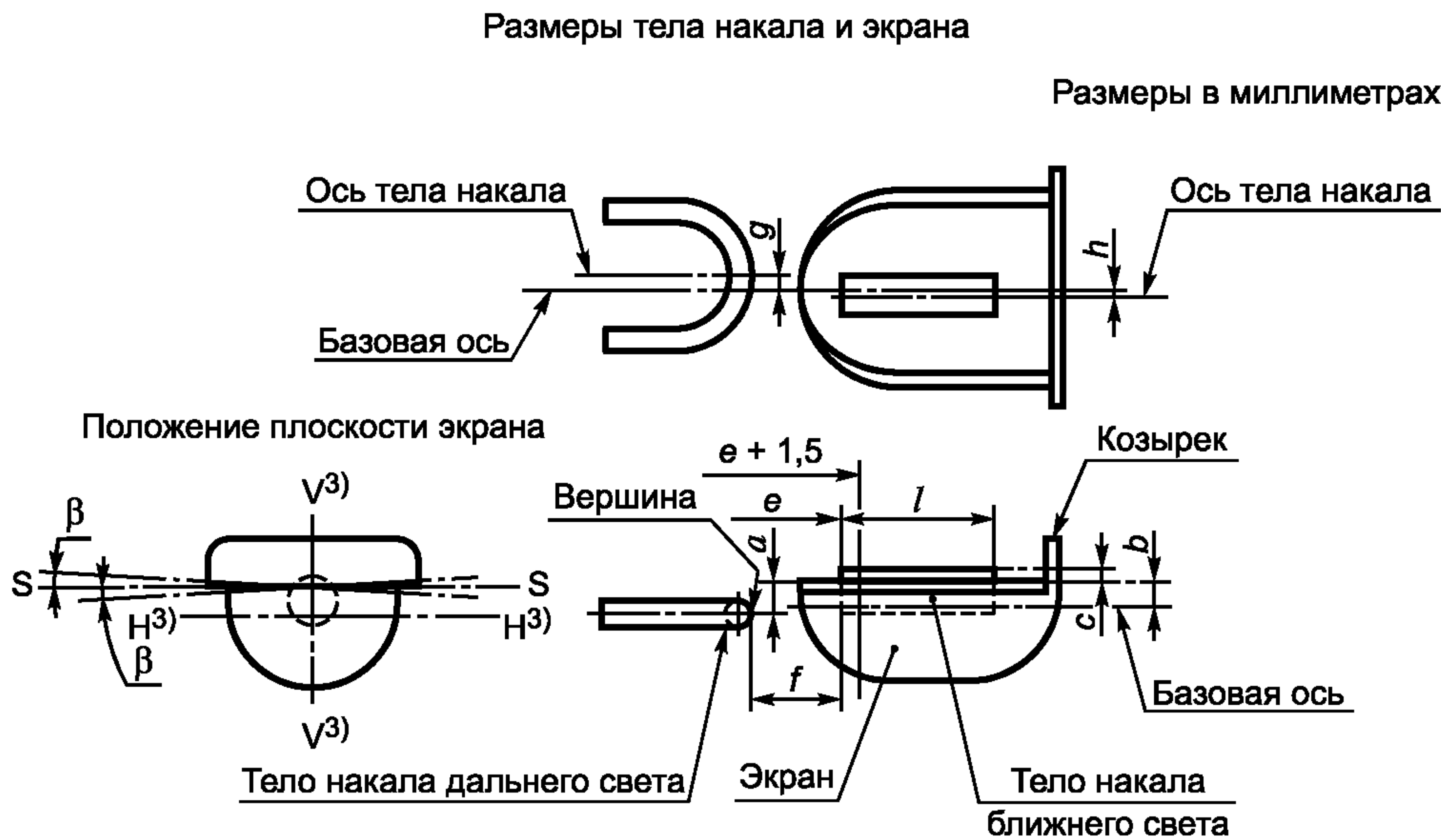
Параметры и размеры лампы накаливания
