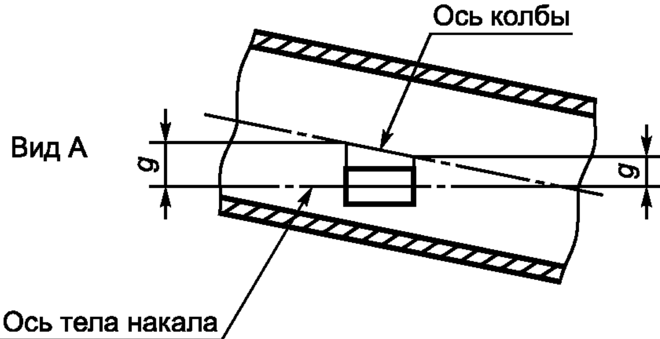
Рисунок 6 — Эксцентриситет колбы 8)
