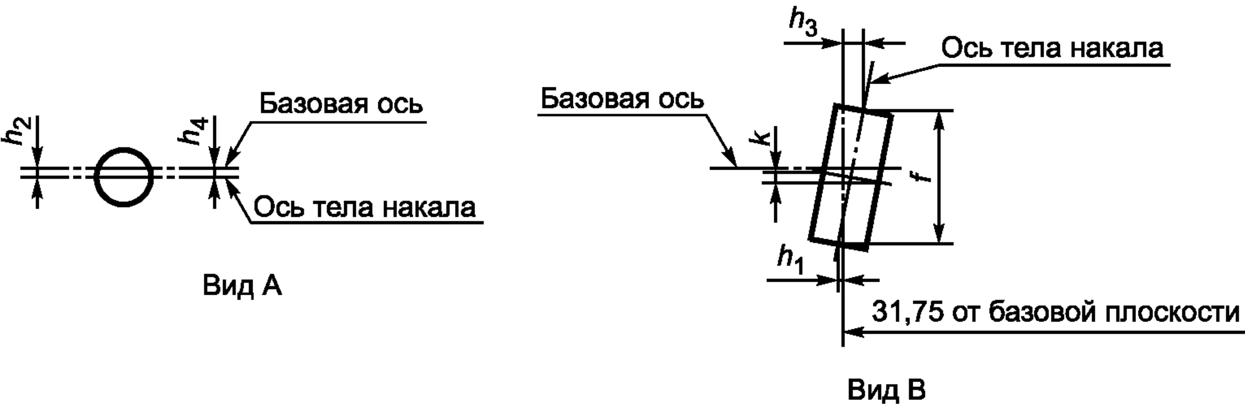
Размеры и положение тела накала
