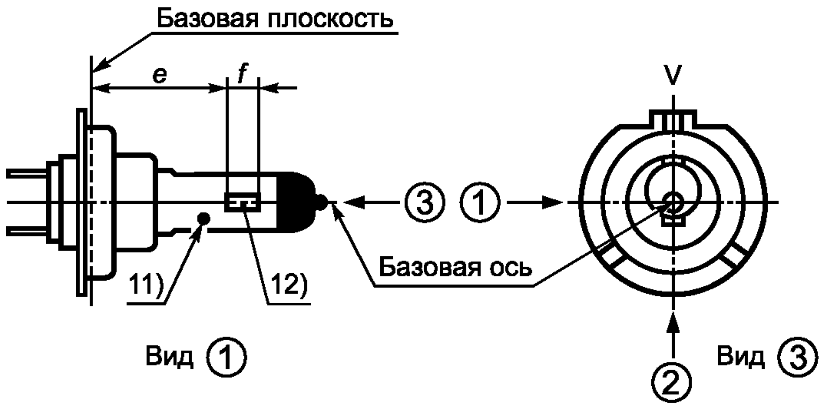
Рисунок 1 — Изображение лампы
