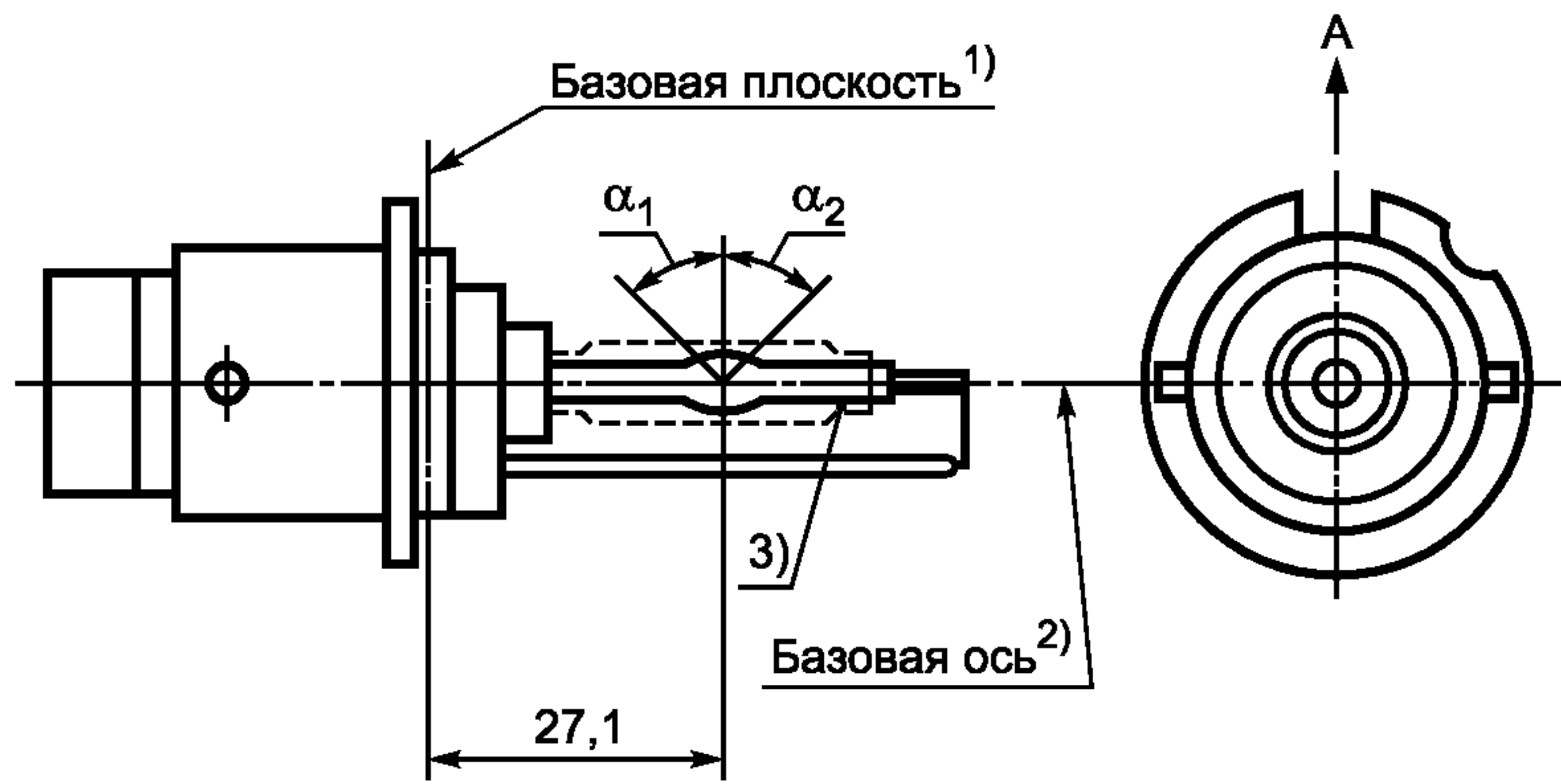
Рисунок 2 — Категория D2S, тип с соединителем, цоколь P32d-2
