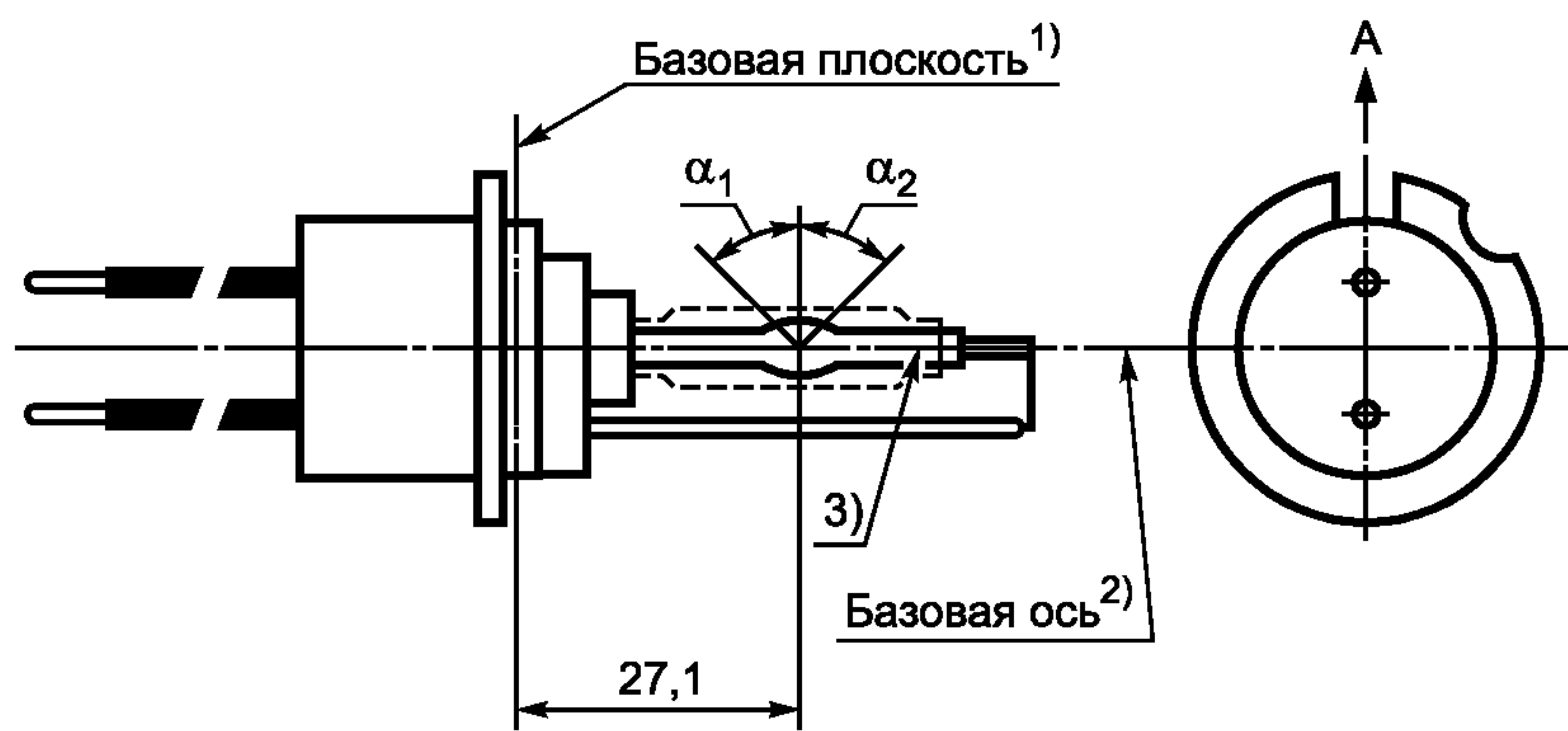
Рисунок 1 — Категория D1S, тип с кабелями, цоколь PK32d-2
