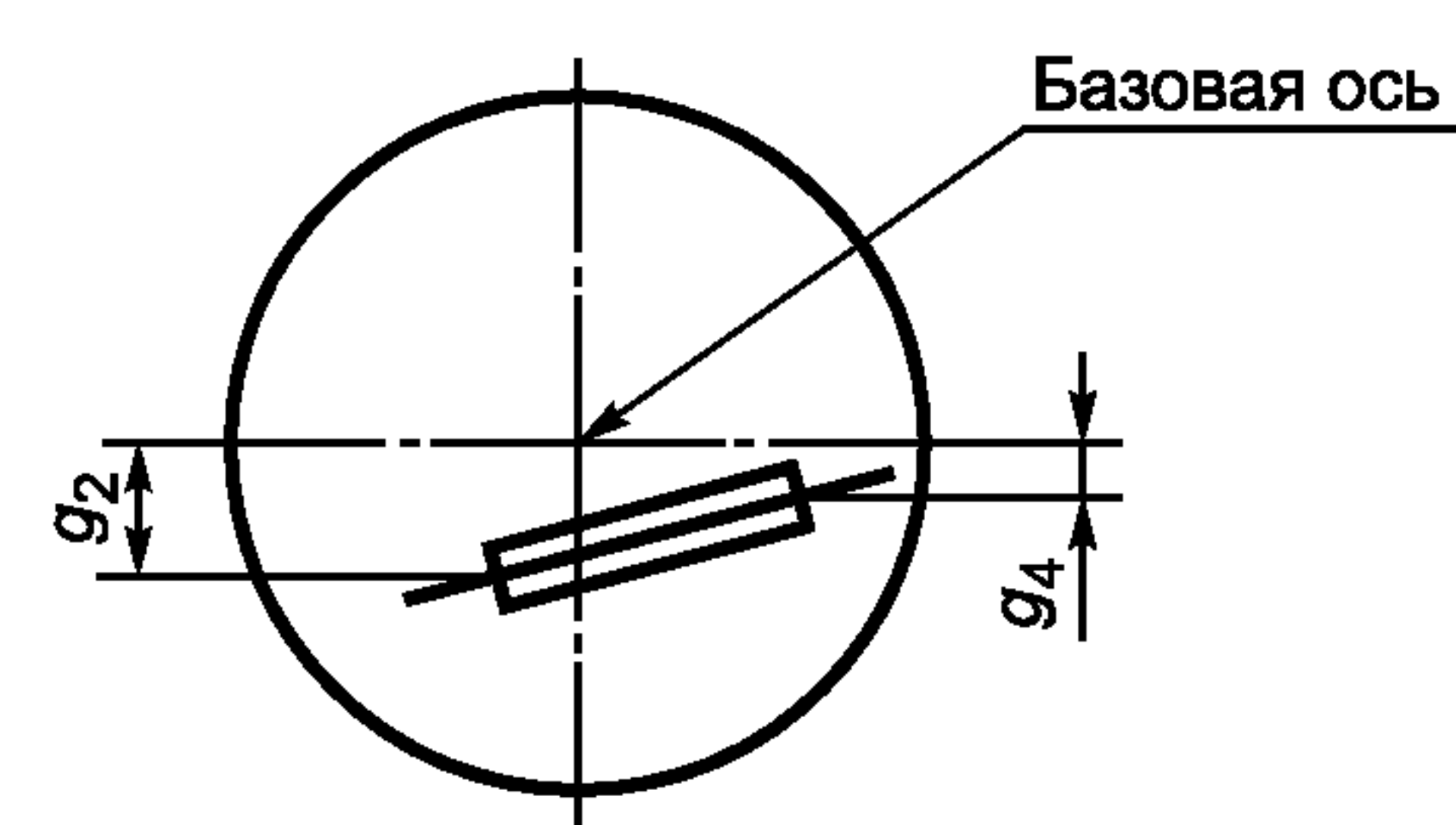
Рисунок 3 — Положение и размеры тела накала
