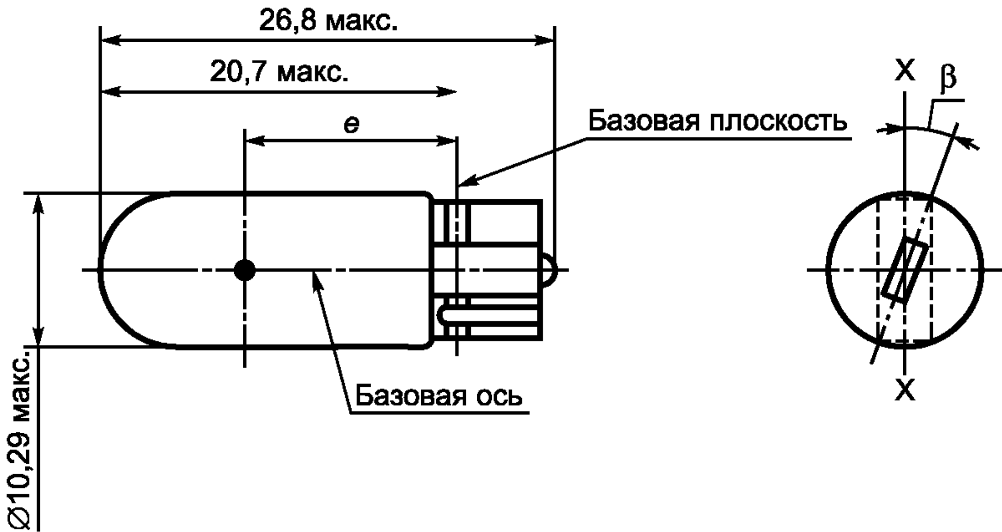
Параметры и размеры лампы накаливания
