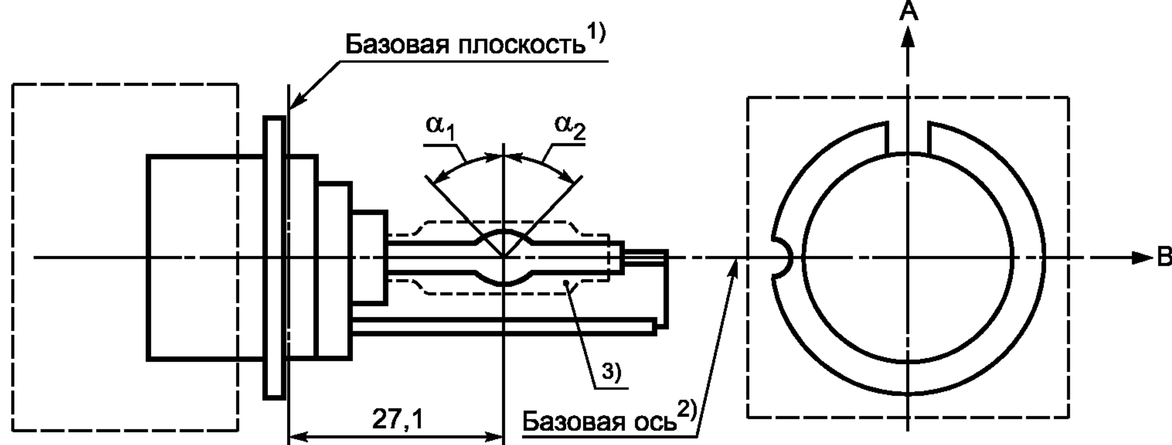
Рисунок 3 — Категория D3S, тип со стартером, цоколь PK32d-5
