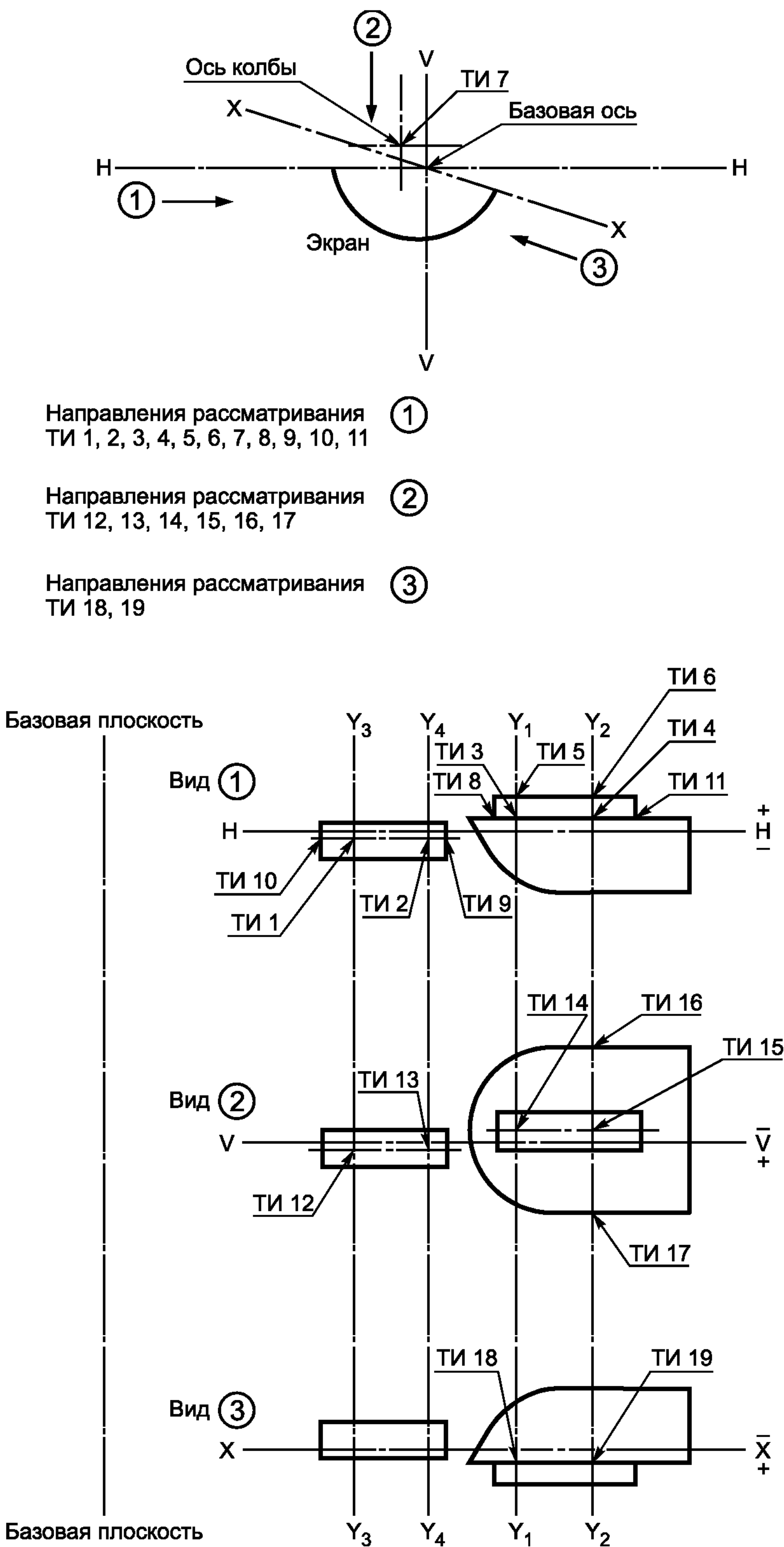
Рисунок Е.2 — Положение измерительных точек ламп H4 и HS1
