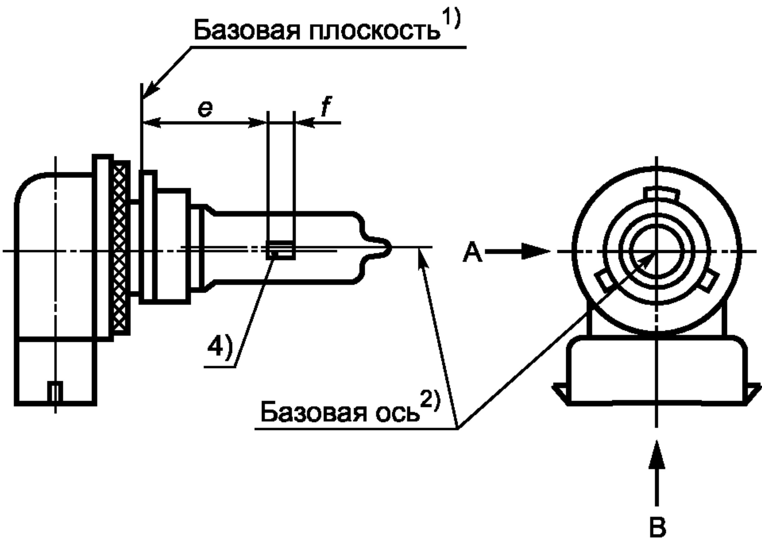
Рисунок 1 — Изображение лампы
