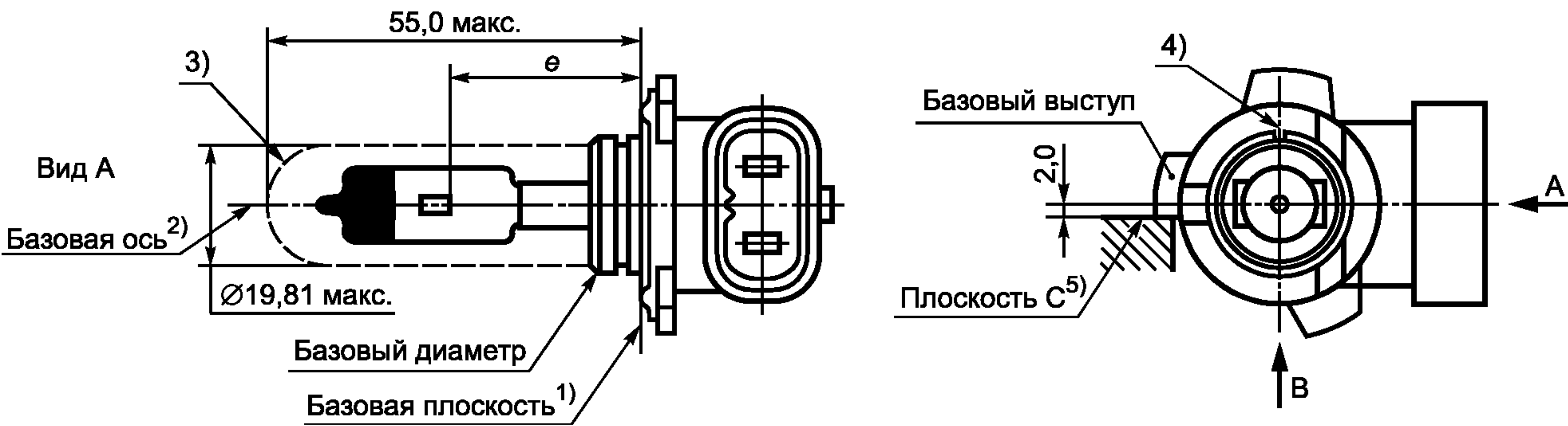
Рисунок 1 — Изображение лампы
