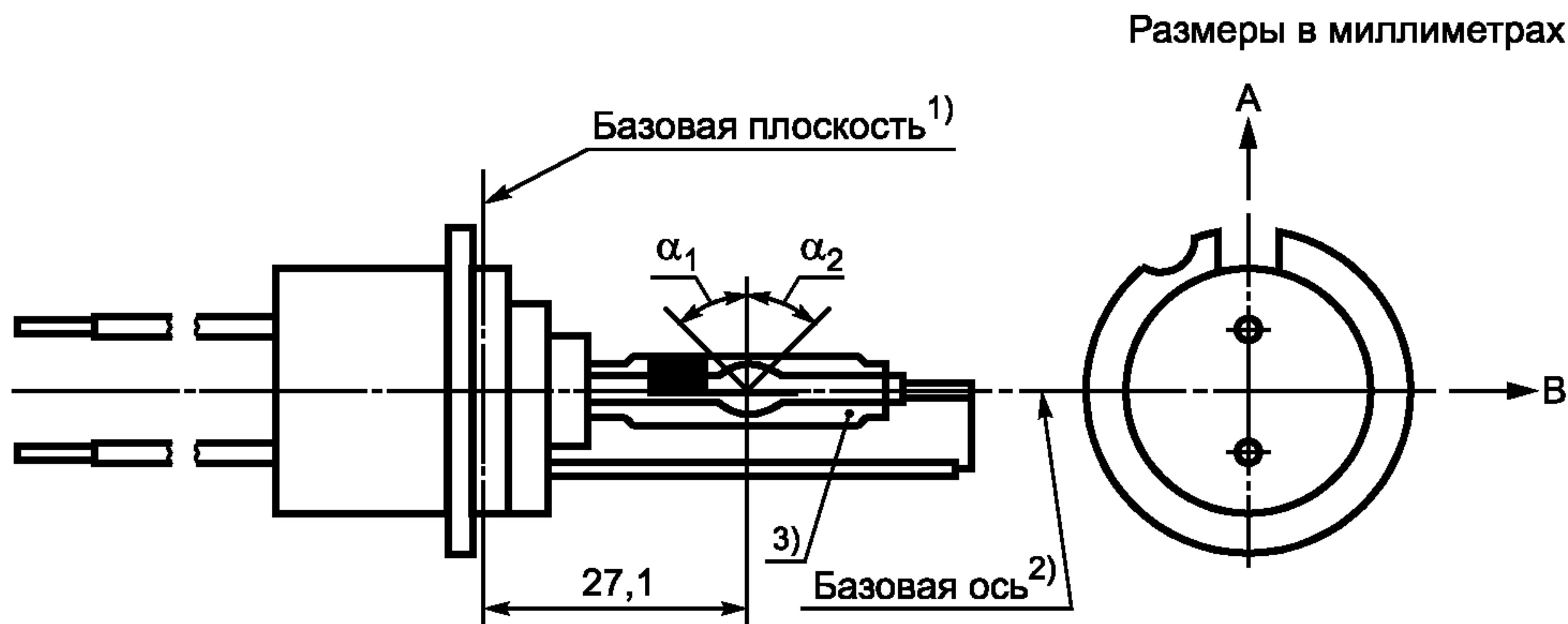
Рисунок 1 — Категория D1R, тип с кабелями, цоколь PK32d
