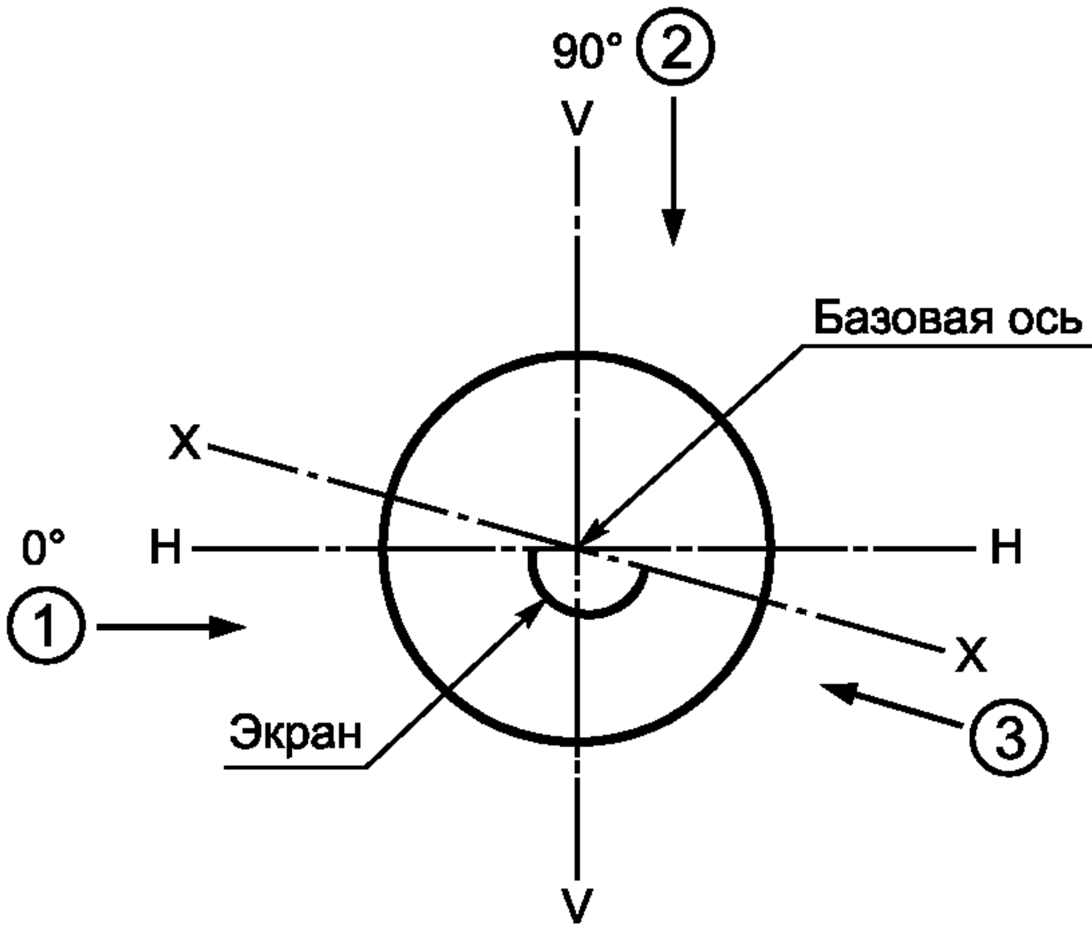
Рисунок Е.1 — Направления видов, рассматривают сверху лампы
