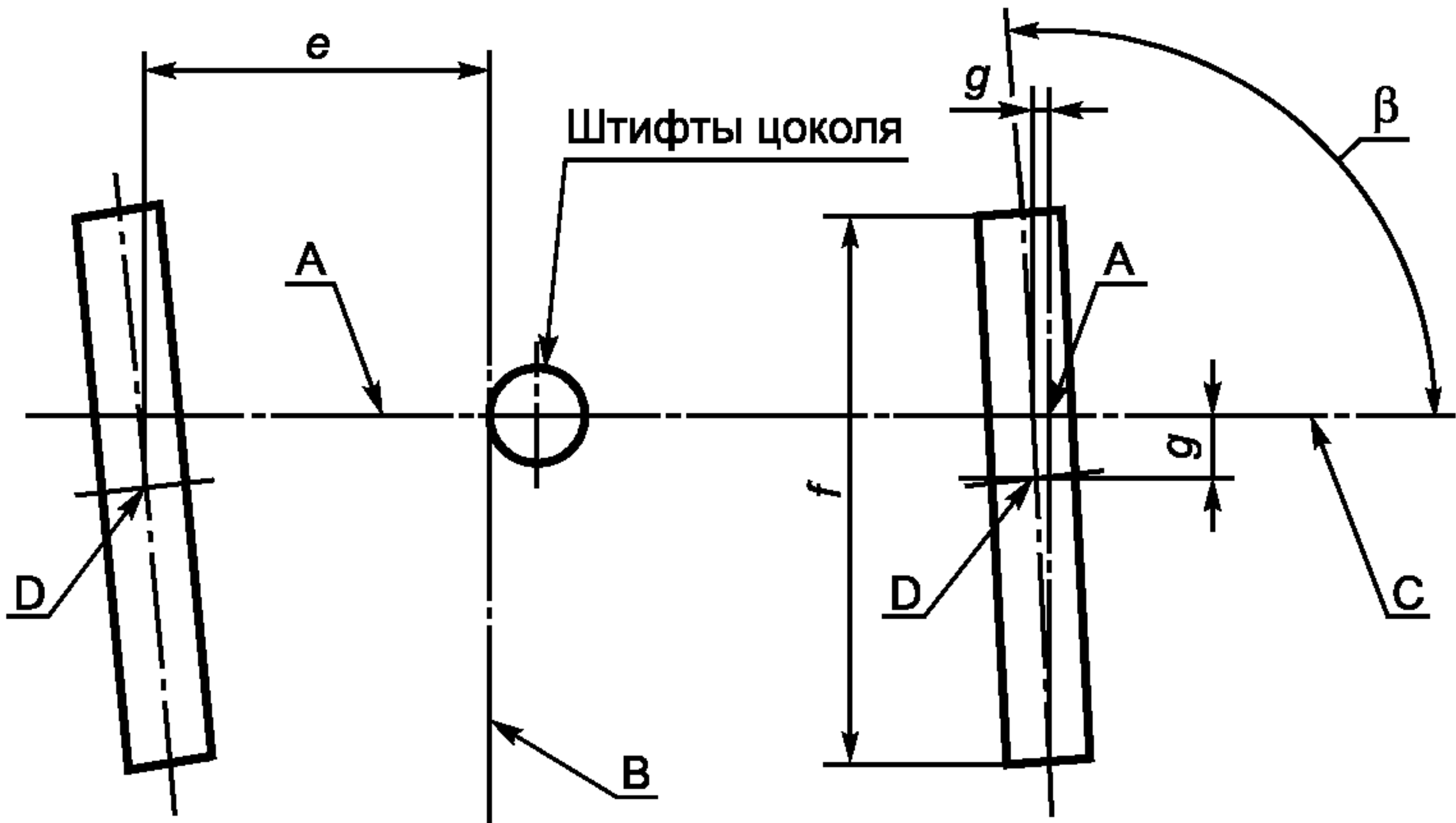
Вид лампы спереди
