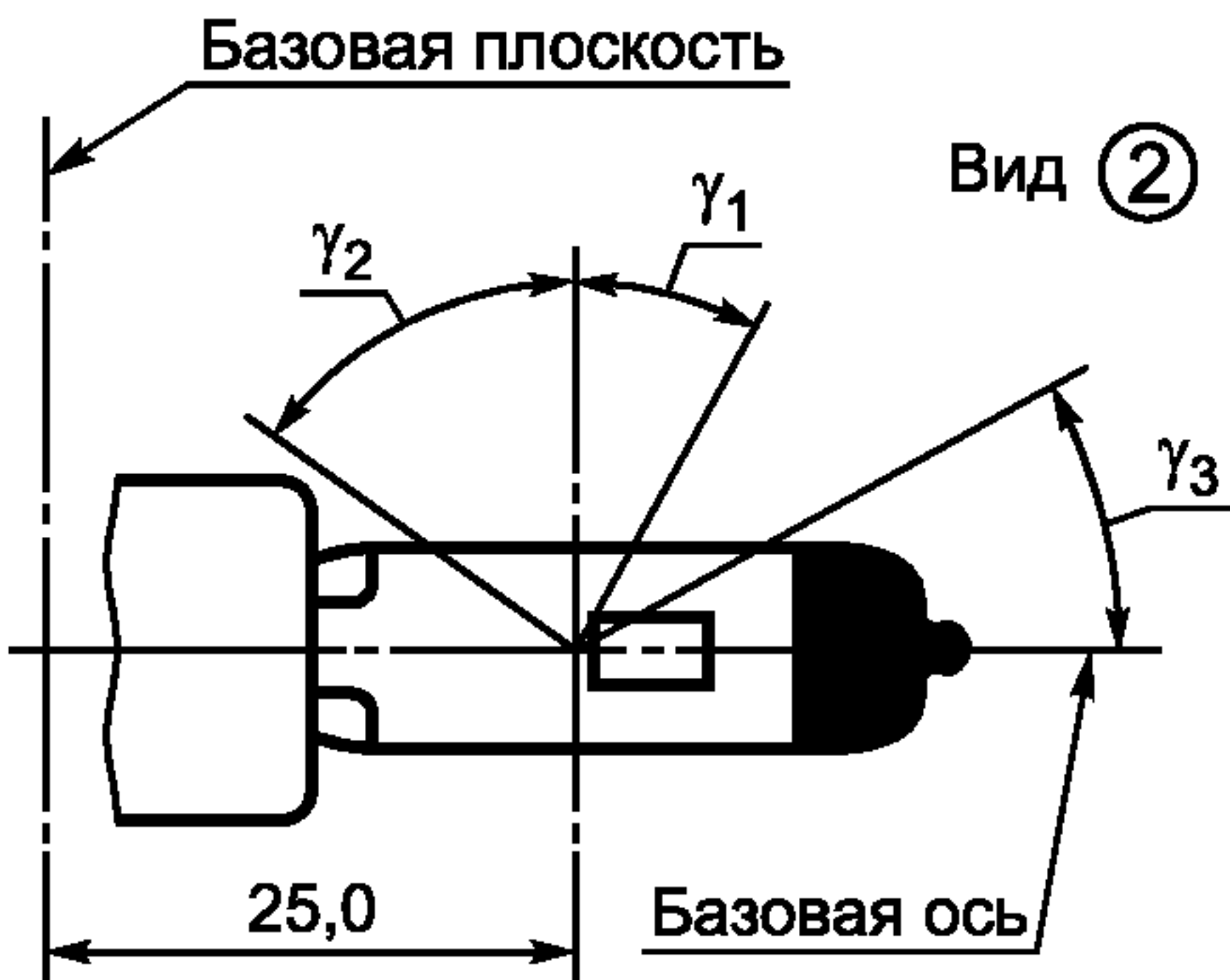
Рисунок 4 — Неискаженные зоны и черный купол
