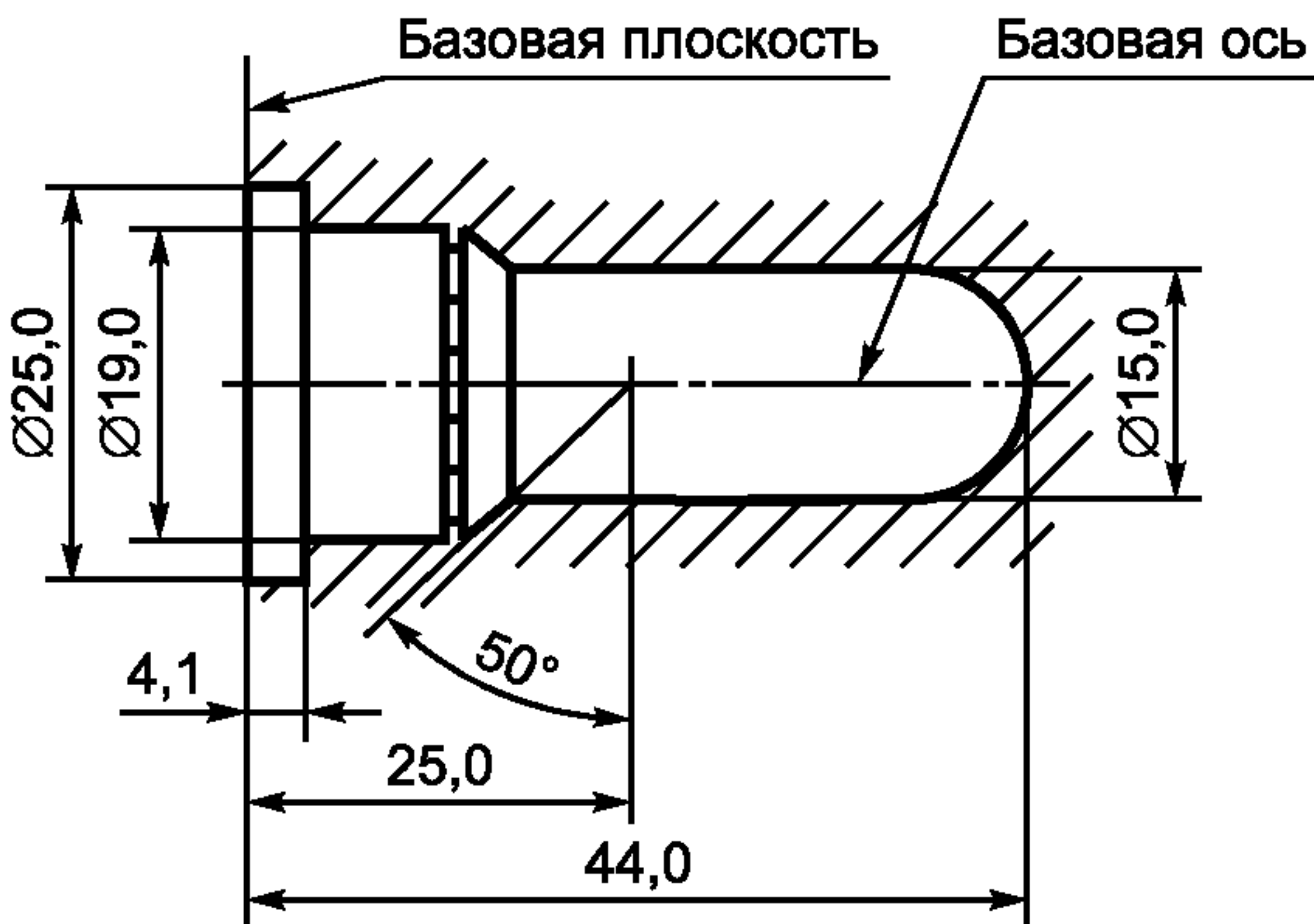
Рисунок 2 — Наибольший контур лампы 3)
