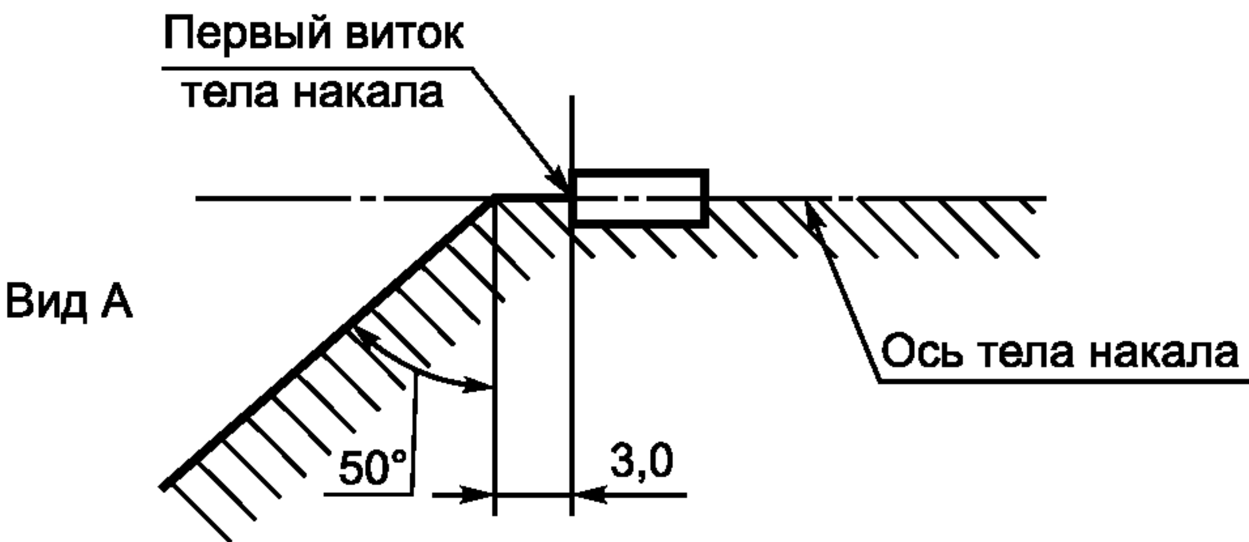
Рисунок 4 — Зона без металлических деталей 6)
