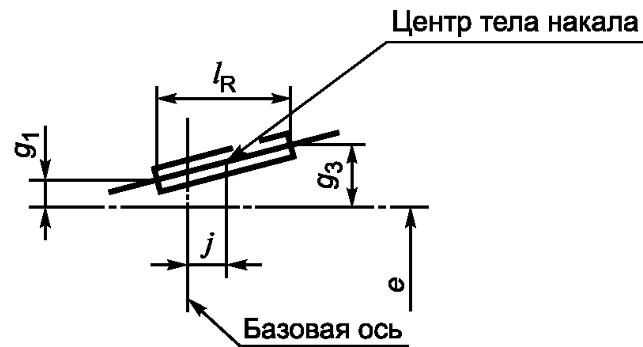
Вид В тела накала дальнего света
