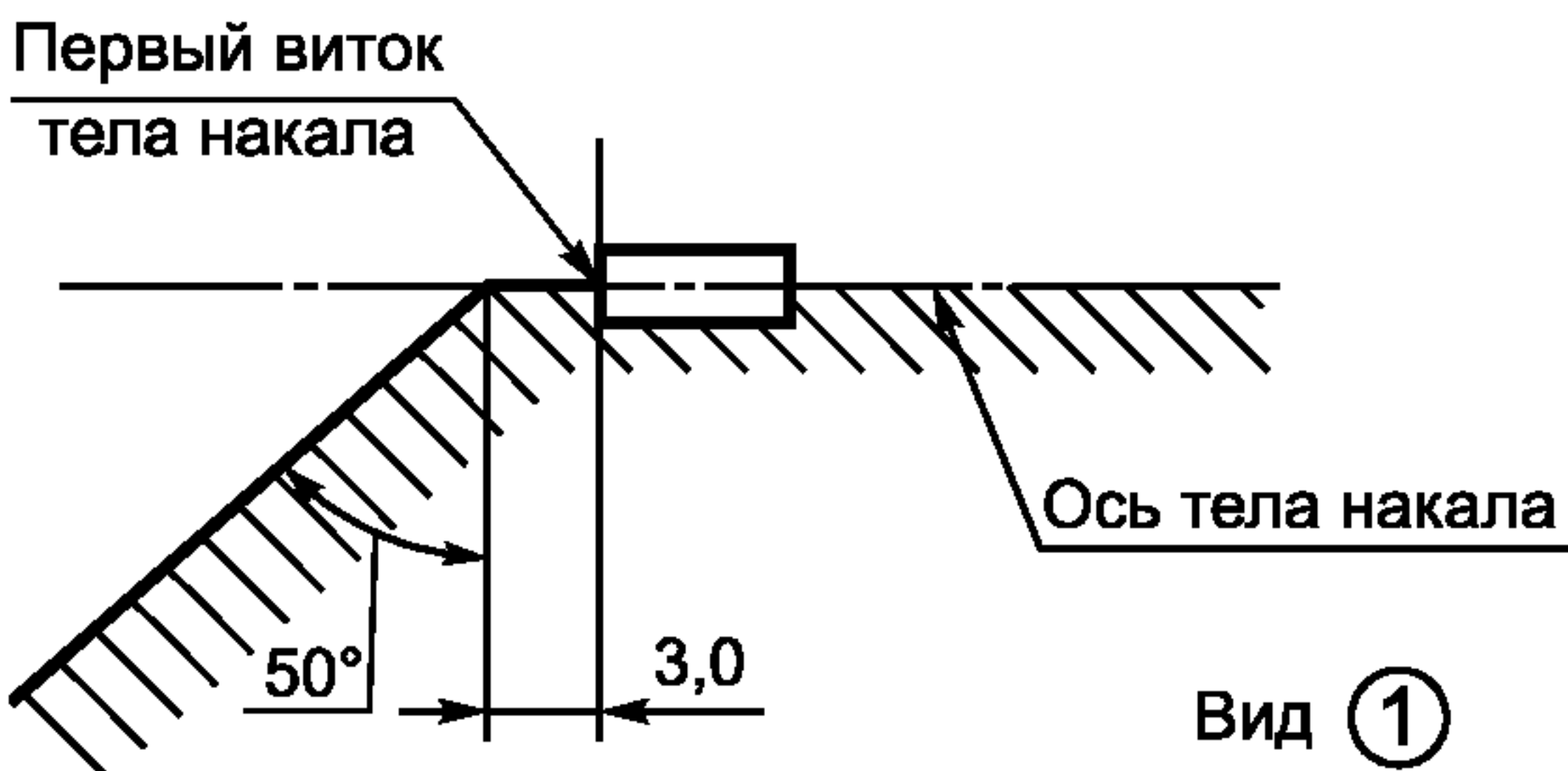
Рисунок 5 — Зона отсутствия металлических частей
