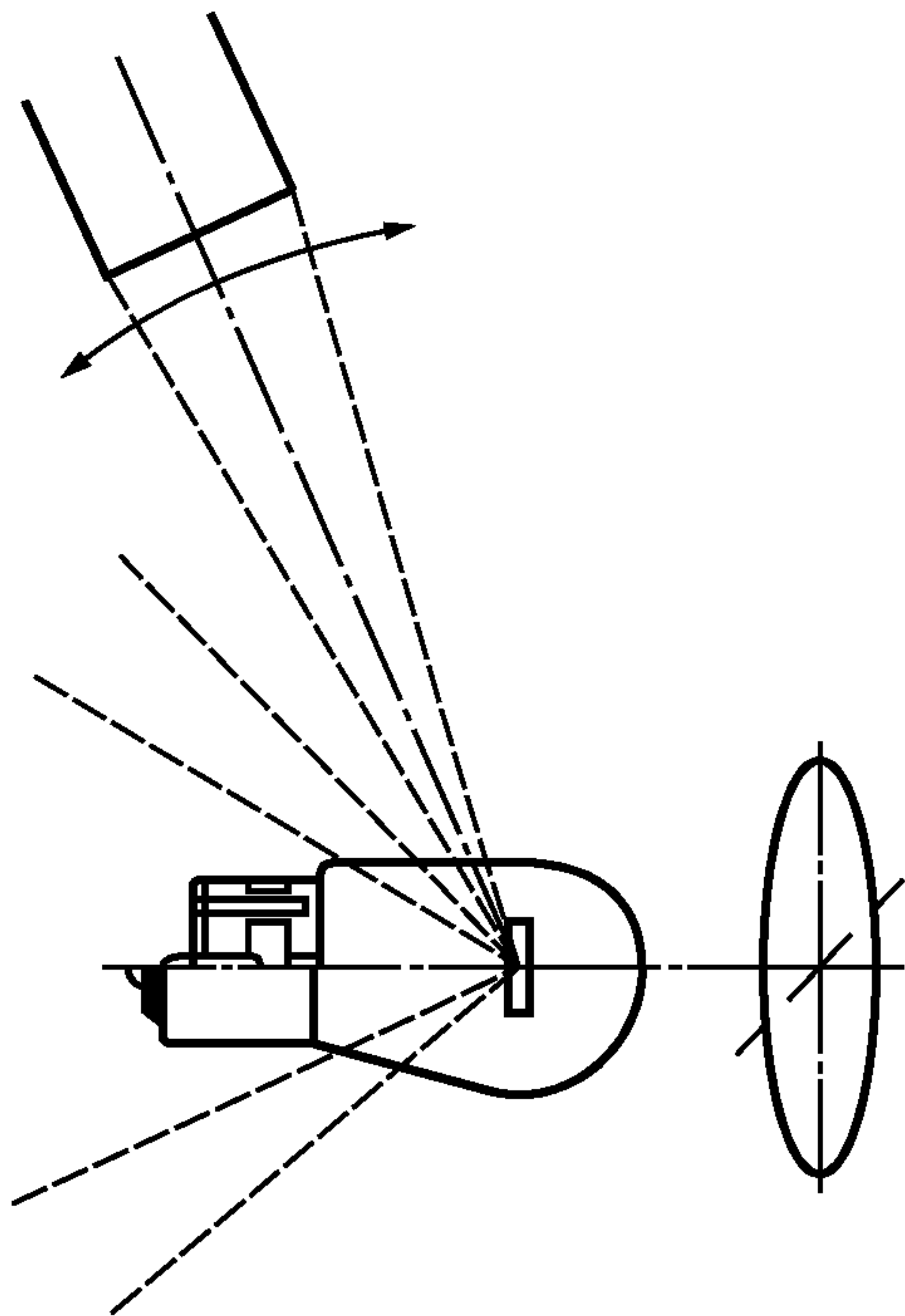
Рисунок В.2 — Положения колориметрической головки при измерении ламп для светосигнальных приборов
