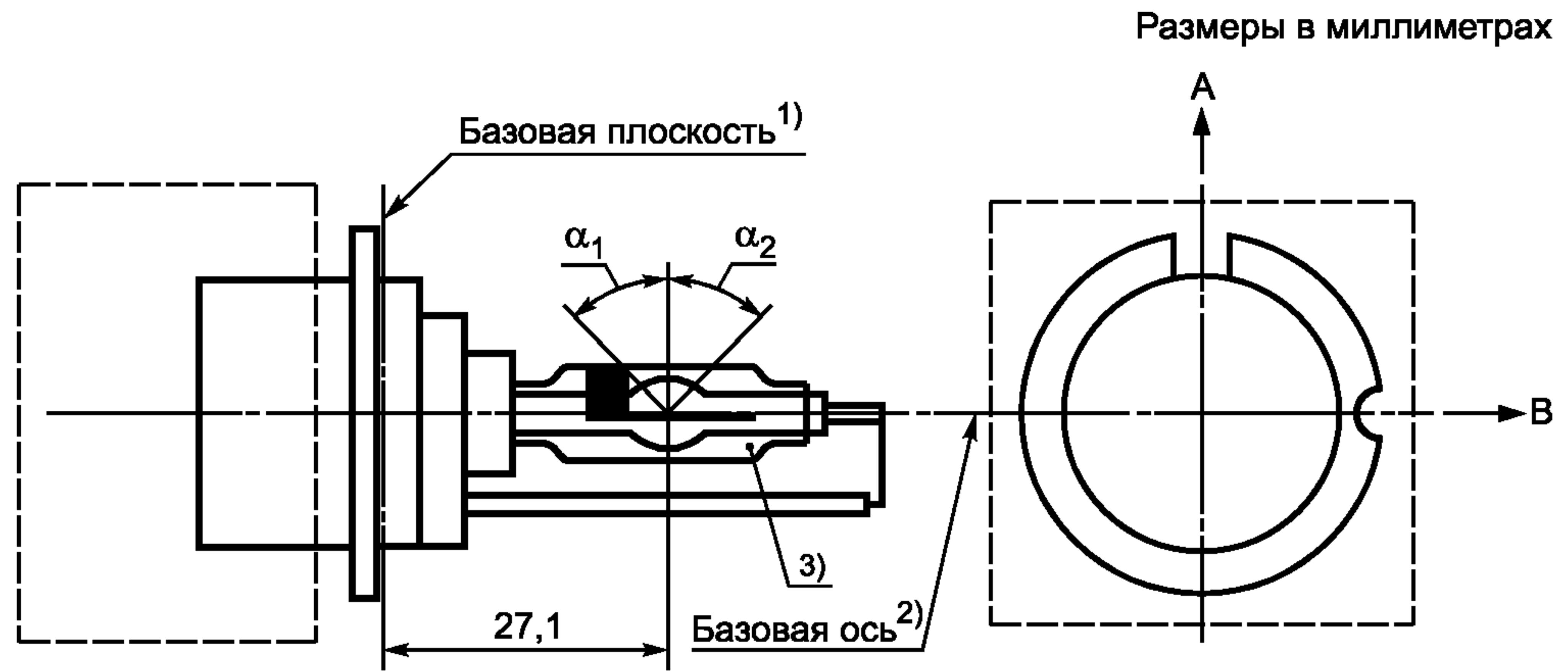
Рисунок 3 — Категория D3R, тип со стартером, цоколь PK32d-6
