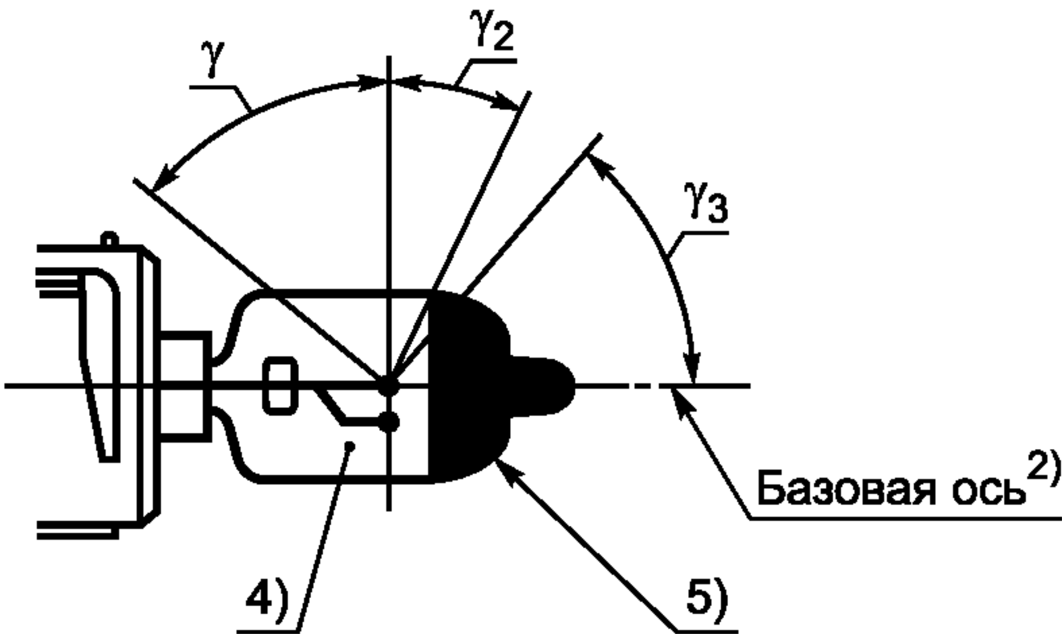
Рисунок 2 — Зона без искажений и черный купол
