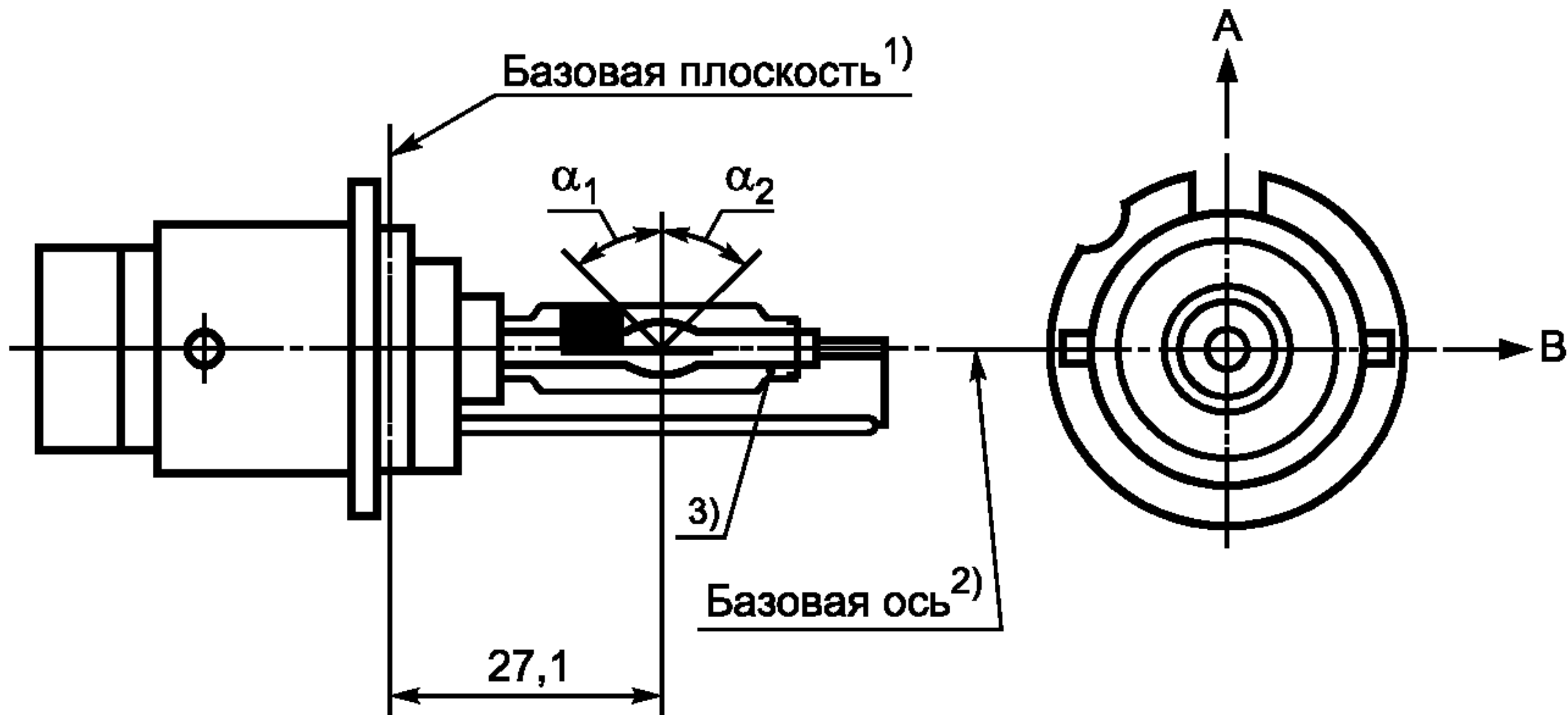
Рисунок 2 — Категория D2R, тип с соединителем, цоколь P32d
