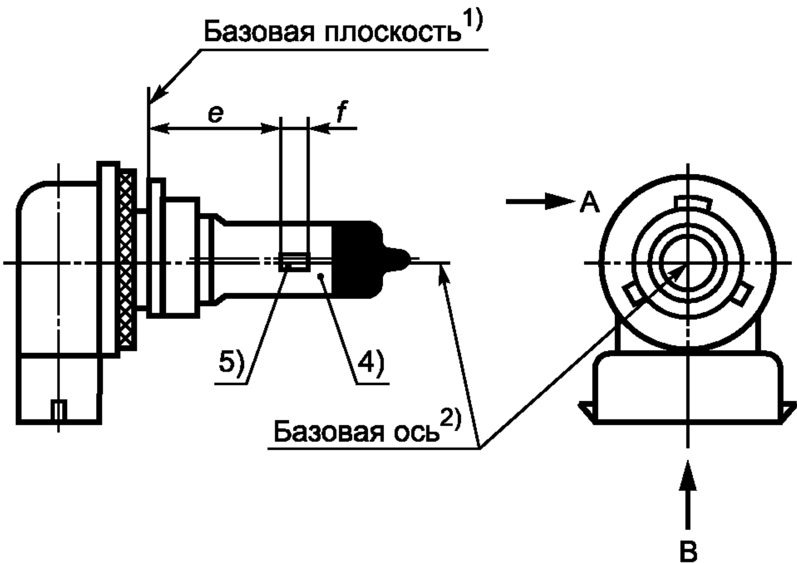
Рисунок 1— Изображение лампы
