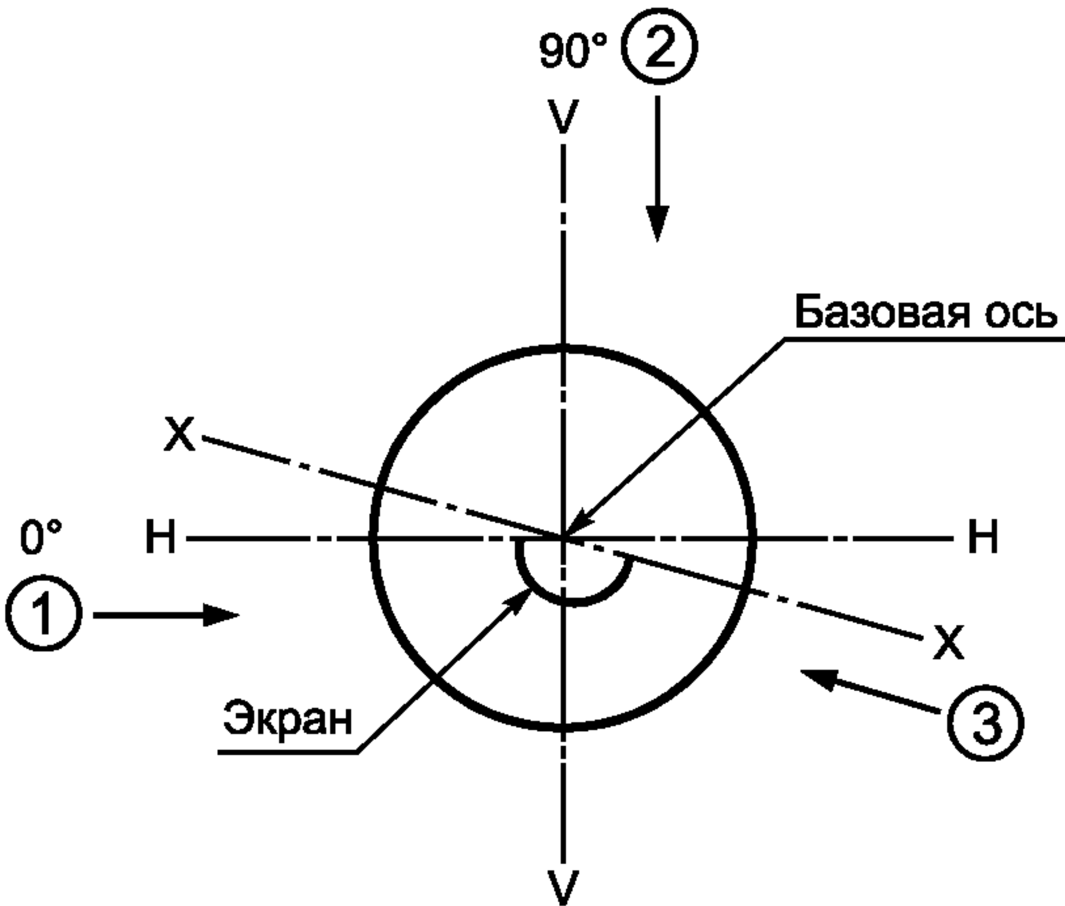
Рисунок D.1 — Направления видов, вид лампы сверху
