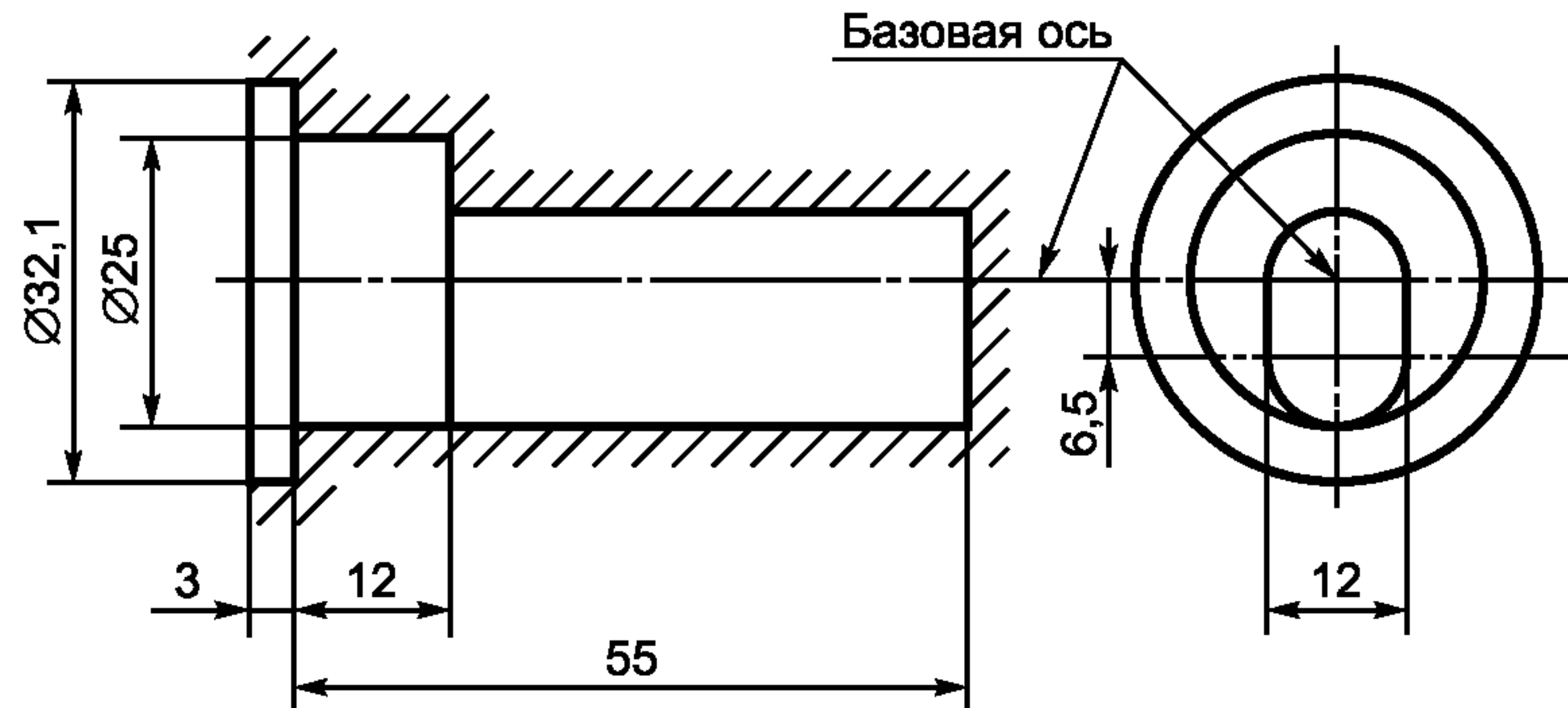
Рисунок 6 — Наибольший контур лампы 2)
