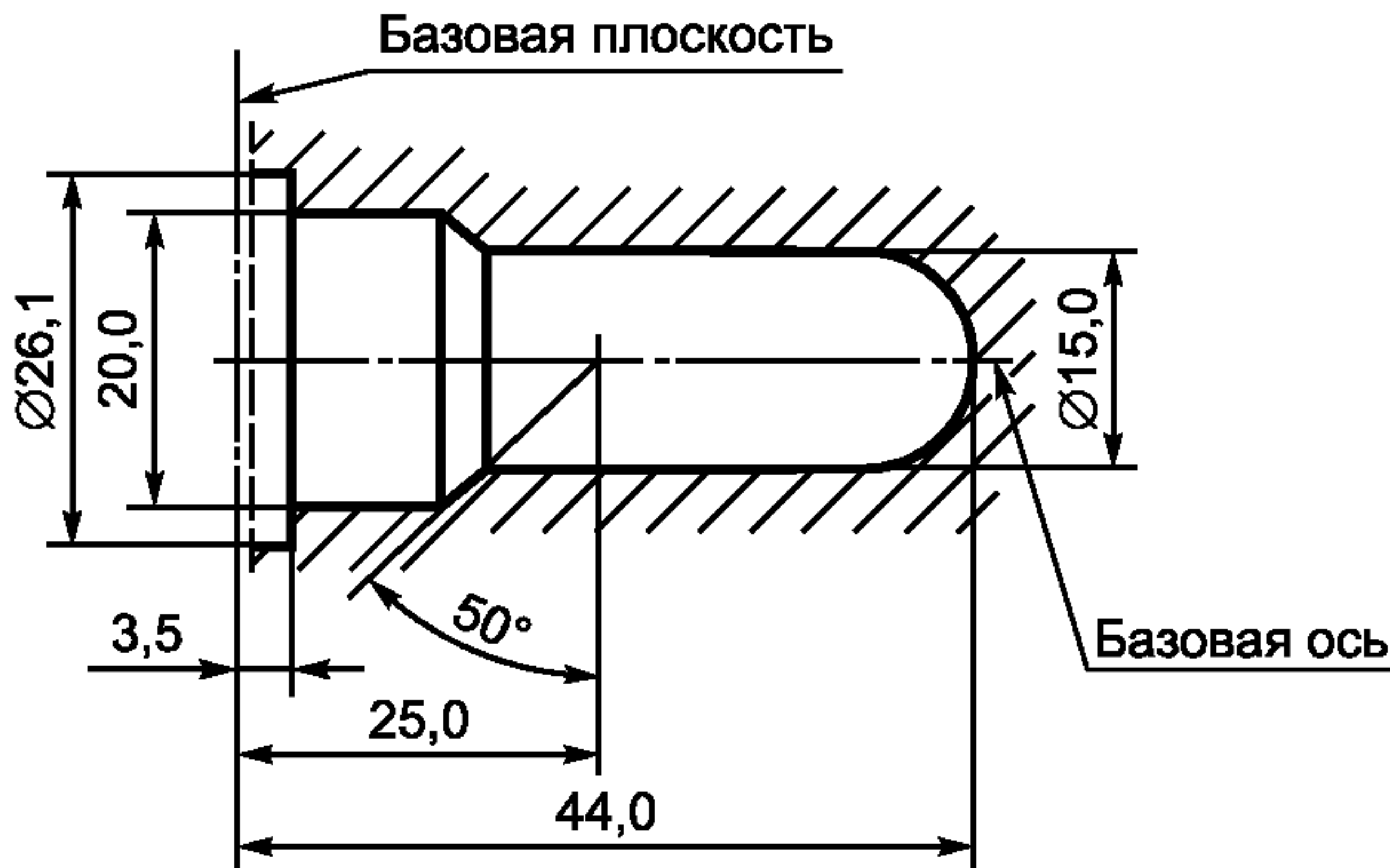
Рисунок 2 — Наибольший контур лампы
