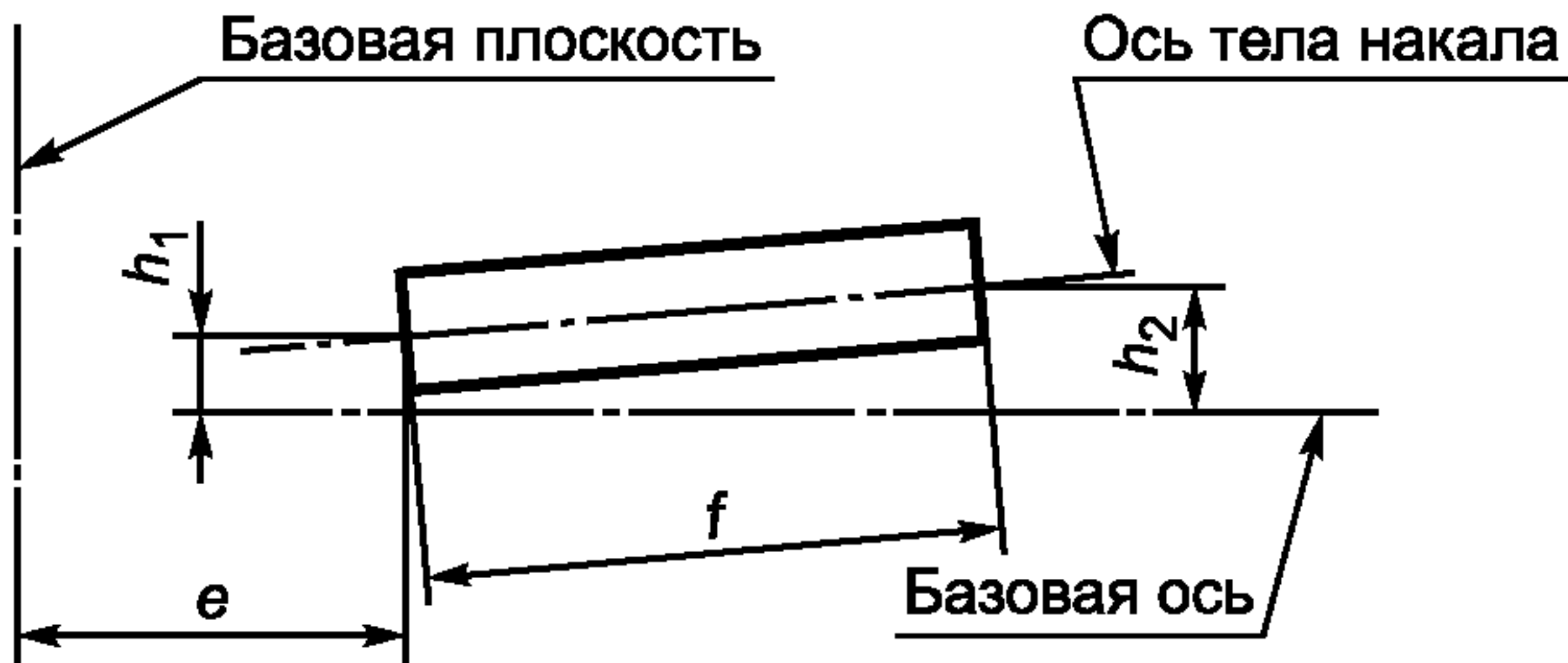
Рисунок 6 — Допустимое отклонение оси тела накала
