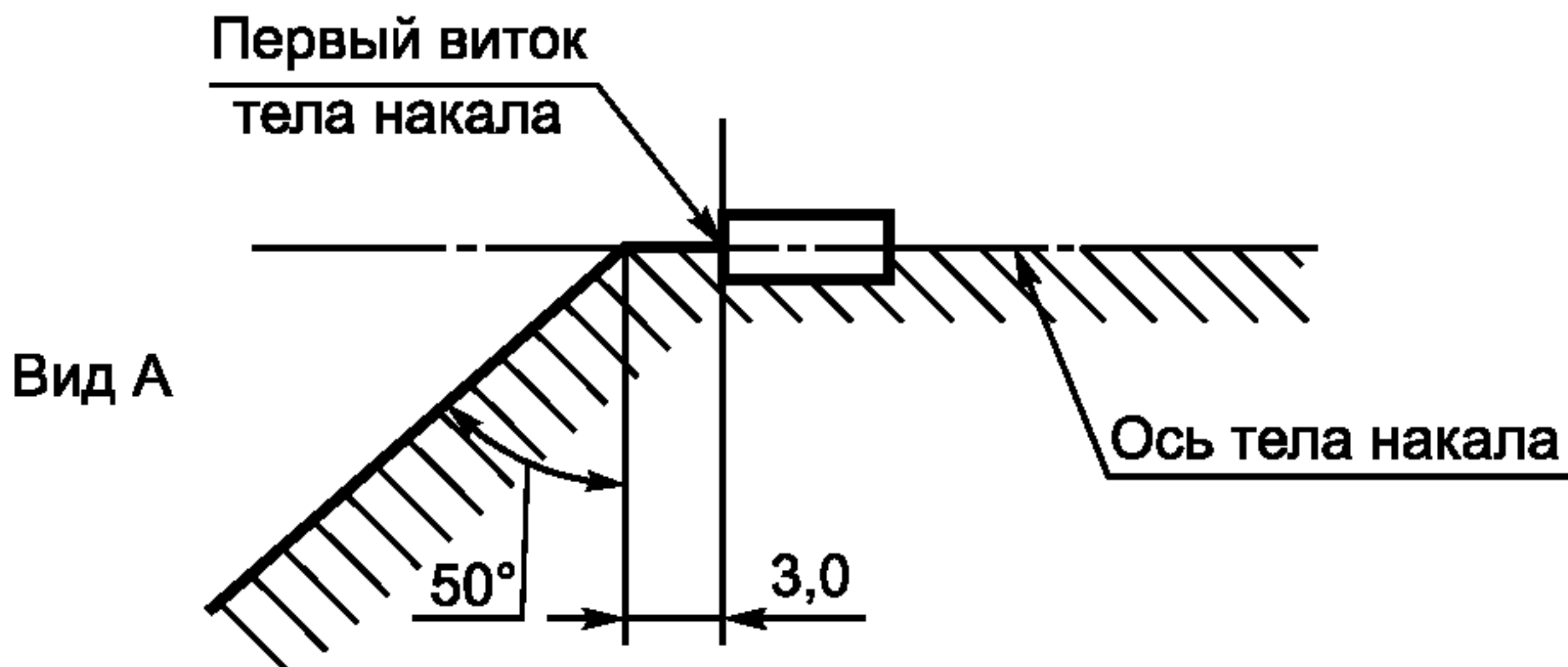
Рисунок 4 — Зона без металлических деталей
