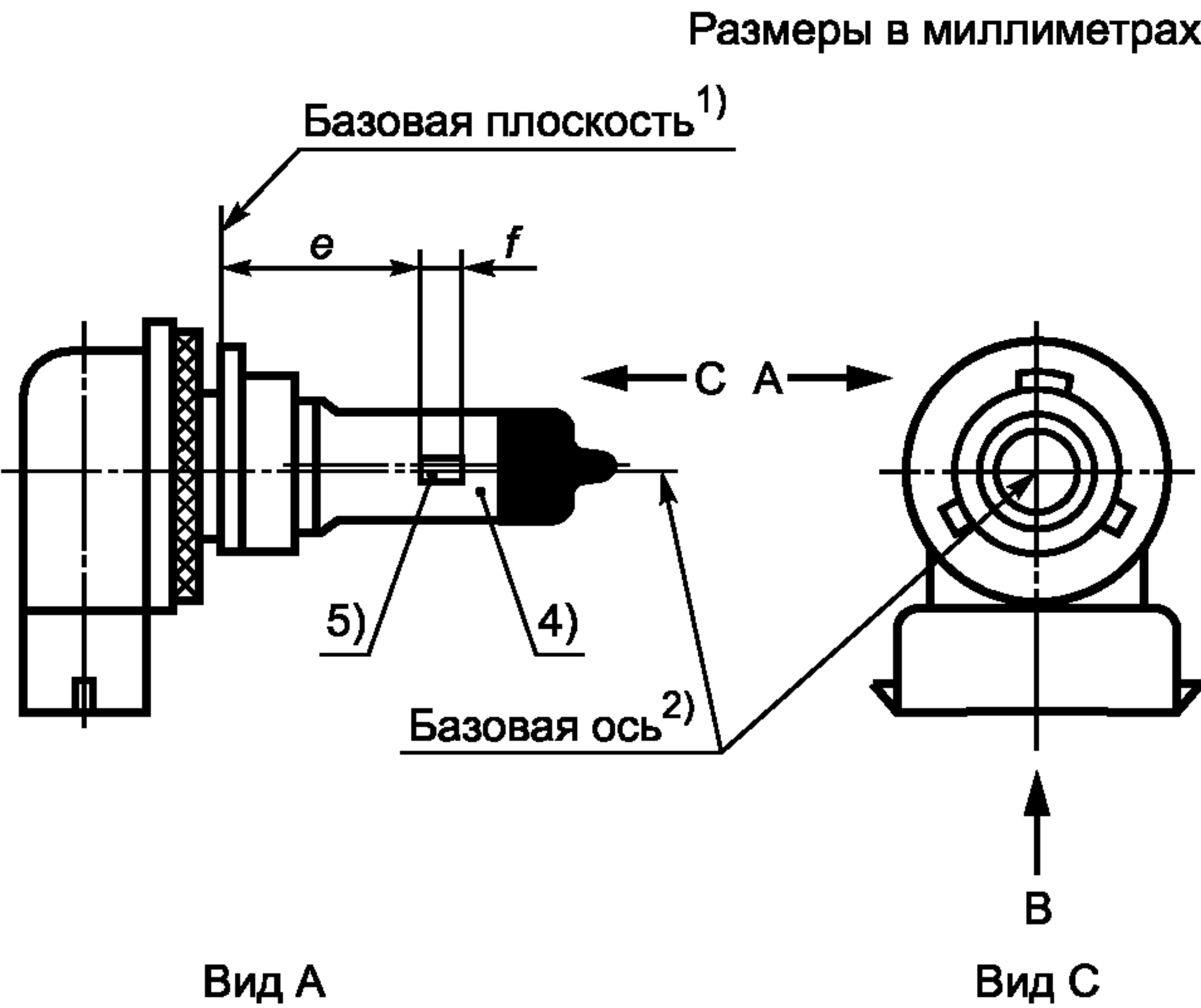
Рисунок 1 — Изображение лампы
