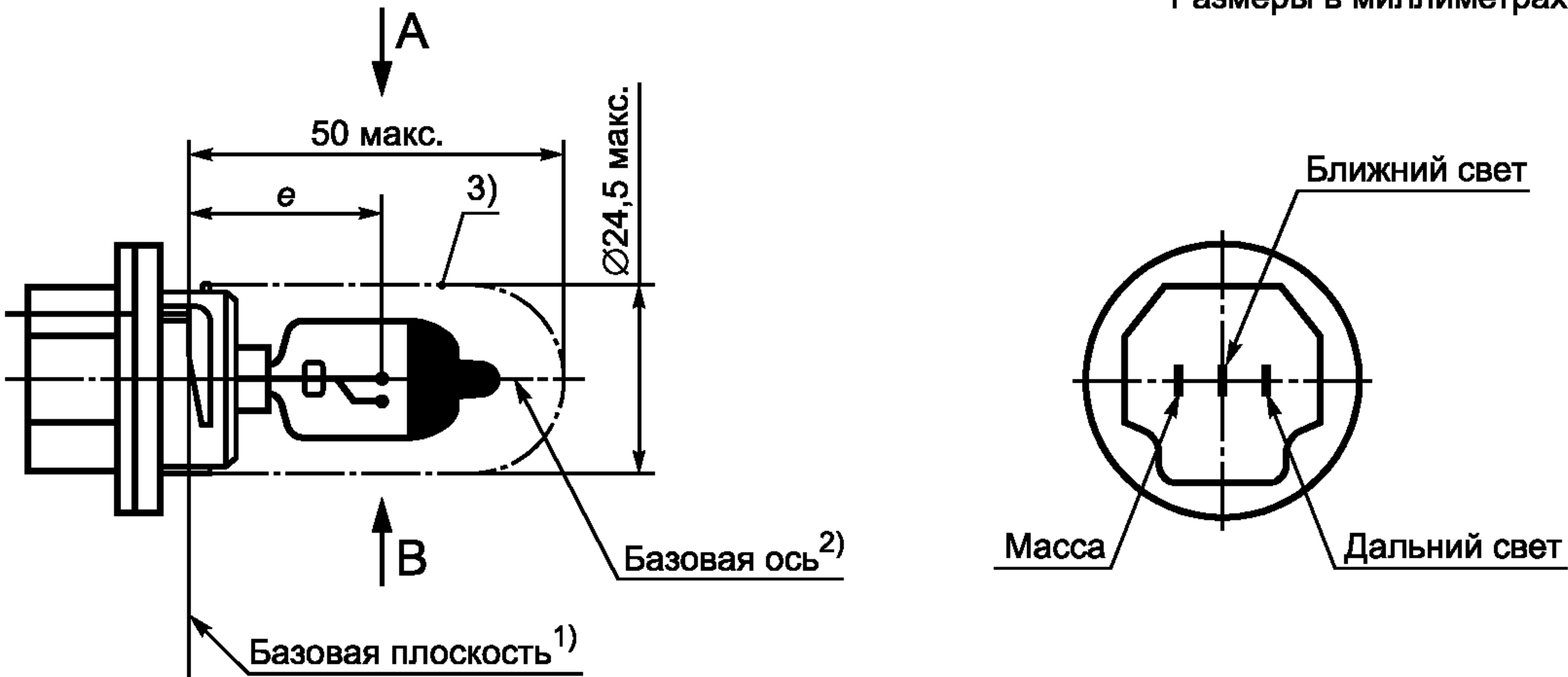
Рисунок 1 — Изображение лампы Цоколь P23t по МЭК 60061-1 (лист 7004-138)
