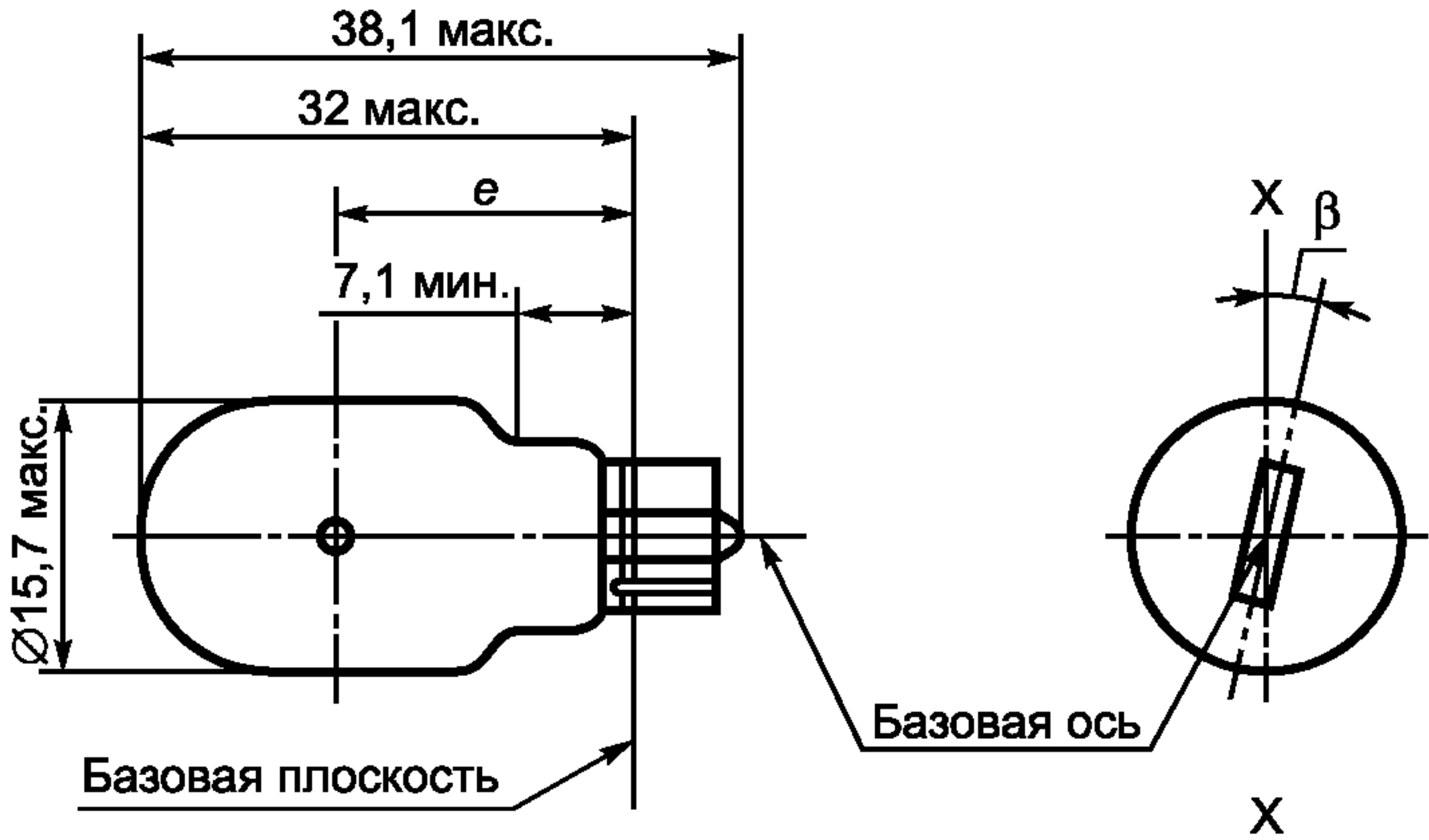
Параметры и размеры лампы накаливания
