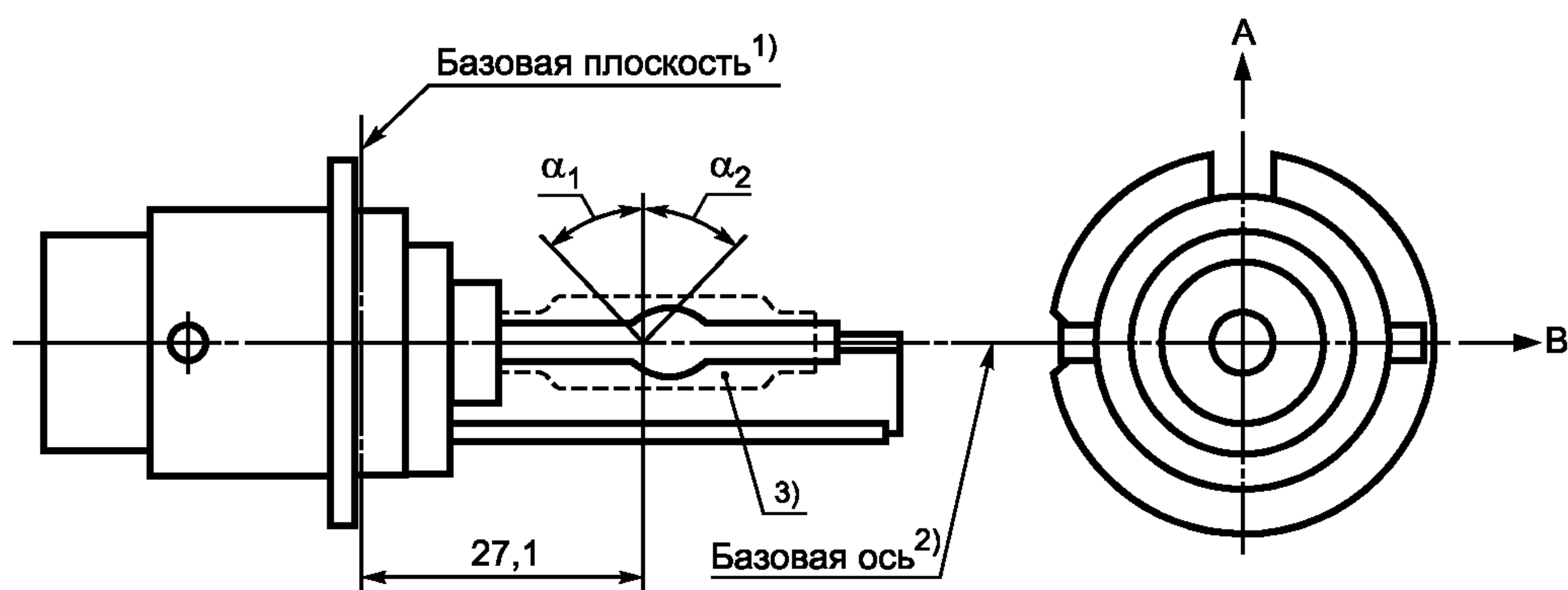
Рисунок 4 — Категория D4S, тип с соединителем, цоколь P32d-5
