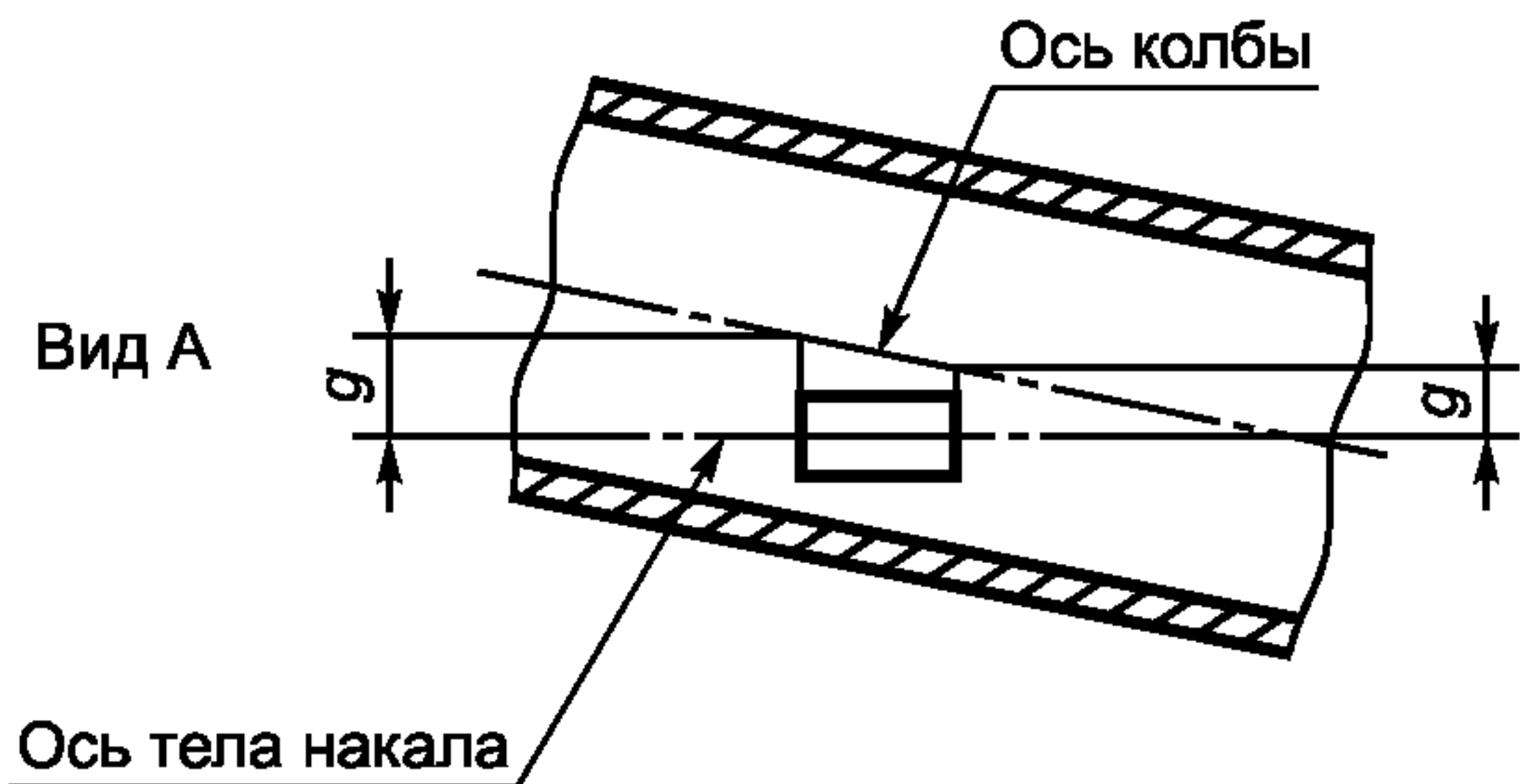
Рисунок 6 — Эксцентриситет колбы 10)
