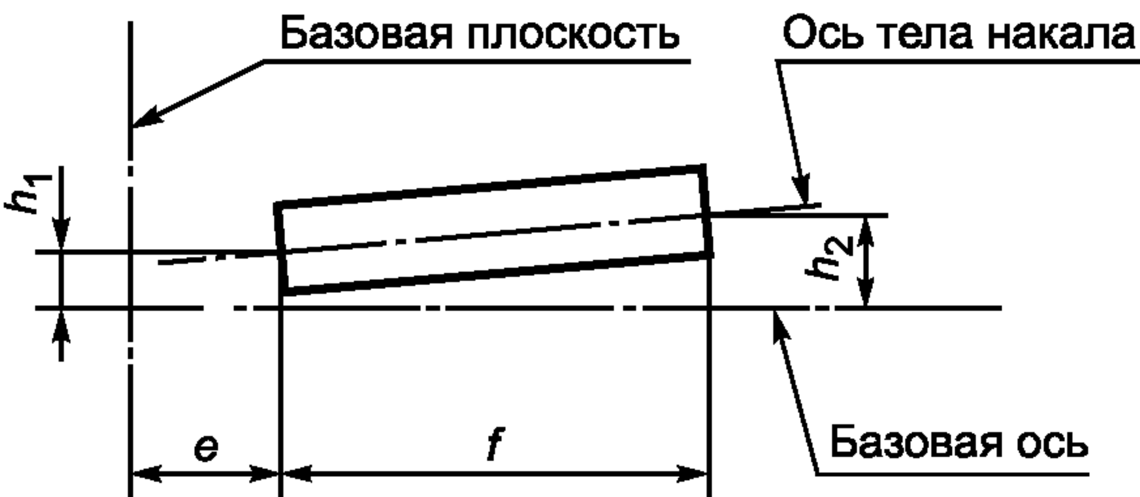
Рисунок 5 — Допустимое смещение оси тела накала 9)
