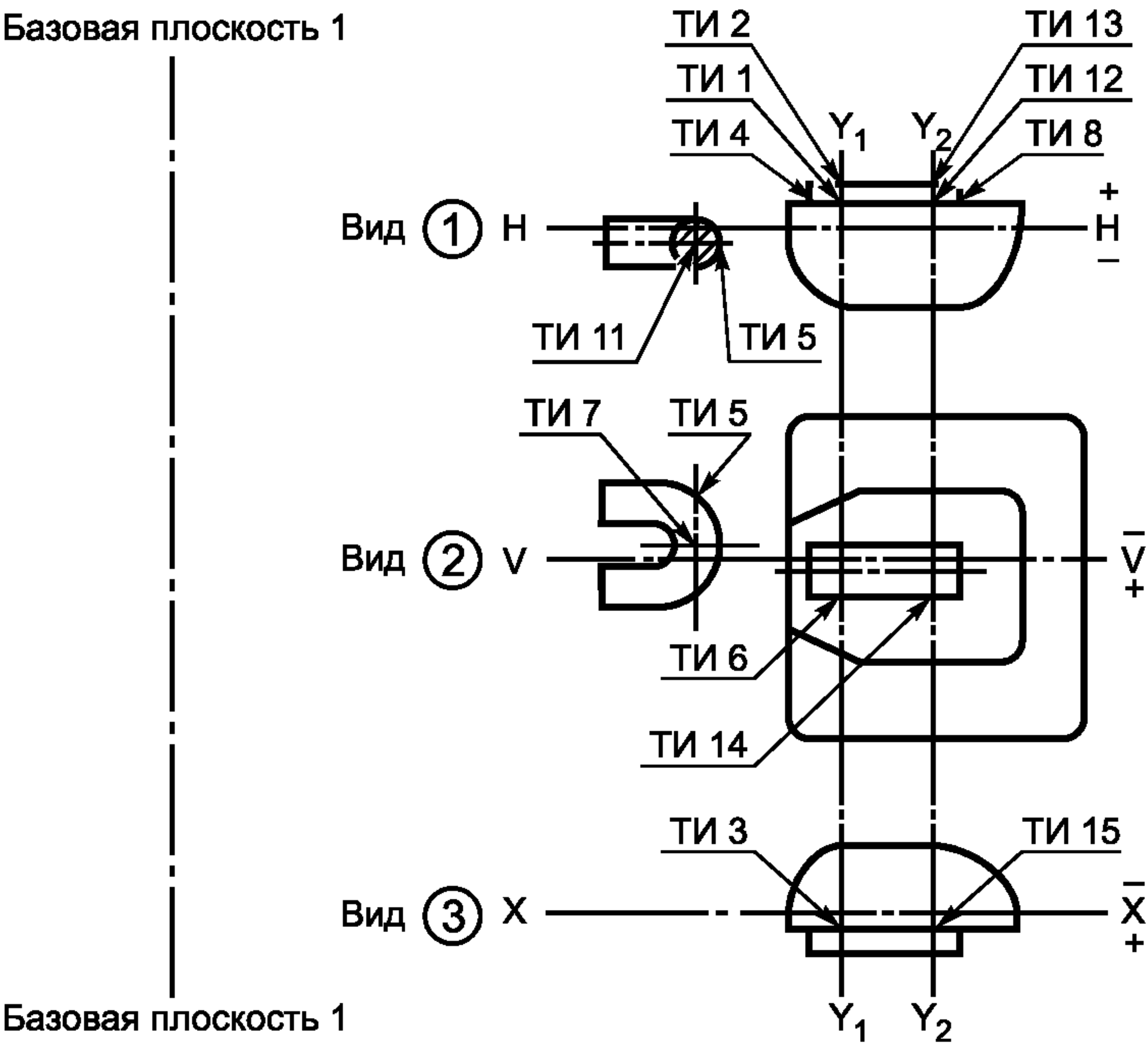
Рисунок D.2 — Положение измерительных точек ламп R2
