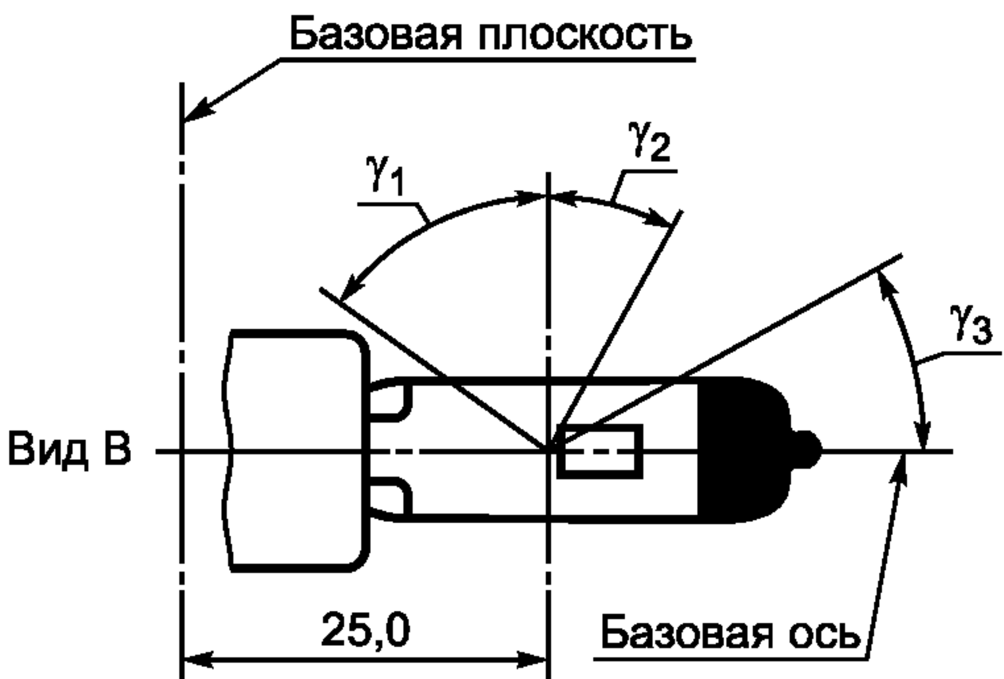
Рисунок 3 — Зона без искажений 6) и черный верх 7)
