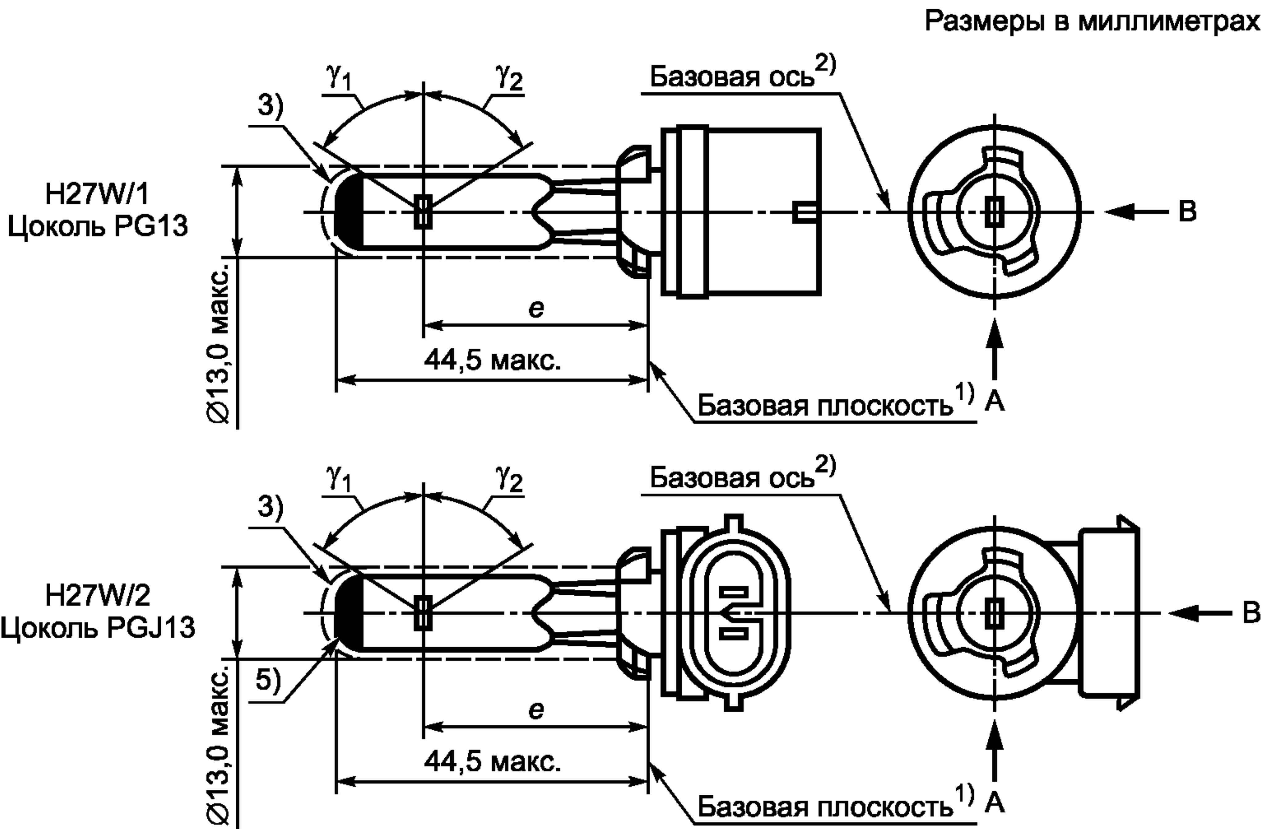
Рисунок лампы накаливания
