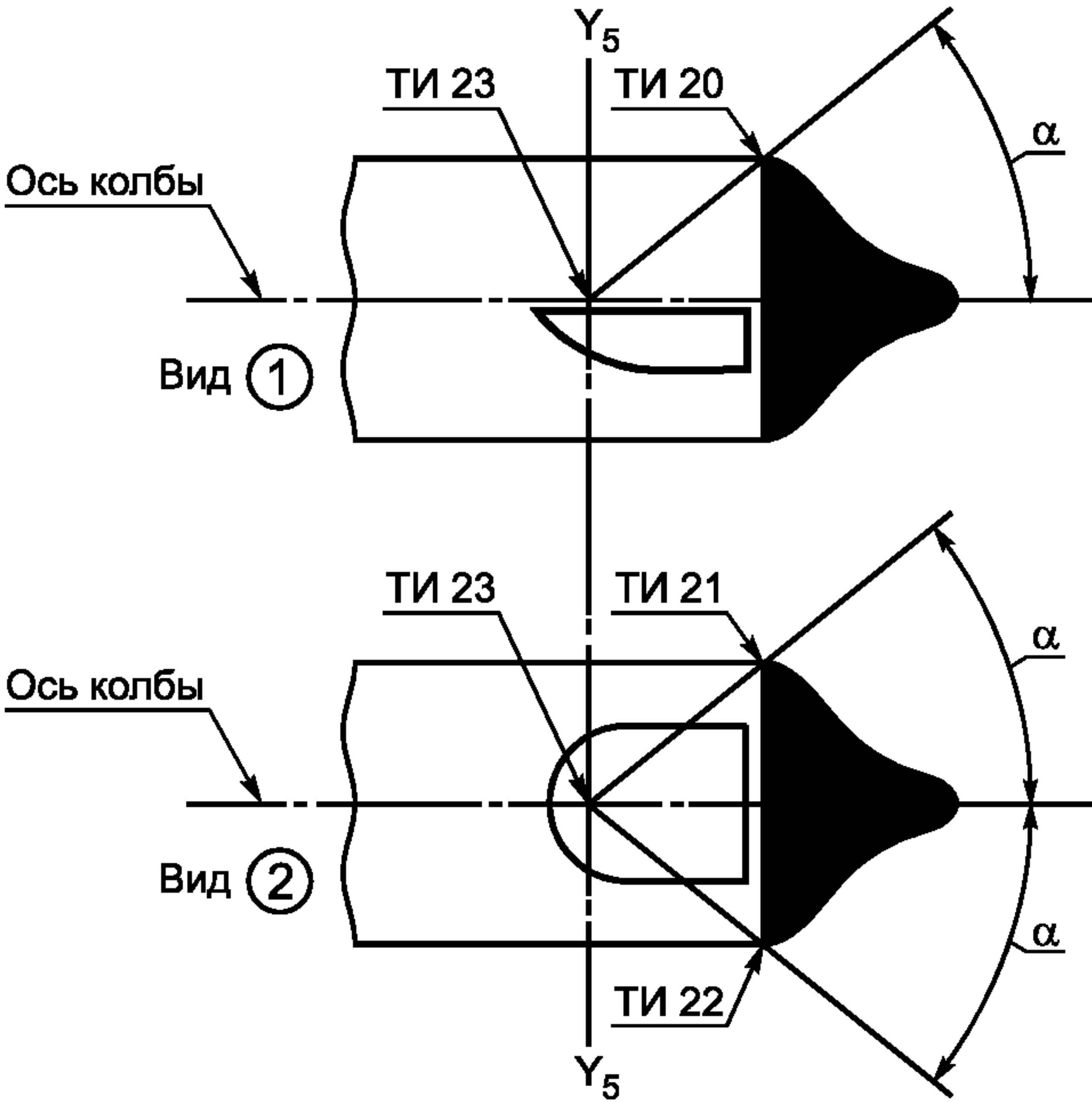
Рисунок Е.3 — Зачернение купола
