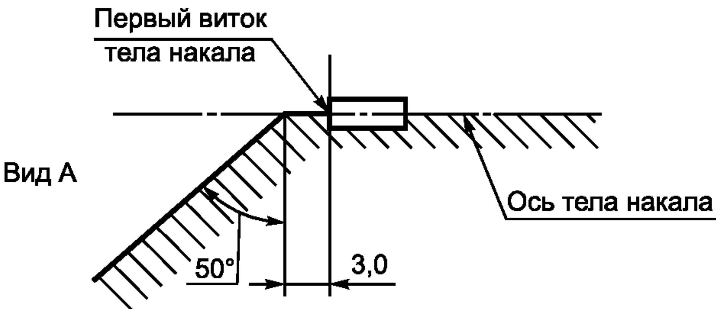
Рисунок 4 — Зона без металлических деталей 8)
