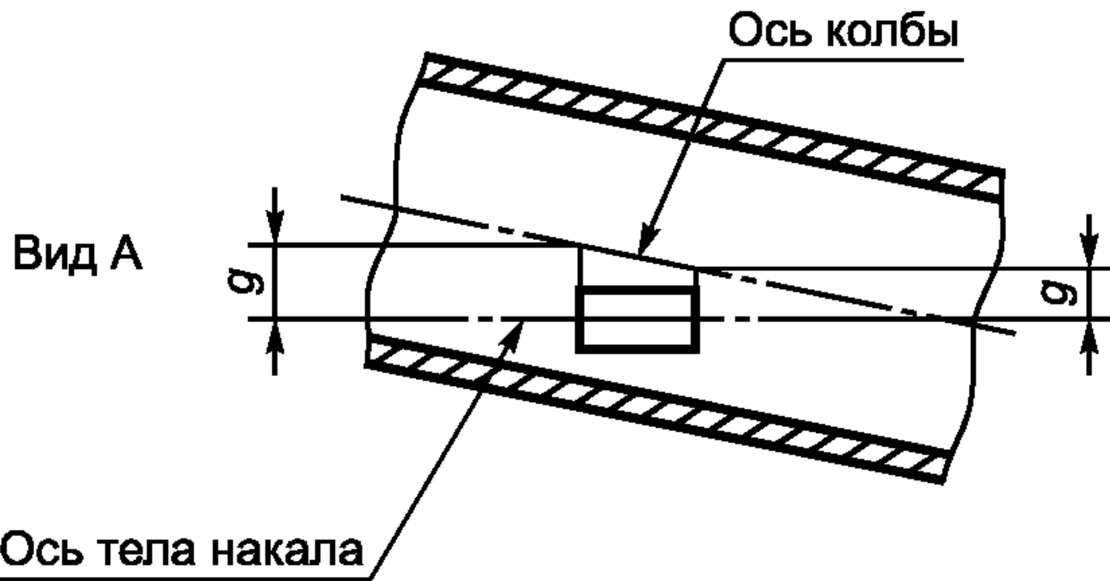
Рисунок 6 — Эксцентриситет колбы 10)
