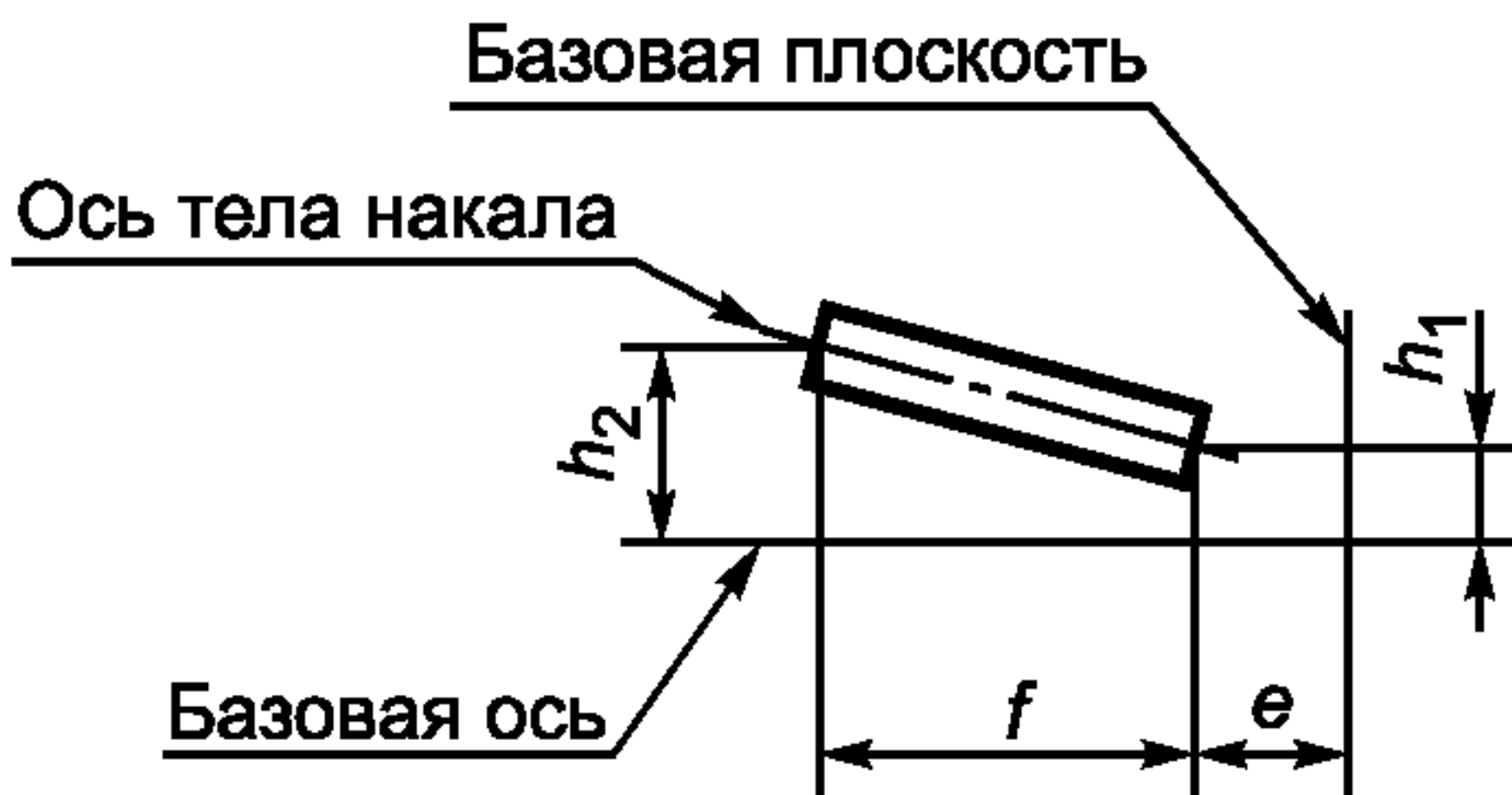
Рисунок 3 — Допустимое смещение оси тела накала 12)
