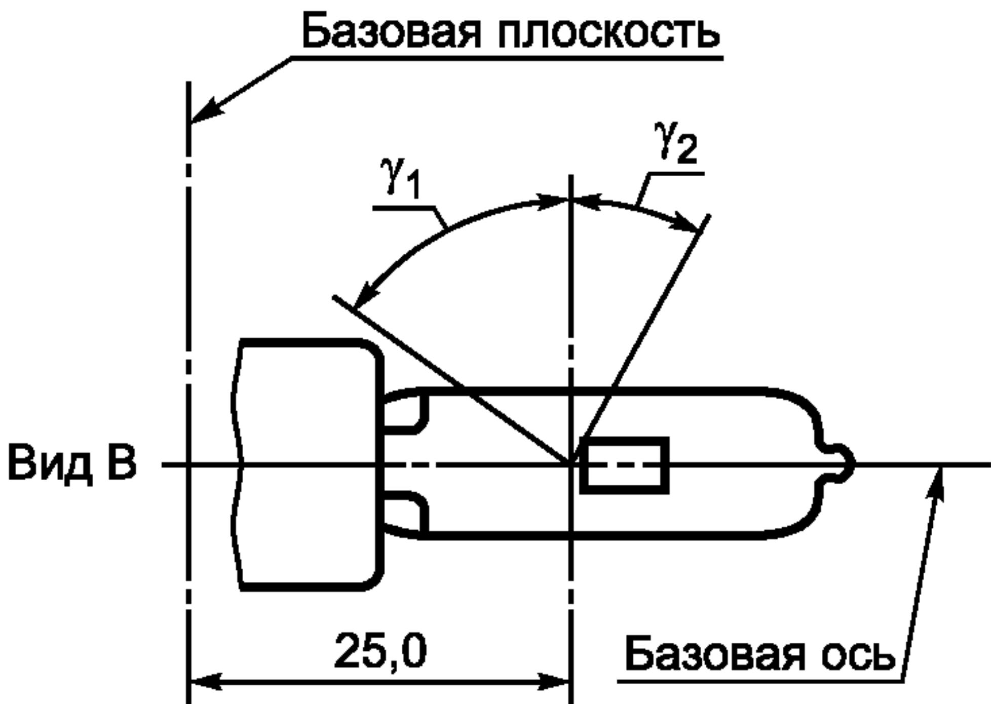
Рисунок 3 — Зона без искажений 5)
