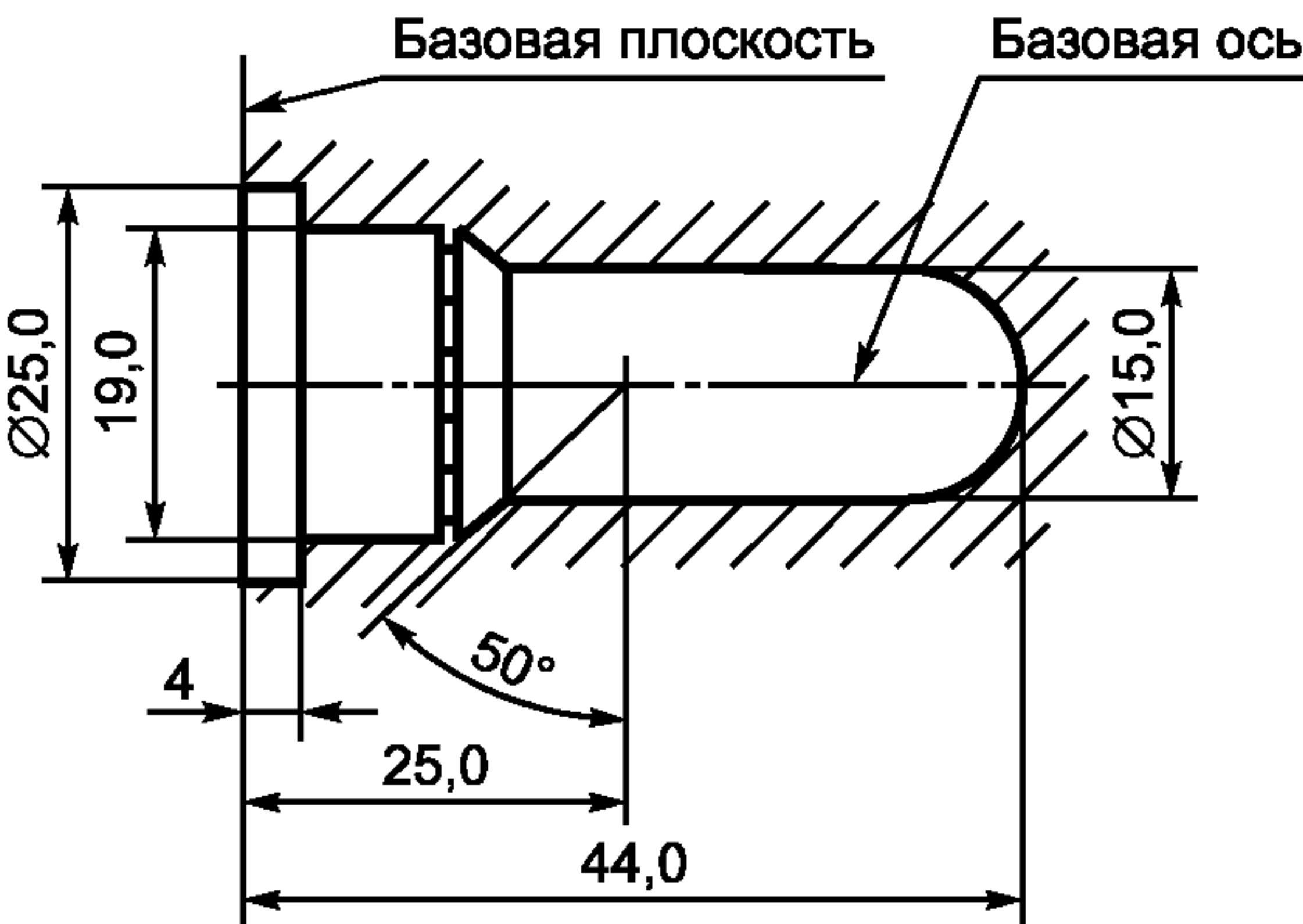
Рисунок 2 — Наибольший контур лампы 3)
