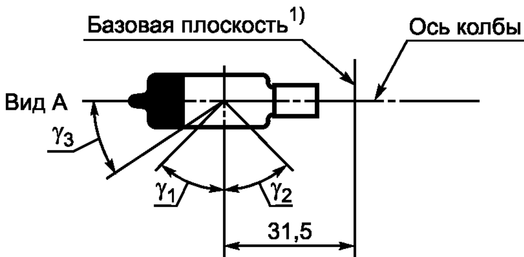
Рисунок 2 — Зона без искажений 6) и черный верх 7)
