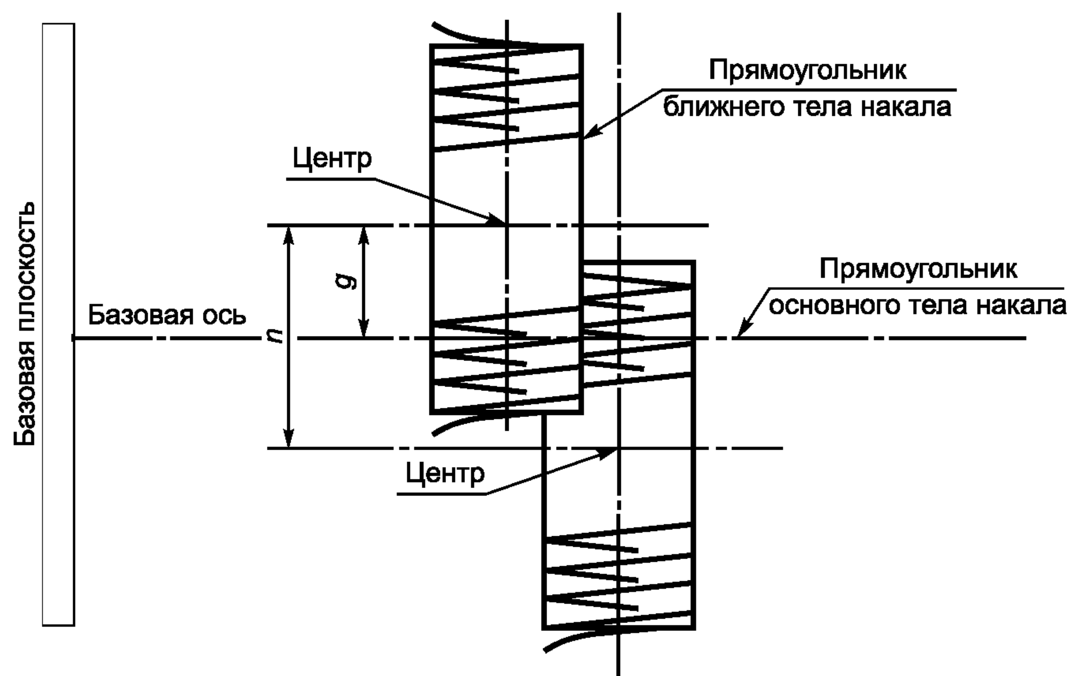
Рисунок F.2 — Вид в плане, вид с 4 1)
