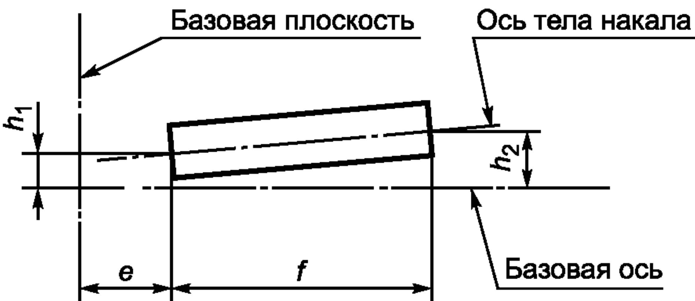
Рисунок 5 — Допустимое смещение тела накала 7) (только для эталонных ламп)
