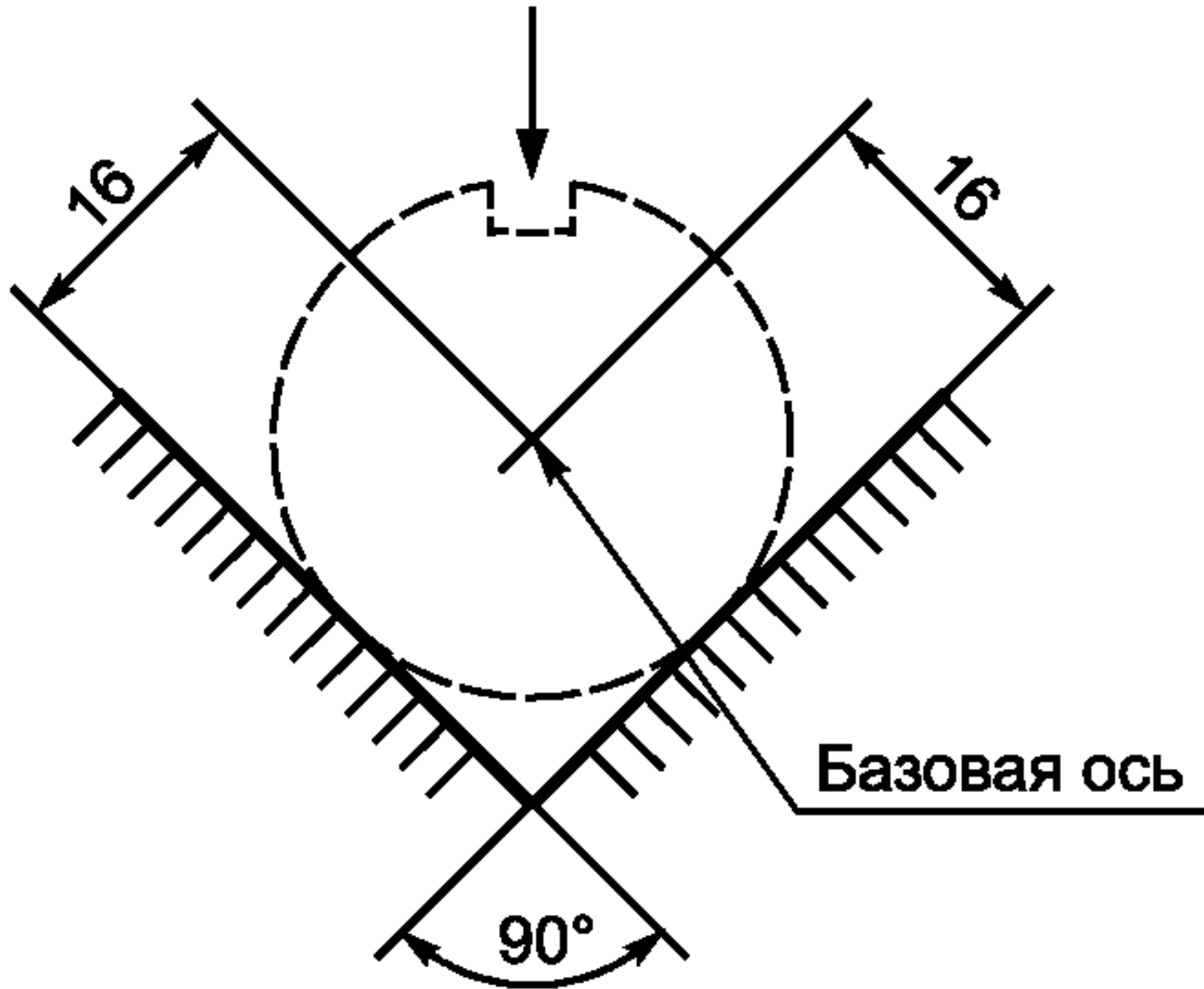
Рисунок 5 — Определение базовой оси 1)
