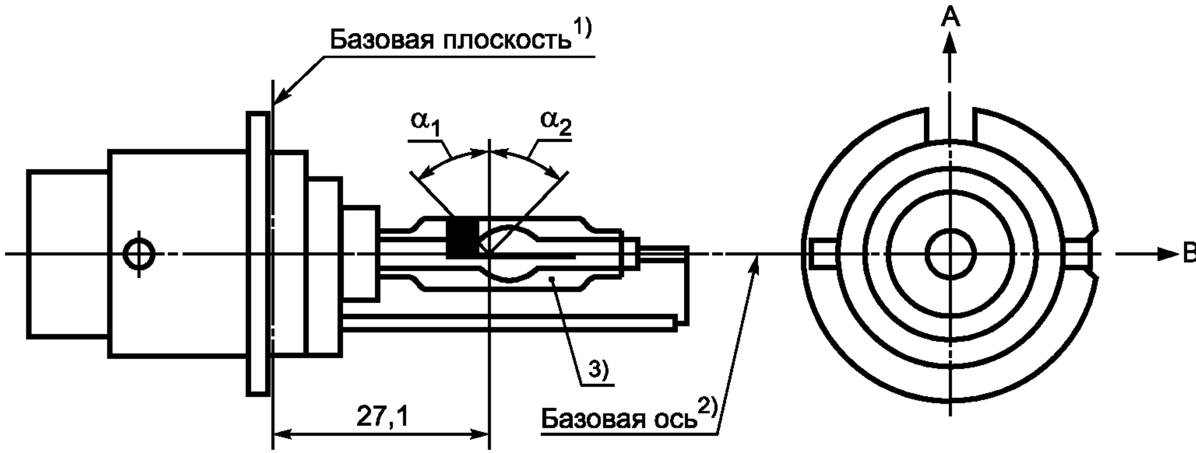
Рисунок 4 — Категория D4R, тип с соединителем, цоколь P32d-6
