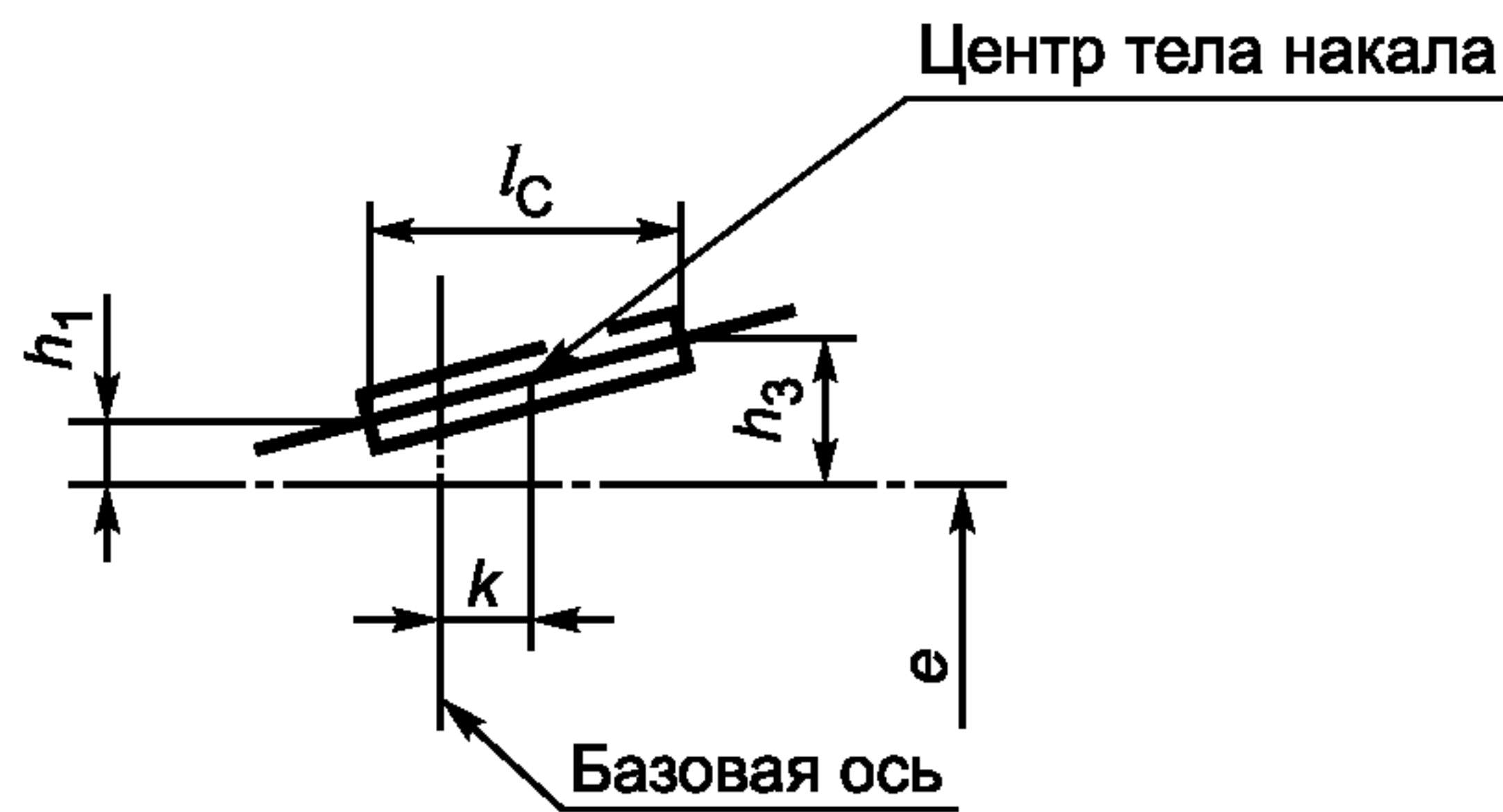
Вид А тела накала ближнего света
