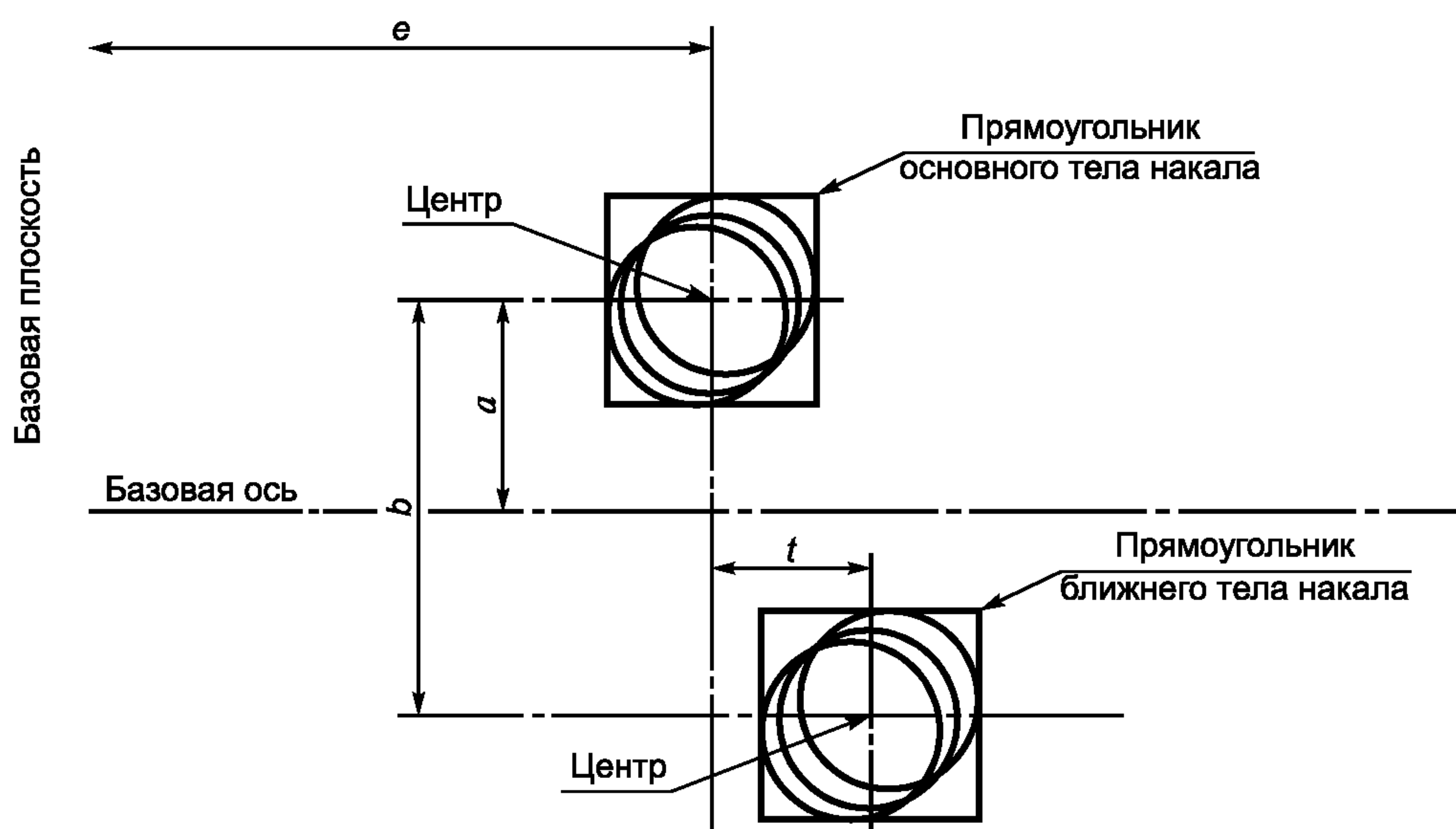
Рисунок F.1 — Вид сбоку, вид с 3 1), 2)
