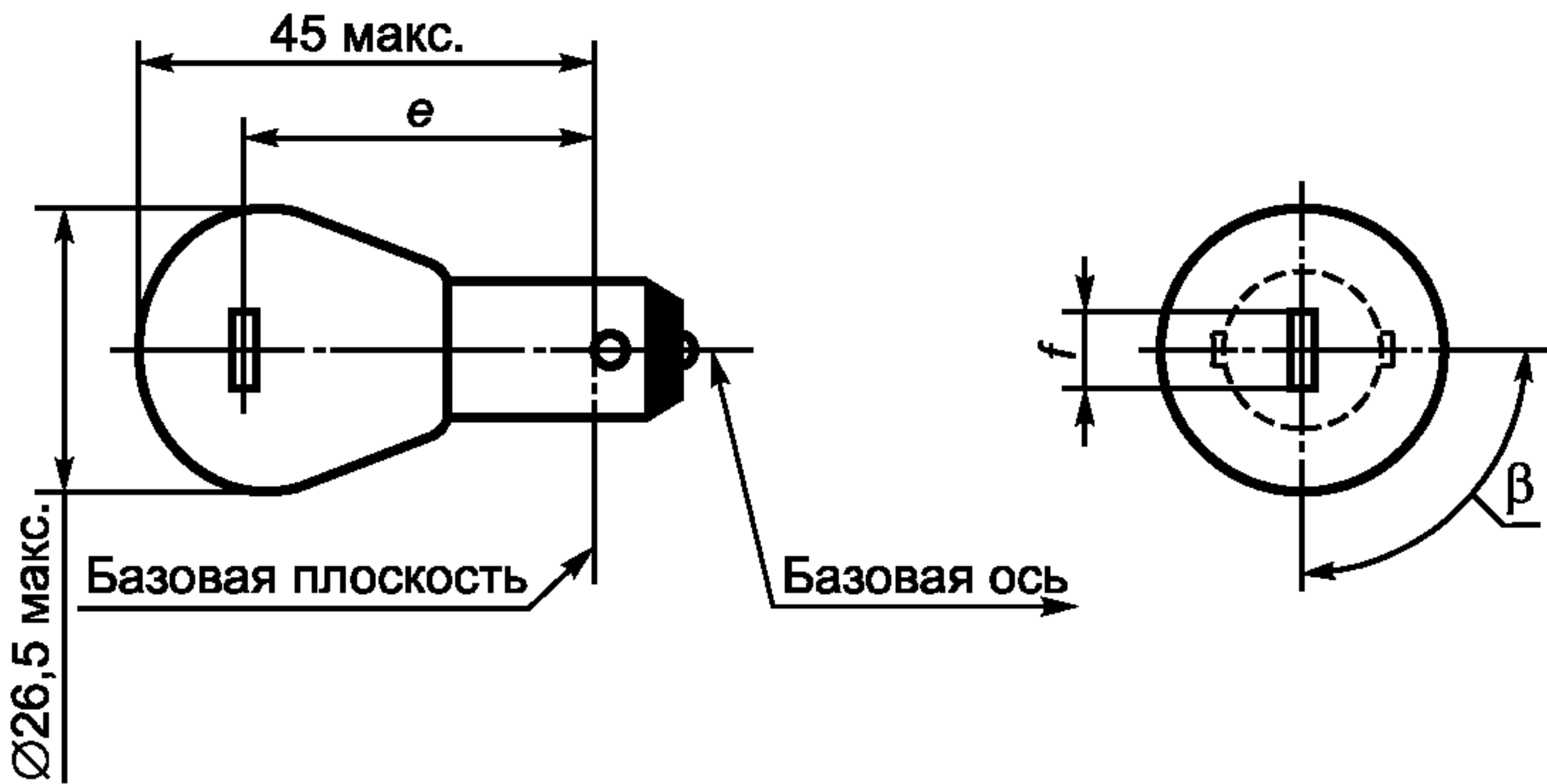
Вид тела накала, показывающий размерные линии e , f , g и \beta (не в масштабе)
