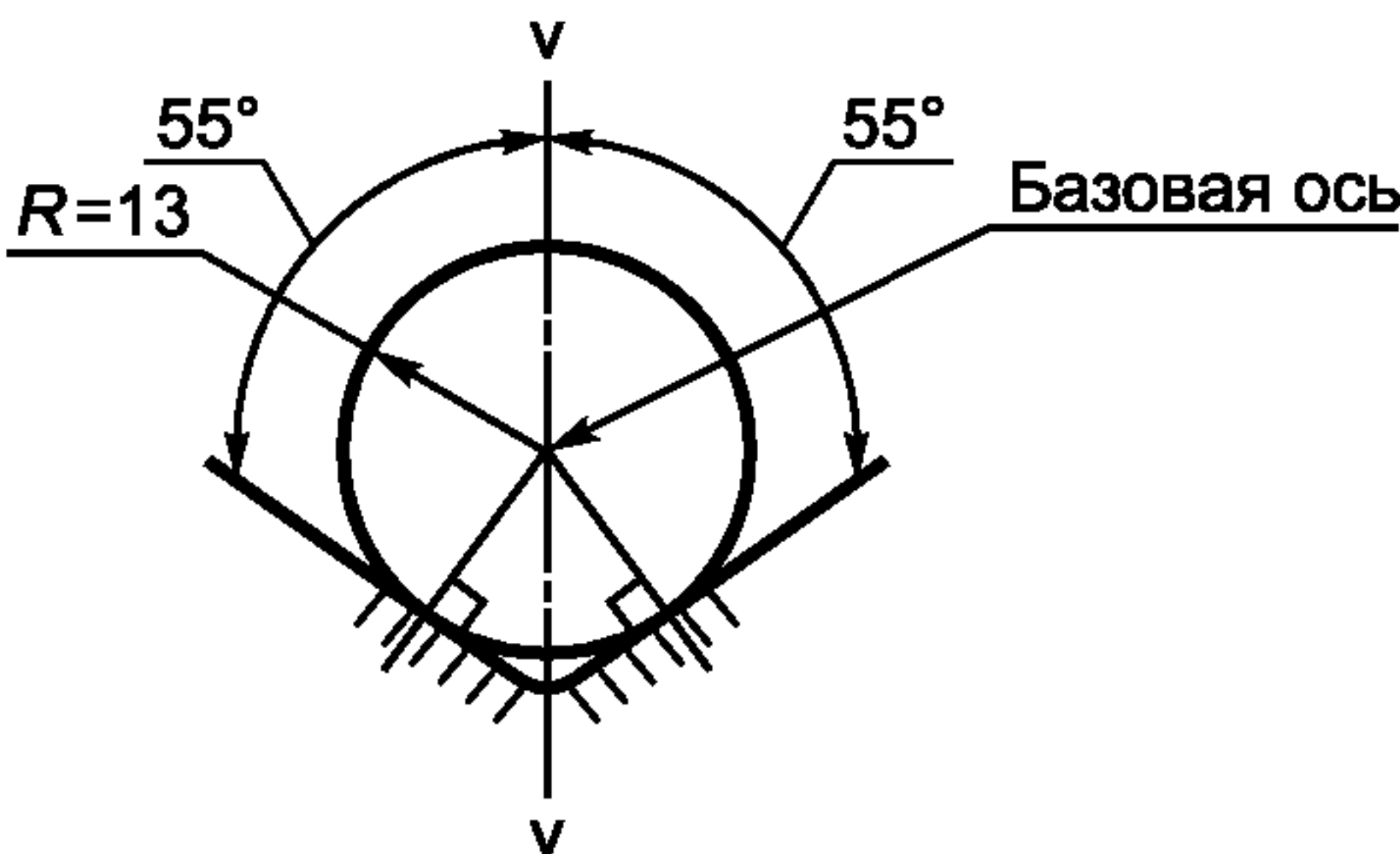
Рисунок 3 — Определение базовой оси
