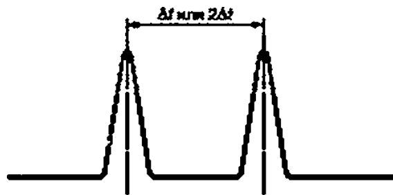
с — излучаемый импульс после настройки частоты повторения таким образом, чтобы второй импульс в канале 1 совпал с переданным импульсом в канале 2
