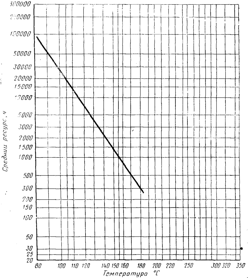
ГРАФИК ЗАВИСИМОСТИ СРЕДНЕГО РЕСУРСА ПРОВОДОВ ОТ ТЕМПЕРАТУРЫ
