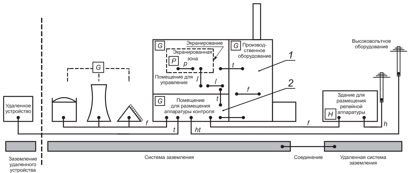
1 — Паровой котел, турбина, генератор, коммутационная аппаратура, оборудование подстанции среднего напряжения и т. д.; 2 — Аппаратура контроля и управления, электрические реле, преобразователи и т. д.
