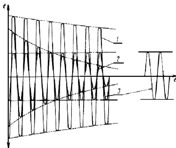
1 - свободная переходная составляющая; 2 - свободная сверхпереходная составляющая; 3 - принужденная составляющая
