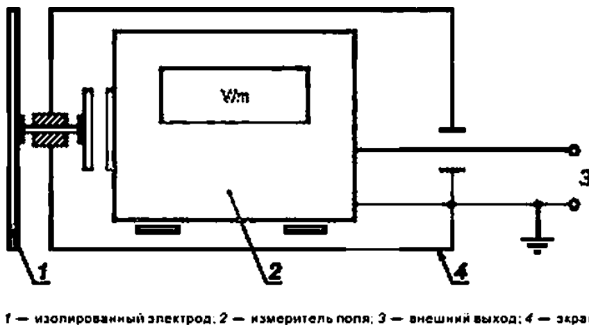
Рисунок 5 — Измеритель заряда пластины
