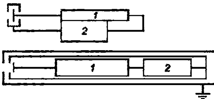
Рисунок 6 — Измеритель поля с обратной связью
