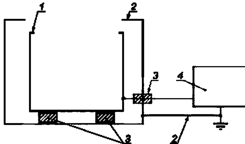
1 — внутренний контейнер; 2 — экран; 3 — изолятор; 4 — детектор
