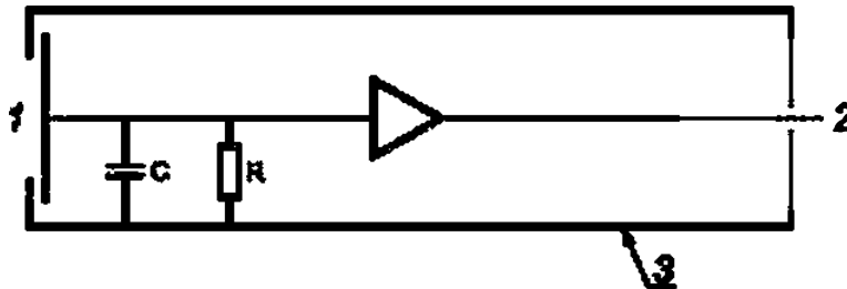
1 — чувствительная область; 2 — выход; 3 — экран; C — емкостное сопротивление; R — входное сопротивление
