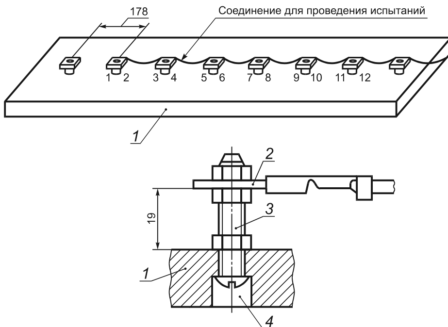
1 — плата из текстолита толщиной 19 мм; 2 — двусторонний штыревой наконечник; 3 — винт и гайка из стали; 4 — цинкованное углубление
