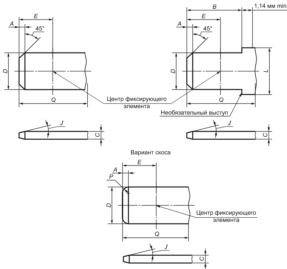
Рисунок 1 — Размеры штыревых контактов (штекеров)
