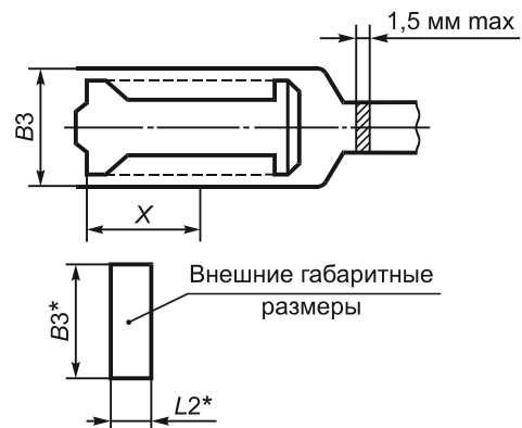
Рисунок 5 — Размеры гнездовых наконечников
