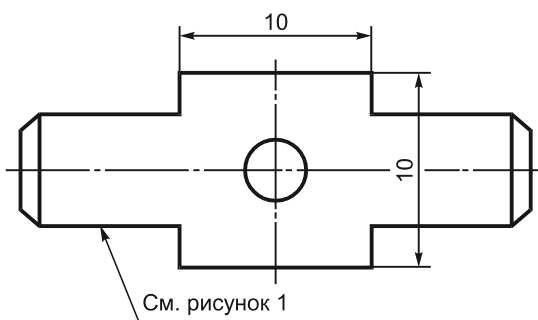
Рисунок 6 — Двухконцевой штекер
