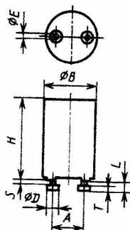
Размеры стартеров
