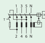
4-х полюсные
