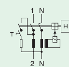
2-х полюсные
