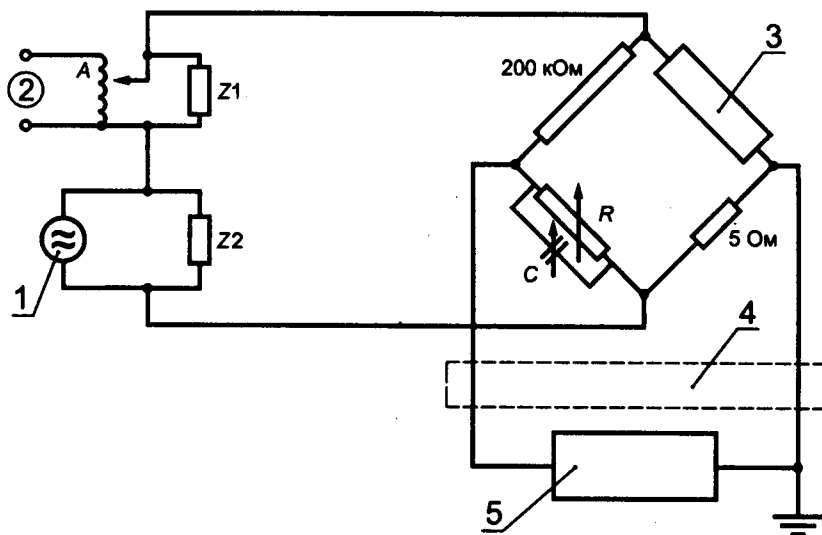
Рисунок А.1 — Измерение токов
