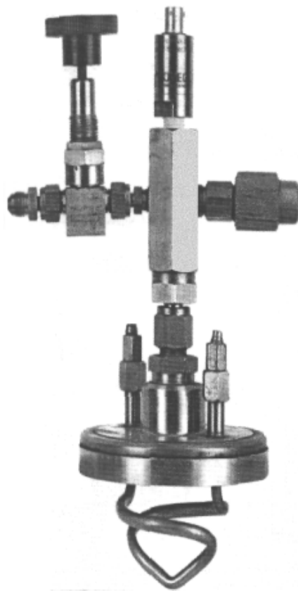
Рисунок 3 — Крышка с охлаждающим змеевиком
