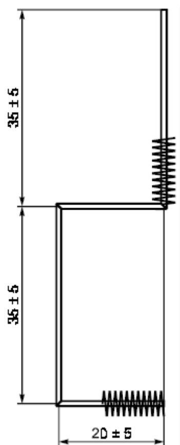
Рисунок 4 — Пример держателя для испытания на облуживание
