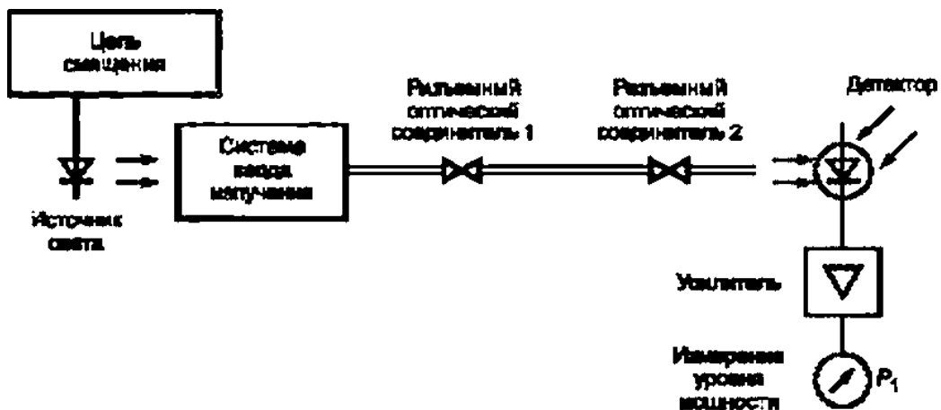
Рисунок В.1 — Калибровка установки для измерения вносимых потерь
