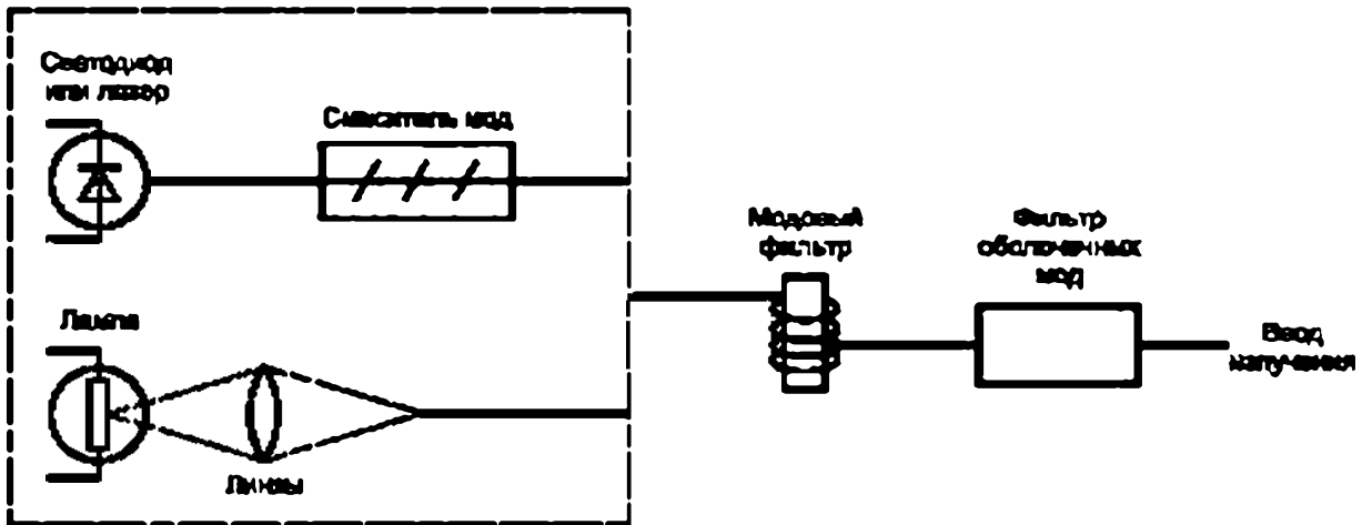
Рисунок A.3 — Общая схема ввода излучения
