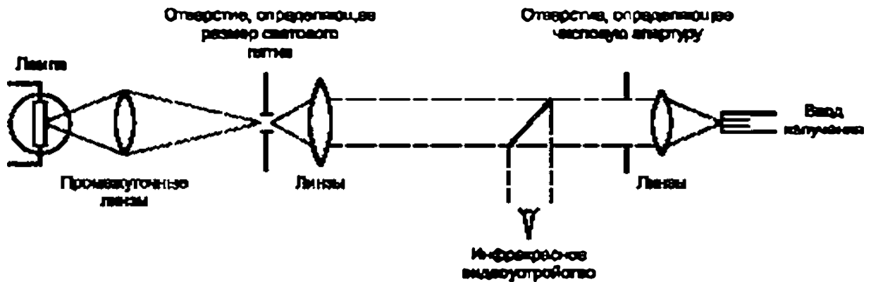
Рисунок А.4 — Оптическая система возбуждения с помощью ограниченного фазового пространства
