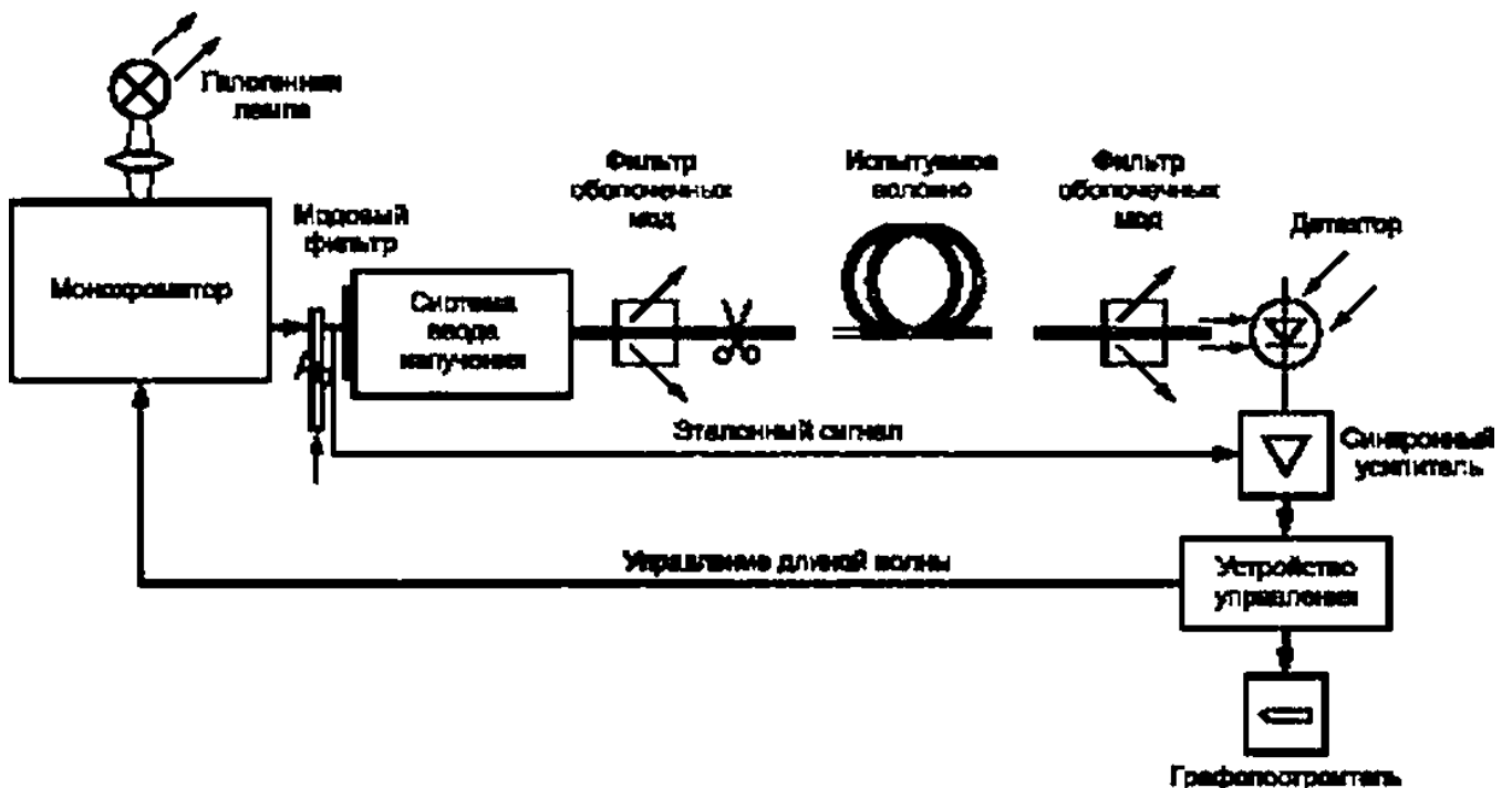
Рисунок А.2 — Расположение оборудования, используемого для получения спектра потерь
