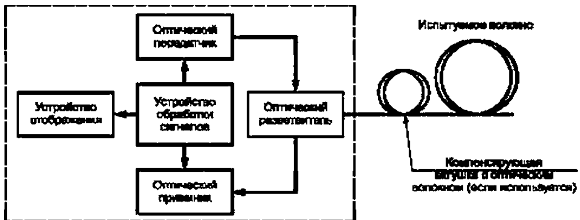
Рисунок С.1 — Блок-схема ОРВО
