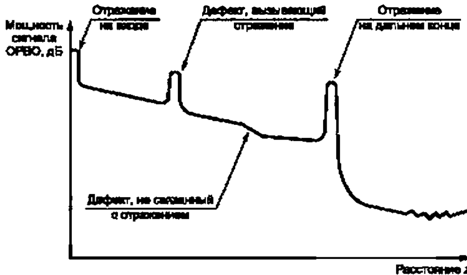
Рисунок С.4 — Схематическая линия ОРВО, показывающая видимые потери вследствие точечных дефектов, один — отражающий и один — не отражающий
