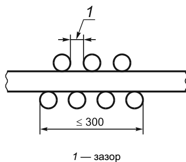
Рисунок 1 — Типичное расположение с зазором кабелей, закрепленных на обеих сторонах стандартной лестницы (категория A F/R)
