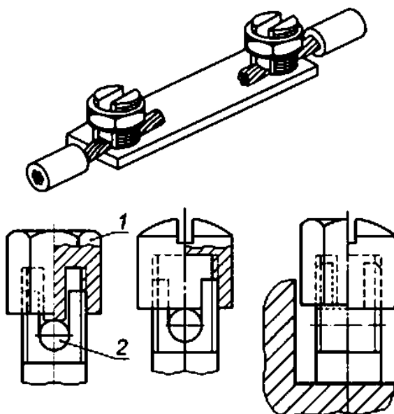
Рисунок S — Зажимы для кабельных наконечников
