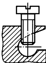
Торцевые зажимы с прямым усилием прижатия жилы проводника без прижимной пластины
