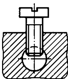
Торцевые зажимы с прямым усилием прижатия жилы проводника без прижимной пластины
