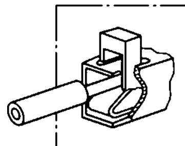
Рисунок 6 — Примеры безвинтовых контактных зажимов
