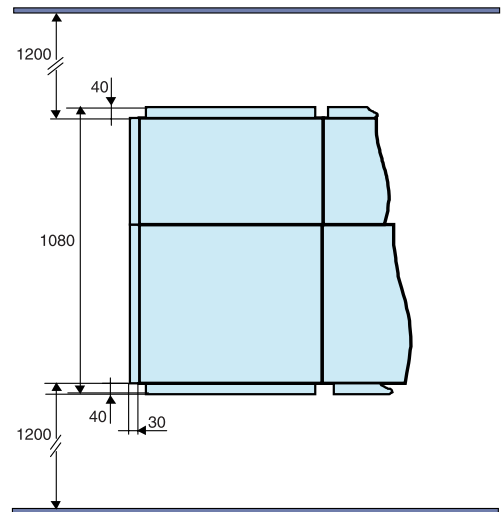
Ячейка с задним присоединением глубиной 1000 мм: минимальное пространство спереди и сзади
