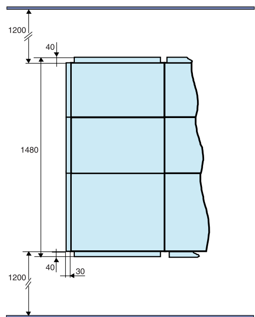
Ячейка с задним присоединением глубиной 1400 мм: минимальное пространство спереди и сзади
