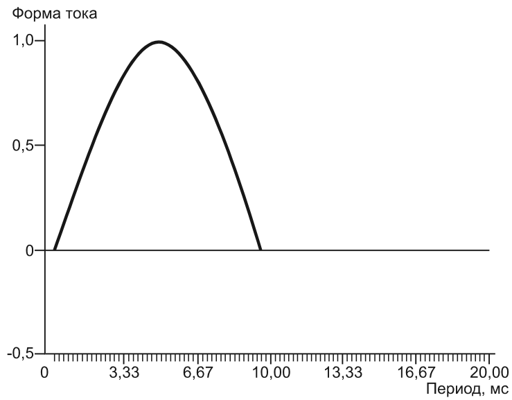
Рисунок А.2 — Форма тока при однополупериодном выпрямлении
