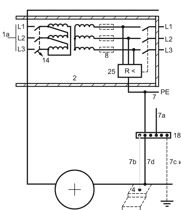
Рисунок 717.5 — Пример соединения с простым разделением и IT-системой с устройством контроля изоляции и отключением после первого замыкания на землю
