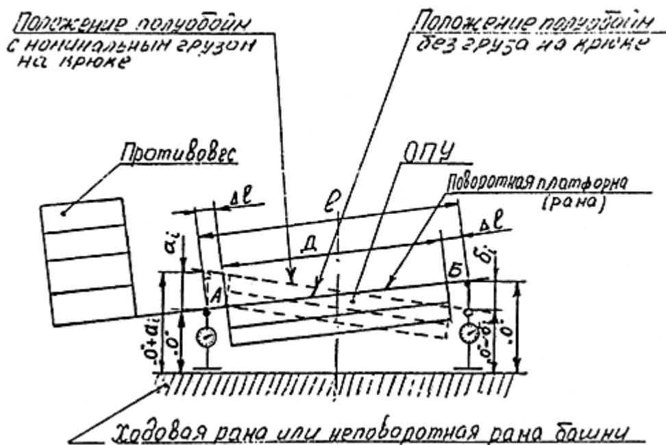
Рис. ИЗ-1. Схема для измерения линейных перемещений полуобойм ОПУ башенных кранов D - диаметр полуобоймы; \Delta l - расстояние от полуобоймы до оси ножки индикатора; l - расстояние между ножками индикаторов; a и b - линейные перемещения (по шкале индикаторов); "0" - установочная высота индикатора
