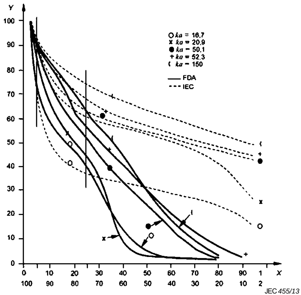
Рисунок 0.3 — Нормированные значения площади поперечного сечения пучка при ограничениях FDA и IEC для пяти преобразователей с различными ka при z = 0.5 см
