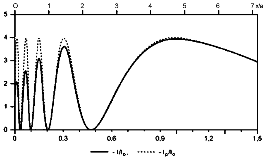
Рисунок А.1 — Осевая зависимость нормированной усредненной по времени акустической интенсивности (сплошная линия) и ее плоско-волновой аппроксимации (штриховая линия) для круглого поршневого излучателя с ka \gg 30 от нормированного расстояния a (где s = Xz/a^2 )
