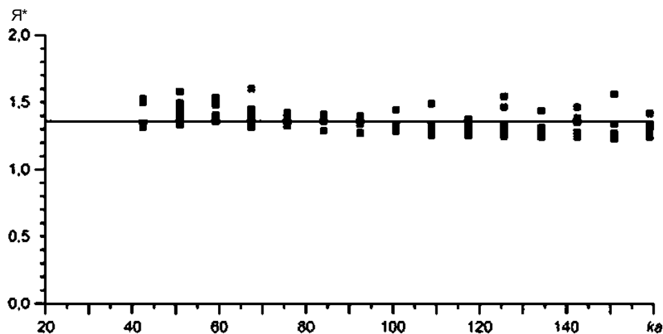
Рисунок Е.1 — Коэффициент преобразования F_k как функция значений ka , лежащих в диапазоне от 40 до 160
