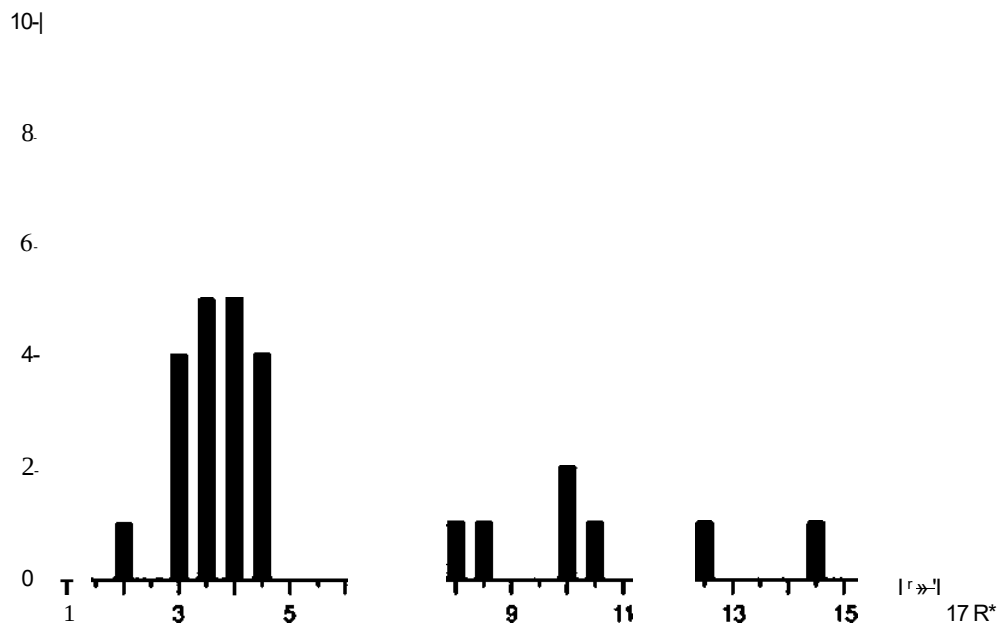
Рисунок А.2 — Гистограмма распределений значений I_{BN} для 37 лечебных головок различных диаметров и частоты
