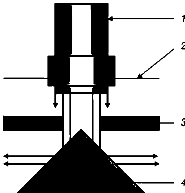
1 — лечебная головка; 2 — поверхность аоаы; 3 — апертурная маска; 4 — мишень измерителя радиационной силы
