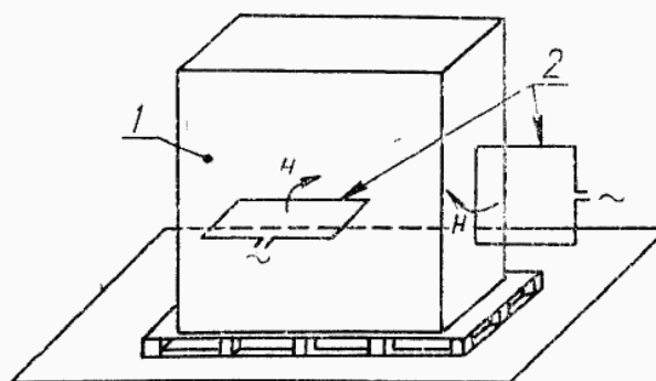
Рисунок 6 — Схема проверки восприимчивости ИТС к ИМП с использованием метода приближения
