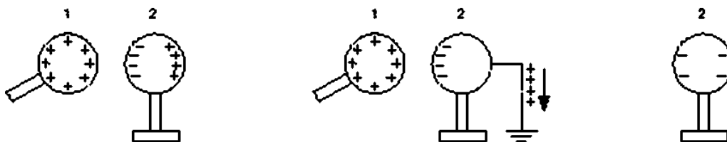
1а) – Сближение заряженного объекта (1) с незаряженным объектом (2)
