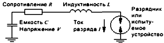
Рисунок 5 – Принципиальная схема устройства для моделирования разрядов статического электричества
