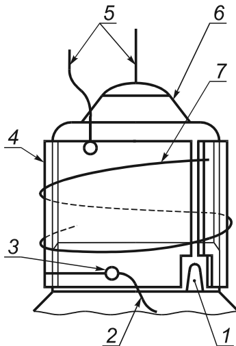
Испытательный патрон для ламп с резьбовым цоколем
