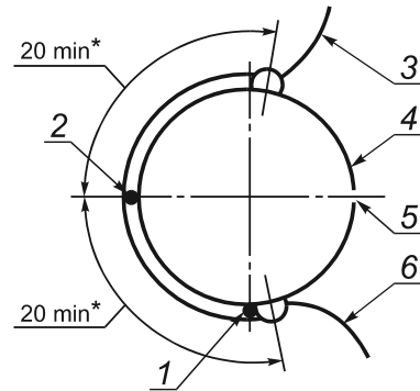
Положение испытательного патрона и термопреобразователя
