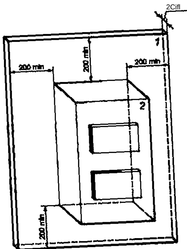
Рисунок 101 - проверка максимальной способности рассеивания мощности P_{0e} на поверхности типового корпуса
