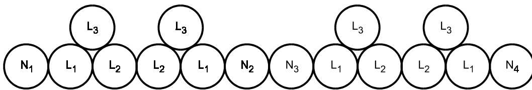
Рисунок Н.52.9 — Специальная конфигурация для 12 параллельных одножильных кабелей, уложенных треугольником (см. 523.7)
