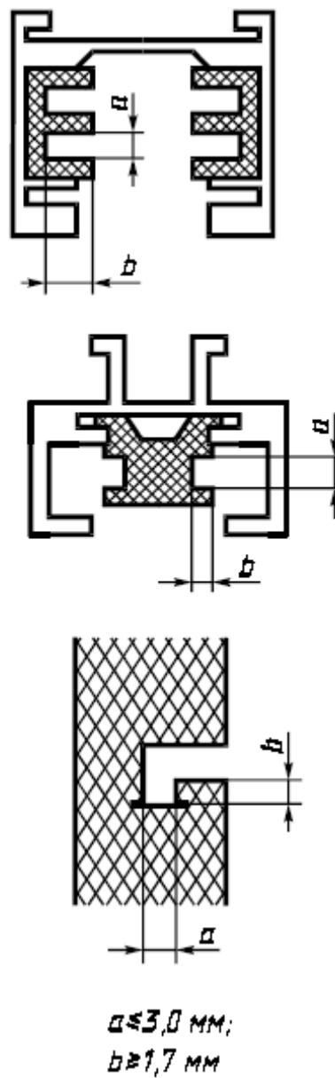
Рисунок 4 - Измеряемые места типичных секций шинпроводов класса I
