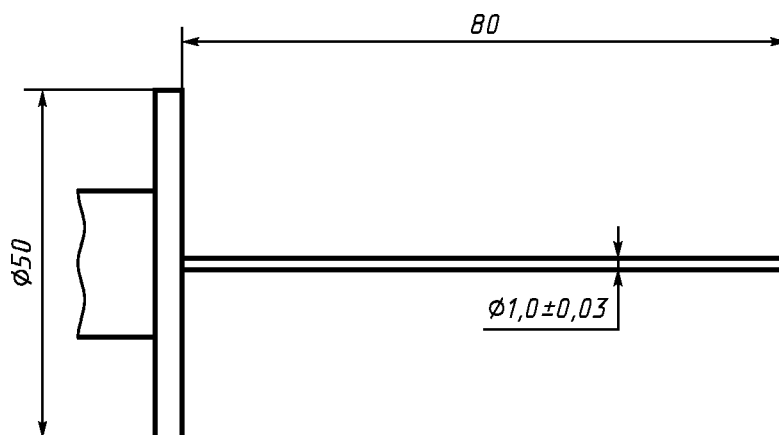
Рисунок 2 - Испытательный щуп
