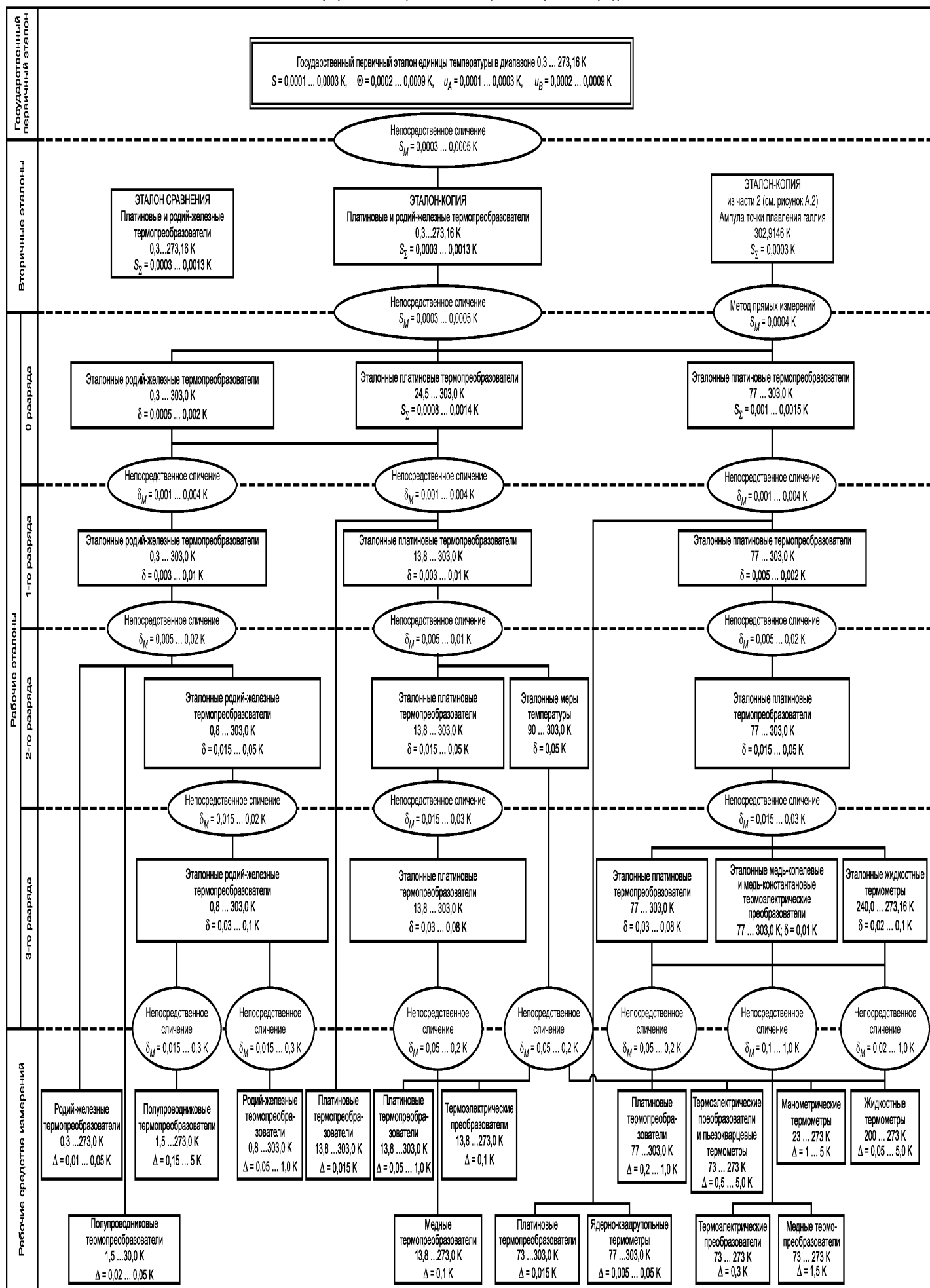
Рисунок А.1 – Поверочная схема для контактных термометров в диапазоне 0,3 К ... 273,16 К
