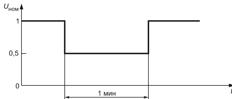
Рисунок В.3 — Провалы напряжения \Delta U = 50\%
