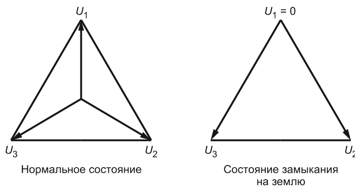
Рисунок С.2 — Напряжения на испытуемом счетчике
