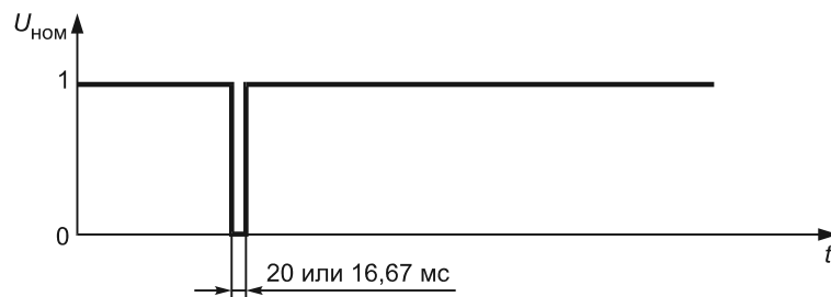
Рисунок В.2 —Прерывания напряжения \Delta U = 100\% , в течение одного цикла при номинальной частоте
