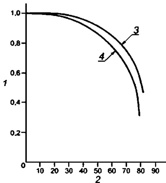
1 — Зависимость от угла падения, 2 — Угол падения (градусы); 3 — Единичный — K_{\text{остекленное покрытие}} , 4 — Двойной — остекленное покрытие
