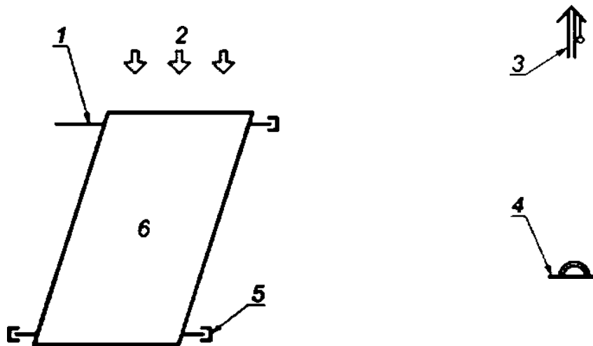
1 — Трубопровод, оставленный открытым. 2 — Солнечная радиация. 3 — Датчик температур окружающей среды. 4 — Пирометр на плоскости коллектора, 5 — Трубопровод, запечатанный с накладной гайкой, 6 — Коллектор
