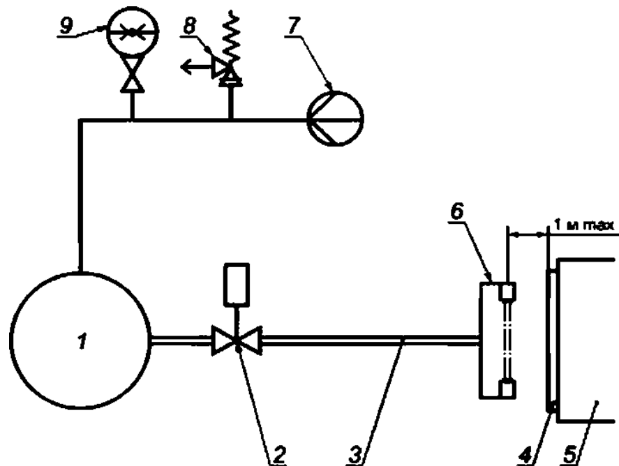
1 — Резервуар; 2 — Соленоидальный боковой клапан, быстрое открытие; 3 — Боченок; 4 — Коллектор; 5 — Жесткая рама; 6 — Фотоэлектрическая система измерения скорости; 7 — Источник пневматического давления; 8 — Предохранительный клапан; 9 — Манометр
