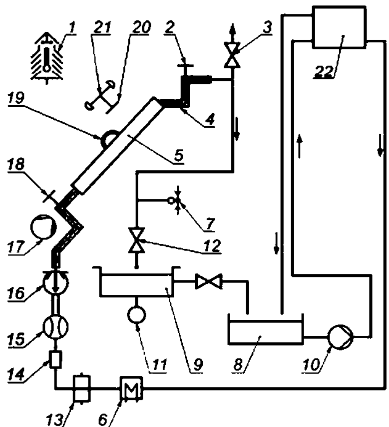
Рисунок 3 — Пример открытого (разомкнутого) испытательного контура
