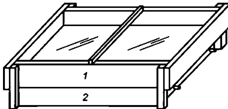
Рисунок А.12 — Описание схемы для испытательной механической нагрузки (положительное давление на поверхность коллектора)
