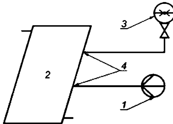
Г — Источник с-амалического давления; 2 — Коллектор; 3 — М*»метр; 4 — Отверстия • зазоре между покрытием коллектора и поглотителем
