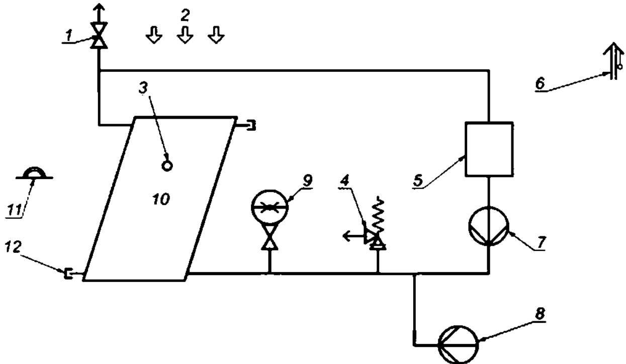
Рисунок А.3 — Описание схемы для испытания на прочность давление органических поглотителей для использования с жидкостями на основе масла (горячий источник масла)
