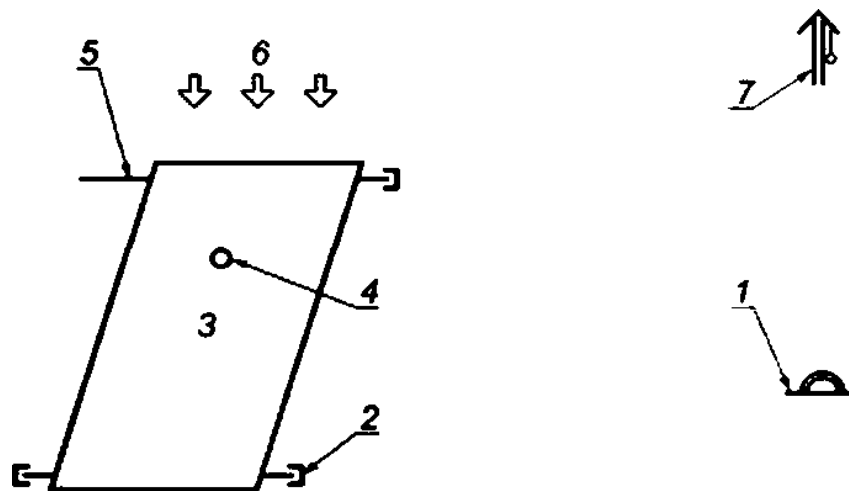
1 — Источник пневматического давления; 2 — Трубопровод, запечатанный с накидной гайкой; 3 — Коллектор; 4 — Температурный датчик, прикреплённый к поглотителю; 5 — Трубопровод, оставленный открытым; 6 — Пирометр на плоскости коллектора; 7 — Естественное или искусственное солнечное излучение; 8 — Датчик температуры окружающей среды
