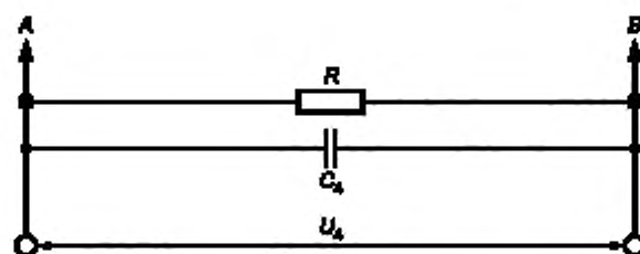
Рисунок G.4 — Схема измерения высокочастотных токов защитного проводника
