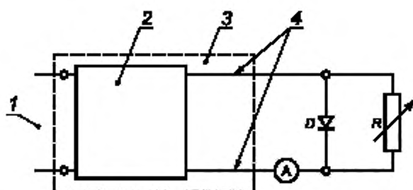
1 — сеть; 2 — ПРА, трансформатор, 3У; 3 — светильник; 4 — место присоединения лампы; D = 100 А, 600 В; R = 0...200 Ом (номинальная мощность резистора должна быть не менее 1/2 мощности лампы)
