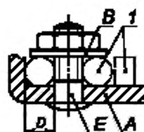
Контактные зажимы с крепежной гайкой
