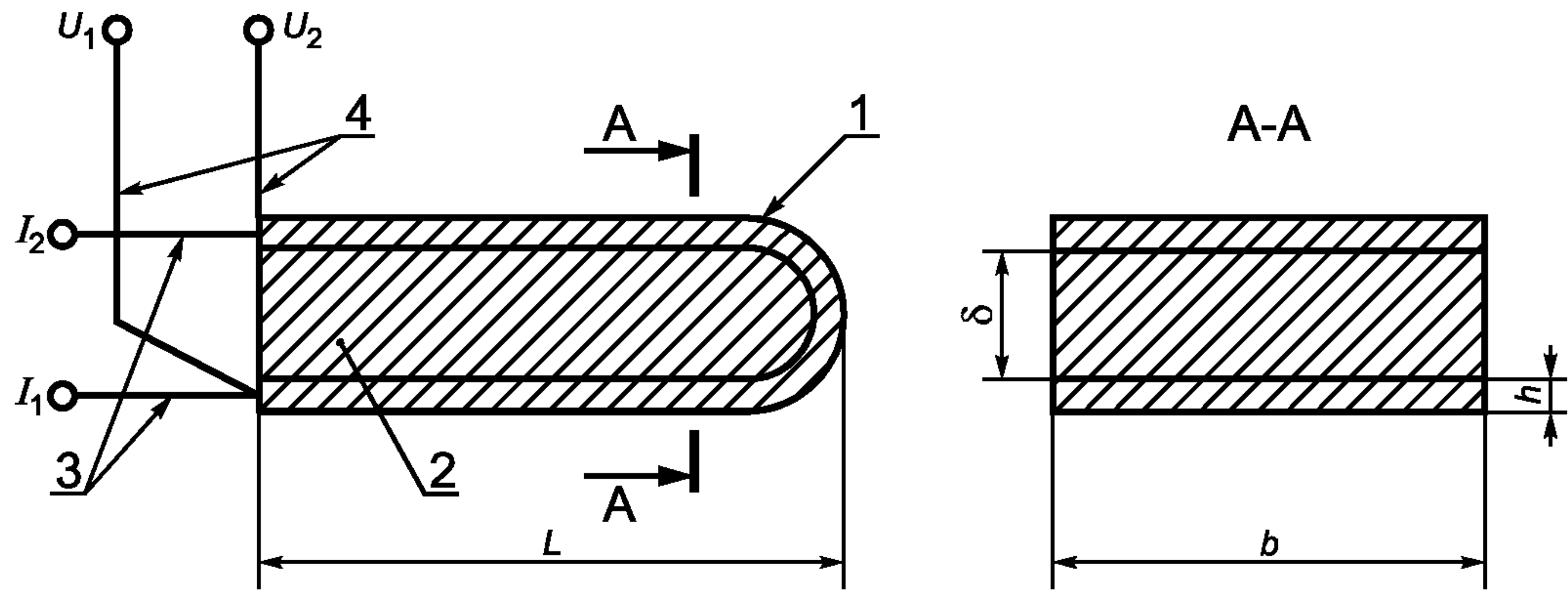
1 — резистивный элемент; 2 — изоляционная прокладка; 3 — токовые выводы; 4 — потенциальные выводы; I_1 и I_2 — токовые зажимы; U_1 и U_2 — потенциальные зажимы
