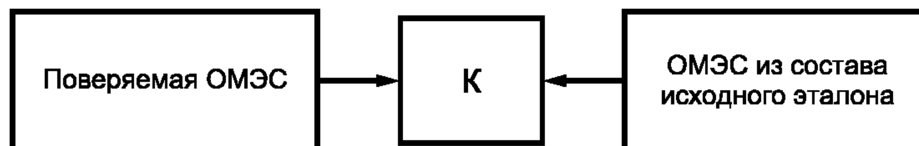
Рисунок Б.3 — Измерение с помощью компаратора сопротивлений
