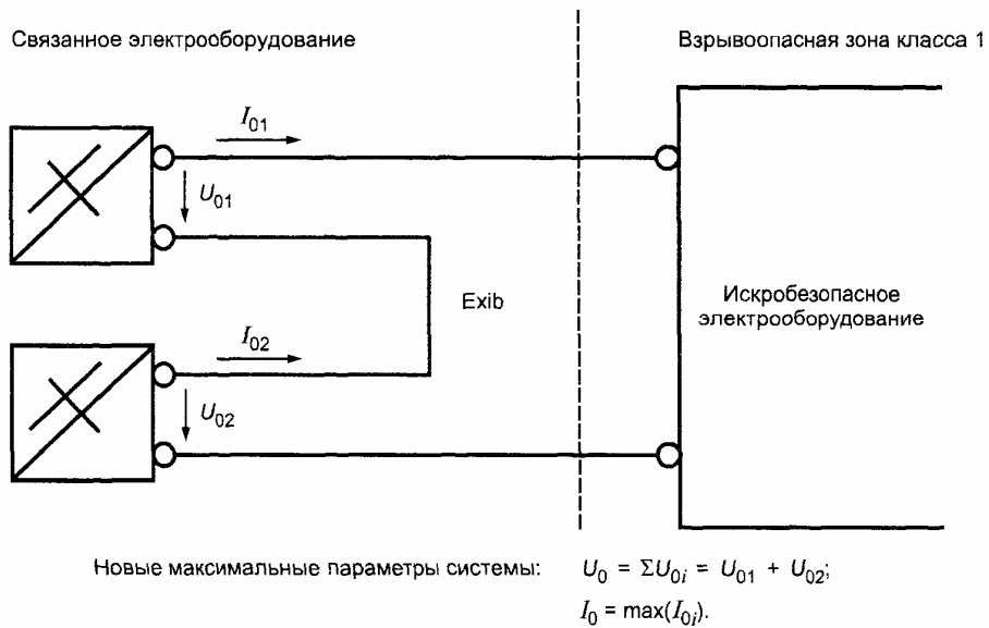
Рисунок В.1 — Последовательное соединение. Суммирование напряжений
