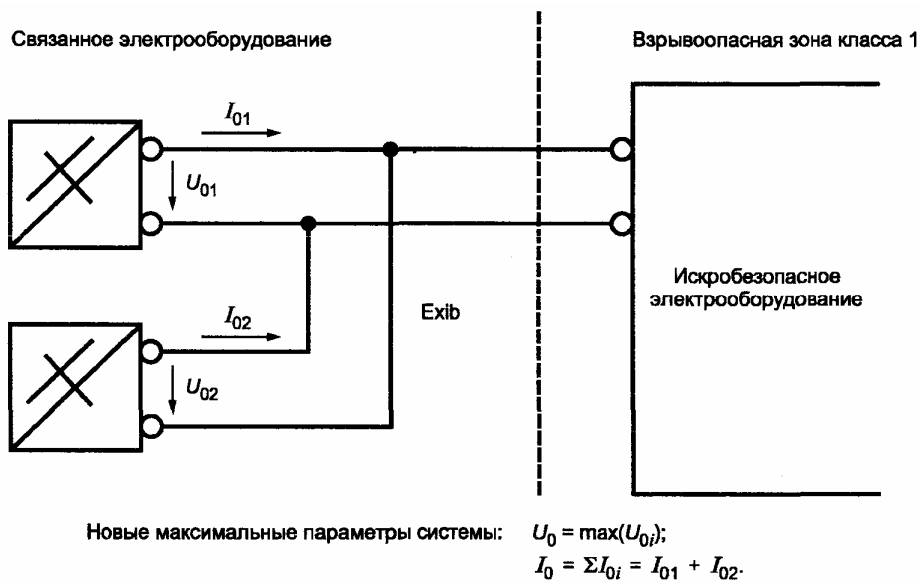
Рисунок В.2 — Параллельное соединение. Суммирование токов
