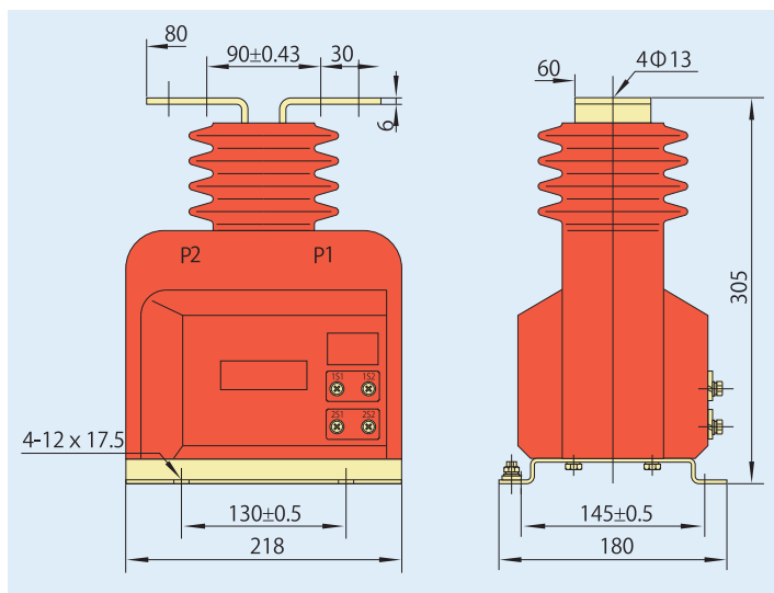
Рис. 6.1 Внешний вид и размеры трансформатора тока LQZBJ-10, LQJ8-10
