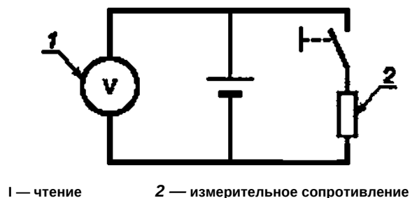
Рисунок 6 — Принципиальная схема
