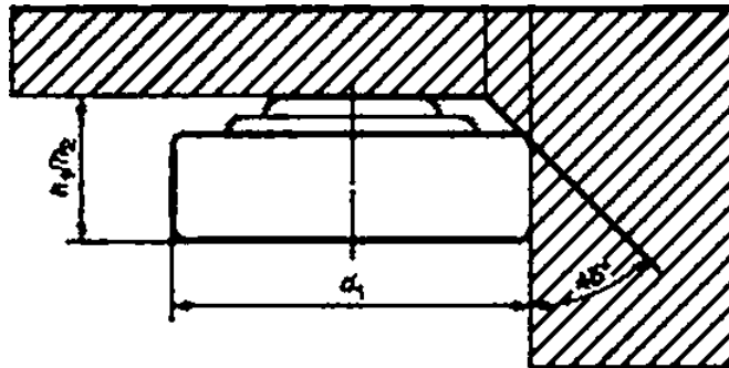
Рисунок 3 — Требования к форме
