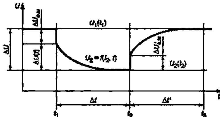
Рисунок 4 — Схематичное представление изменения напряжения при переходном процессе
