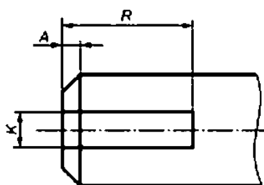
Рисунок Е.12 — Размеры штыревого наконечника
