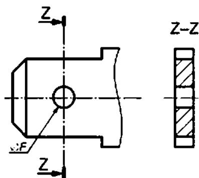
Рисунок Е.6 — Размеры прямоугольных элементов фиксации (см. рисунок Е.6)
