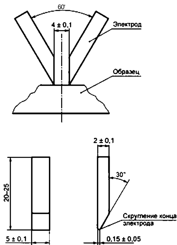
Рисунок 9 — Расположение и размеры электродов для испытания на треинтостойкость
