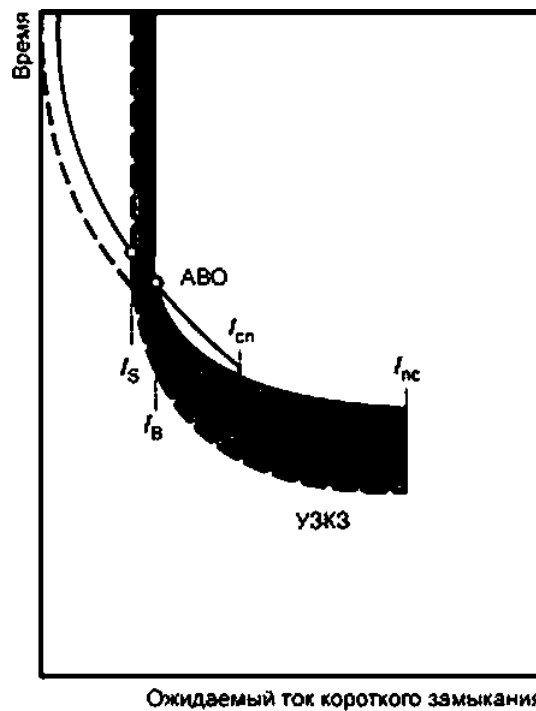
Рисунок F.4 — АВО с гидравлической электромагнитной защитой и резервная защита автоматическим выключателем с тепловой и электромагнитной защитой
