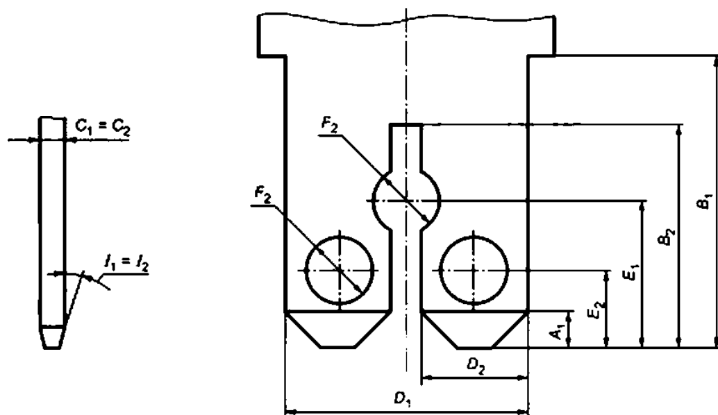
Рисунок Е.13 — Размеры штыревых наконечников для двух различных гнездовых соединителей (см. 6.1.7.1)
