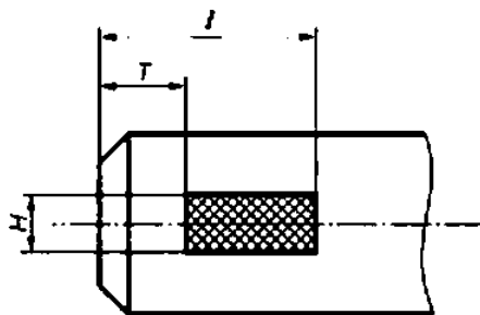
Рисунок Е.10 — Размеры штыревого наконечника
