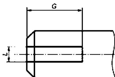
Рисунок Е.11 — Размеры штыревого наконечника
