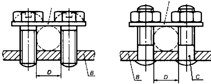
A — планка; в — неподвижная часть; C — винт. O — окно для проводника
