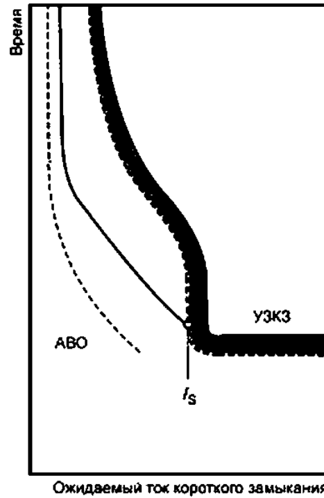
Рисунок F.4 — АВО с гидравлической электромагнитной защитой и резервная защита автоматическим выключателем с тепловой и электромагнитной защитой
