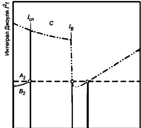
Рисунок F.8b — Ненадлежащая координация
