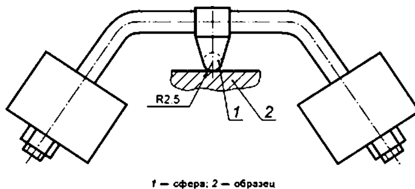
Рисунок 8 — Установка для испытаний давлением шарика
