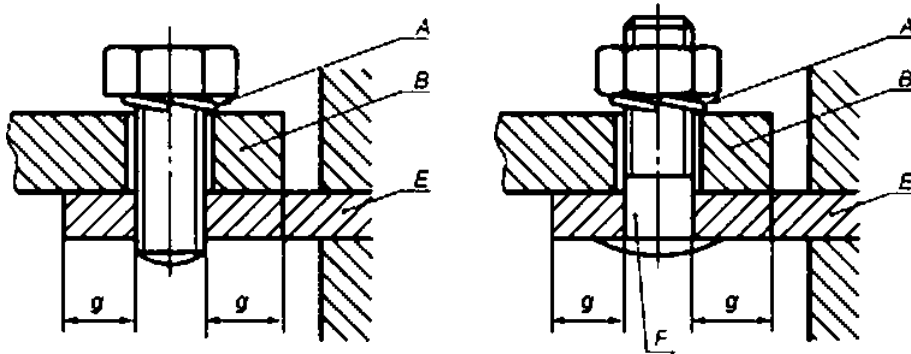
A — устройство против самоотвинчивания. в — кабельный наконечник или шина; E — неподвижная часть; F — винт, \delta — расстояние перекрытия
