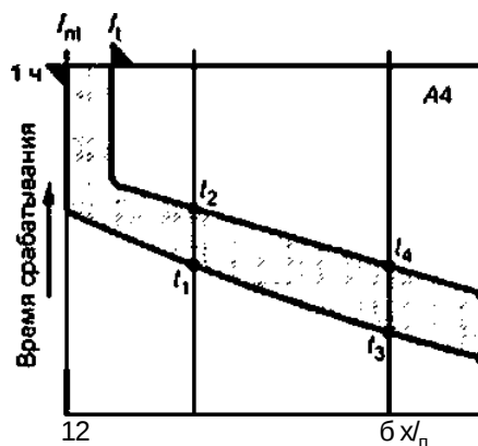
Рисунок А.4 — Характеристика гибридно-электромагнитной защиты
